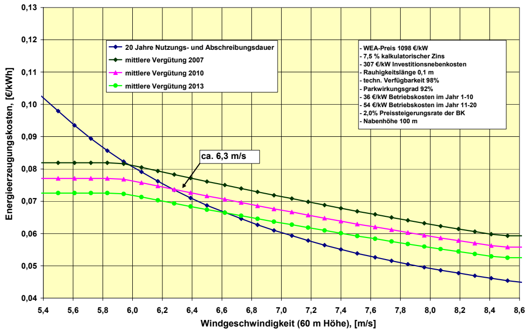
Abb. 10-1: Orientierungswerte für Stromgestehungskosten und mittlere Vergütung über der Standortqualität für Windenergieanlagen der Leistungsklassen von 1,3 bis 1,9 MW bei einer Nabhöhe von 100 m nach ZSW et al. 2007 [1]
