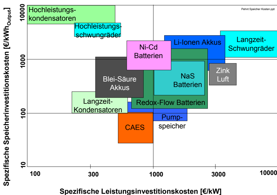
Abb. 12-2: Einordnung der Betriebs- und Investitionskosten verschiedener Speichertechnologien (heutiger Stand und kurzfristiges Senkungspotenzial) [41, 45]
