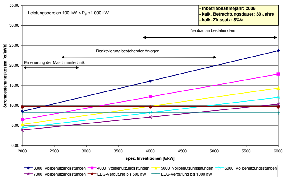
Abb. 6-1: Orientierungswerte der Stromgestehungskosten von Wasserkraftanlagen im Leistungsbereich von 100 bis 1000 kW nach ZSW et al. 2007 [1]
