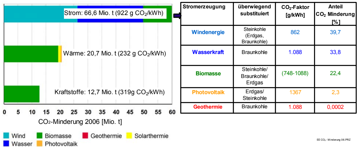
Abb. 4-1: CO 2 -Vermeidung durch die Nutzung Erneuerbare Energien im Jahr 2006 nach [1]
