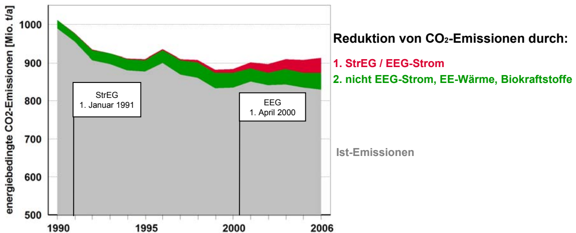
Abb. 4-2: Entwicklung der energiebedingten CO 2 -Emissionen in Deutschland im Zeitraum 1990 bis 2006 [2]
