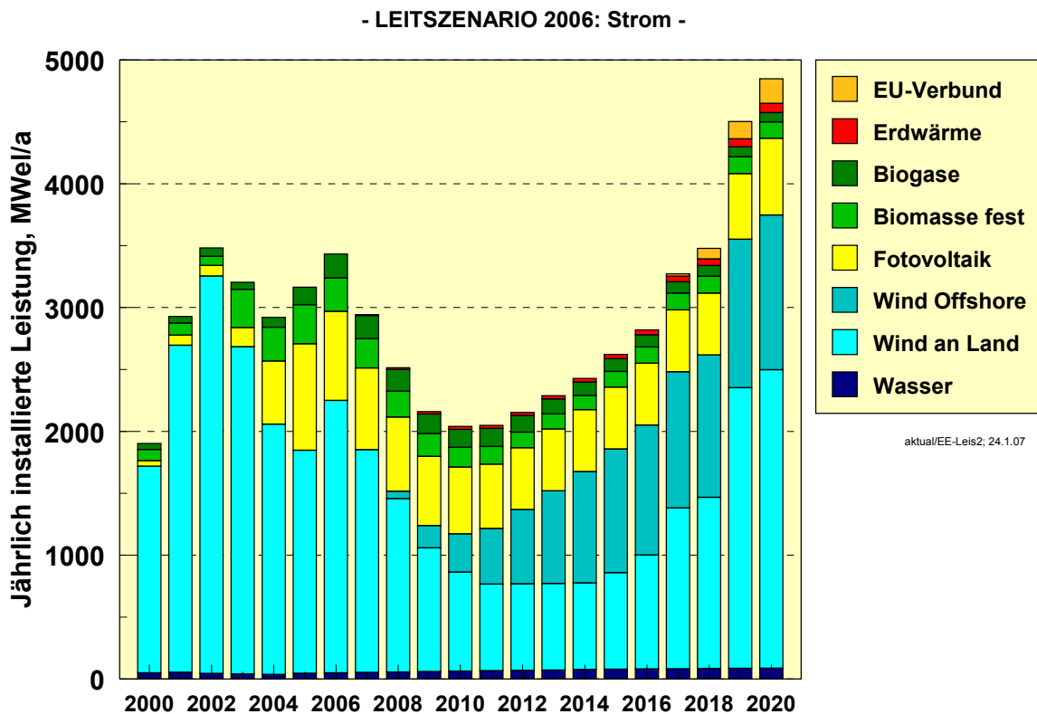
Abb. 14-1: Entwicklung der jährlich zugebauten installierten Leistung von Anlagen zur Erzeugung von Strom aus Erneuerbaren Energien von 2000 bis 2020 gemäß Leitstudie [5]
