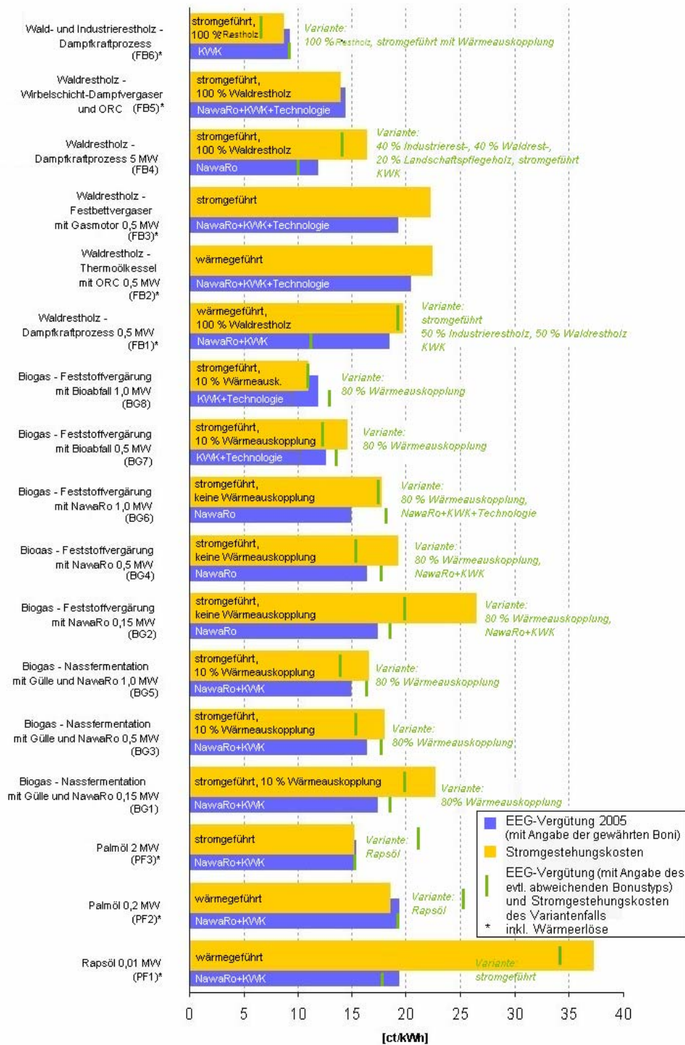
Abb. 8-2: Vergleich der Stromgestehungskosten von Anlagen zur Biomassennutzung mit der EEG-Einspeisevergütung nach IE/Prognos 2006 [14]
