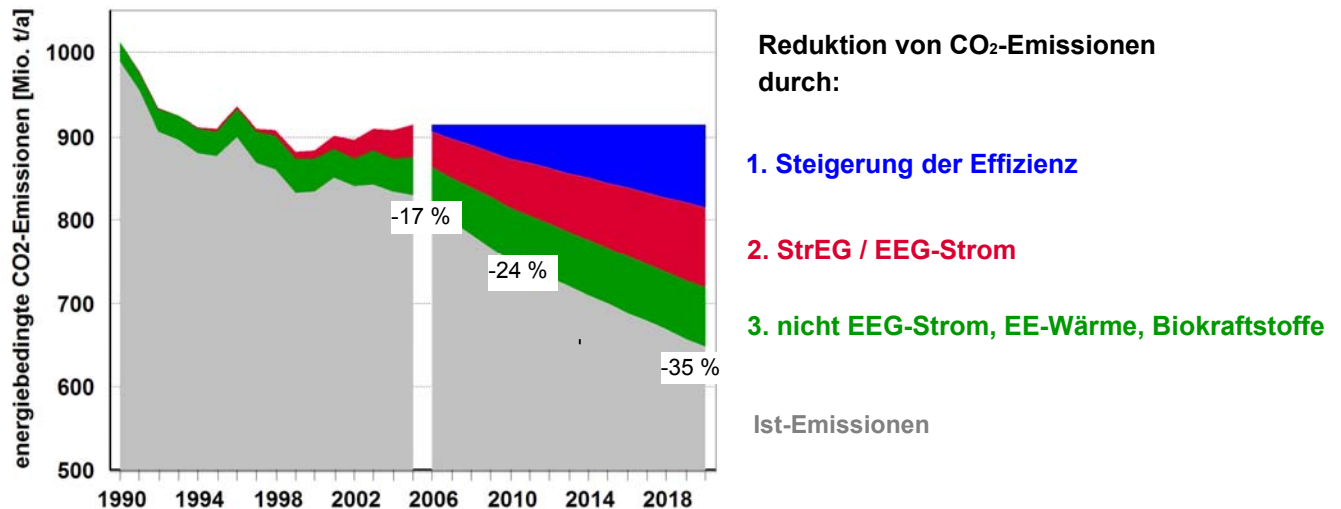
Abb. 14-6: Entwicklung der energiebedingten CO 2 -Emissionen in Deutschland im Zeitraum 1990 bis 2020 auf Basis der Annahmen in [5]
