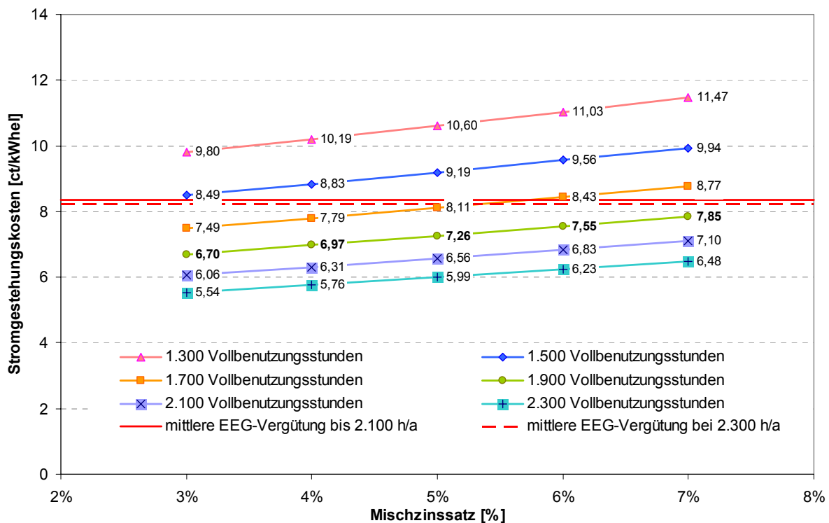
Abb. 10-5: Stromgestehungskosten bei einer Repowering-Windenergieanlage von 1,5 MW in Abhängigkeit vom Zinssatz und den Vollbenutzungsstunden in ct/kWh nach IE/Pognos 2006 [14]
