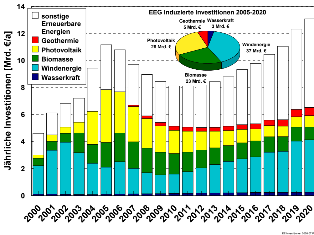
Abb. 14-7: Investitionen in Anlagen zur Stromerzeugung aus Erneuerbaren Energien nach [5]
