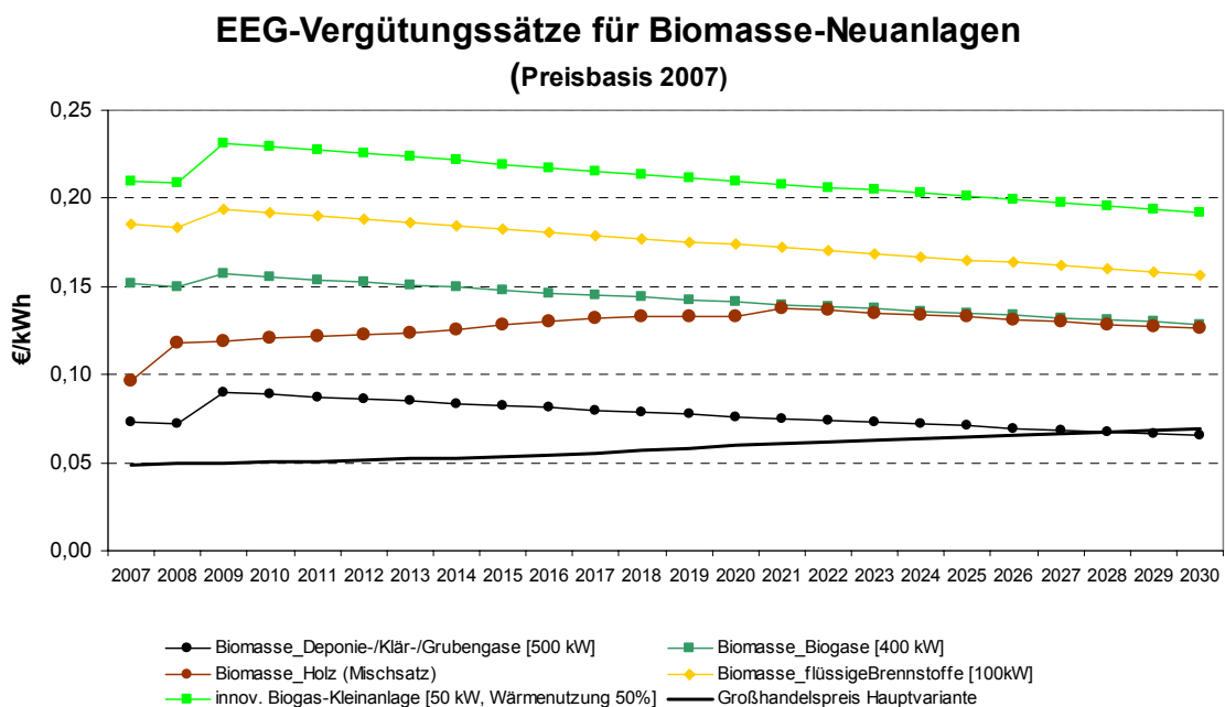
Abb. 14-4: Entwicklung der EEG-Vergütungssätze für ausgewählte Anwendungen im Bereich der Biomasse nach Inbetriebnahmejahr auf Basis der Maßnahmen-Empfehlungen im Erfahrungsbericht (Preisbasis 2007).
