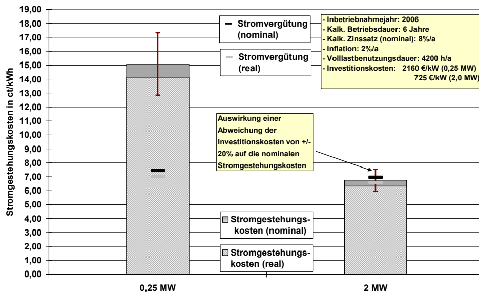
Abb. 7-2: Orientierungswerte für reale und nominale Stromgestehungskosten für Neuanlagen (Inbetriebnahmejahr 2006) gegenüber der mittleren Vergütung (real und nominal) von Deponiegasanlagen (Variante) nach ZSW et al. 2007 5 [1]
