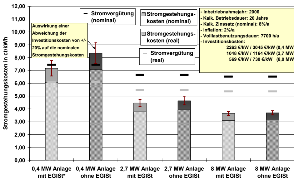
Abb. 7-4: Orientierungswerte für reale und nominale Stromgestehungskosten für Neuanlagen (Inbetriebnahmejahr 2006) gegenüber der mittleren Vergütung (real und nominal) von Grubengasanlagen (Basisfall) nach ZSW et al. 2007 6 [1]
