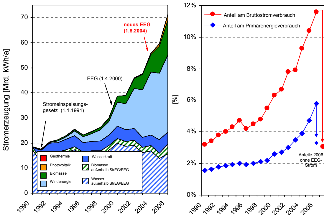
Abb. 3-3: Entwicklung der Stromerzeugung aus Erneuerbaren Energien und Anteile am Bruttostromverbrauch und am Primärenergieverbrauch (berechnet nach Wirkungsgradmethode) im Zeitraum 1990 bis 2006 [1]
