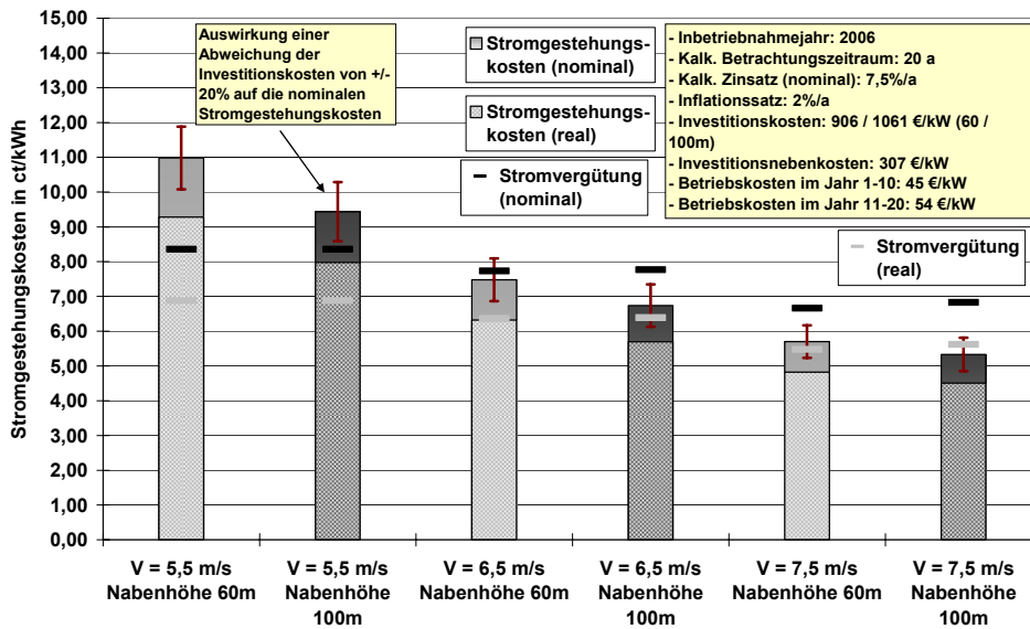
Abb. 10-3: Orientierungswerte für reale und nominale Stromgestehungskosten für Neuanlagen (Inbetriebnahmejahr 2006) gegenüber der mittleren Vergütung (real und nominal) von Windenergieanlagen der Leistungsklassen von 2,0 bis 3,0 MW nach ZSW et al. 2007 15 [1]
