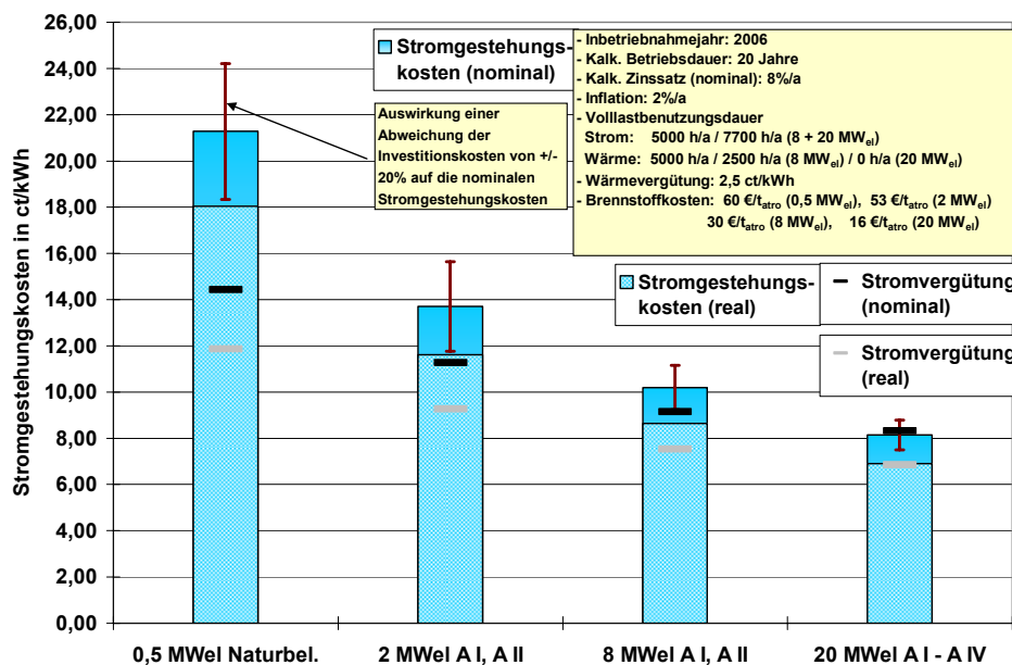
Abb. 8-1: Orientierungswerte für reale und nominale Stromgestehungskosten für Neuanlagen (Inbetriebnahmejahr 2006) gegenüber der mittleren Vergütung (real und nominal) von Biomasse(heiz)kraftwerken im Basisfall nach ZSW et al. 2007 9 [1]
