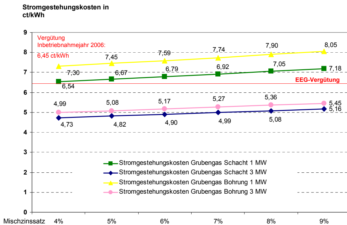
Abb. 7-7: Stromgestehungskosten bei Grubengas in Abhängigkeit vom Zinssatz Bewertung der Ergebnisse in ct/kWh nach IE/Prognos 2006 [14]
