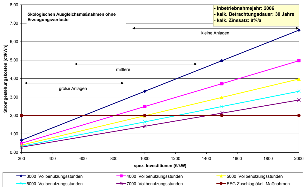
Abb. 6-4: Orientierungswerte für zusätzlich durch die Umsetzung von ökologischen Anpassungsmaßnahmen entstehende Stromgestehungskosten im Verhältnis zum gewährten EEG-Bonus nach ZSW et al. 2007 [1]
