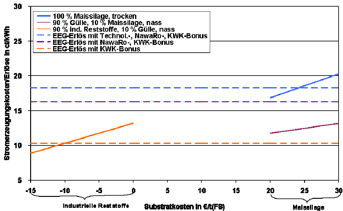
Abb. 8-5: Orientierungswerte für nominale Stromgestehungskosten für Neuanlagen (Inbetriebnahmejahr 2006) gegenüber der mittleren Vergütung (nominal) von 0,5 MW el -Biogasanlagen beim Einsatz diverser Substrate in Abhängigkeit von den Substratkosten (Für die Verwendung von Gülle wurden keine Beschaffungs- und Transportkosten angesetzt; die weiteren Parameter sind mit denen in Abb. 8-3 identisch) [23]
