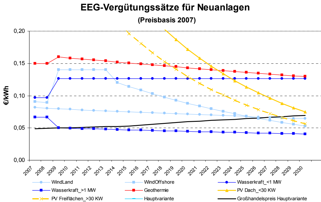
Abb. 14-3: Entwicklung der EEG-Vergütungssätze für ausgewählte Anwendungen (ohne Biomasse) nach Inbetriebnahmejahr auf Basis der Maßnahmen-Empfehlungen im Erfahrungsbericht (Preisbasis 2007). 20
