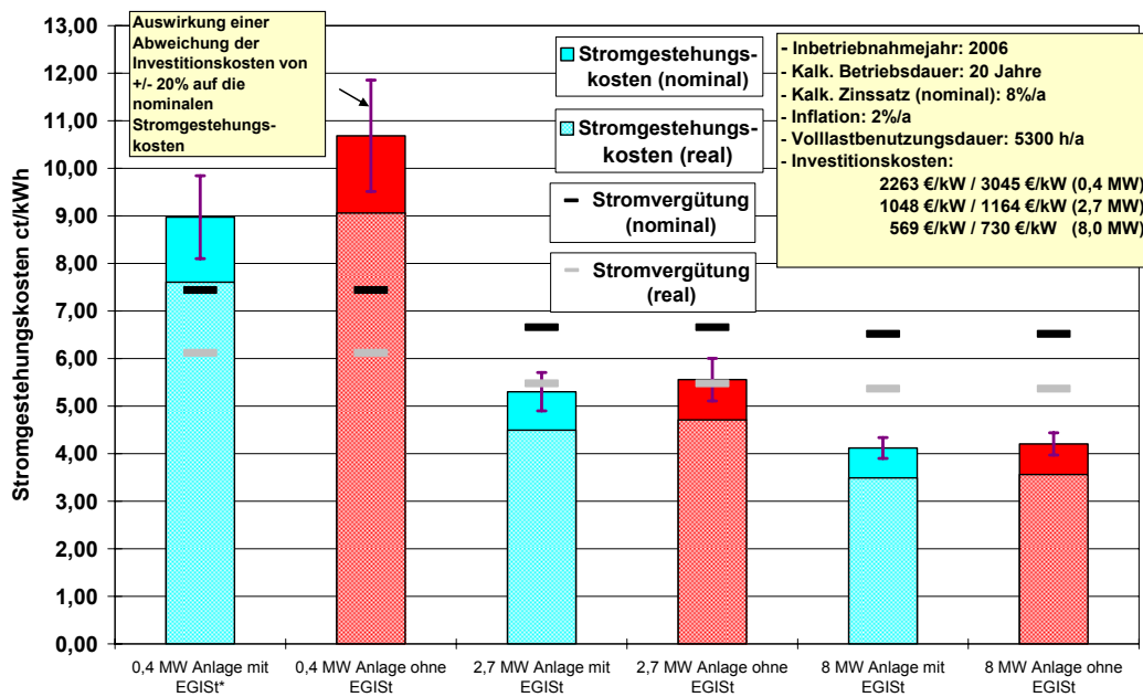
Abb. 7-6: Orientierungswerte für reale und nominale Stromgestehungskosten für Neuanlagen (Inbetriebnahmejahr 2006) für Anlagen mit einer Vollastbenutzungsdauer von 5.300 h/a gegenüber der mittleren Vergütung (real und nominal) von Grubengasanlagen (Variante 2) nach ZSW et al. 2007 8 [1]
