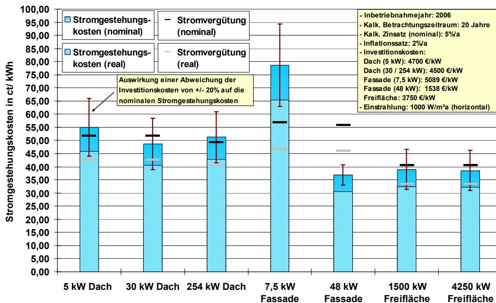
Abb. 11-1: Orientierungswerte für Stromgestehungskosten typischer Photovoltaikanlagen 17 [1]
