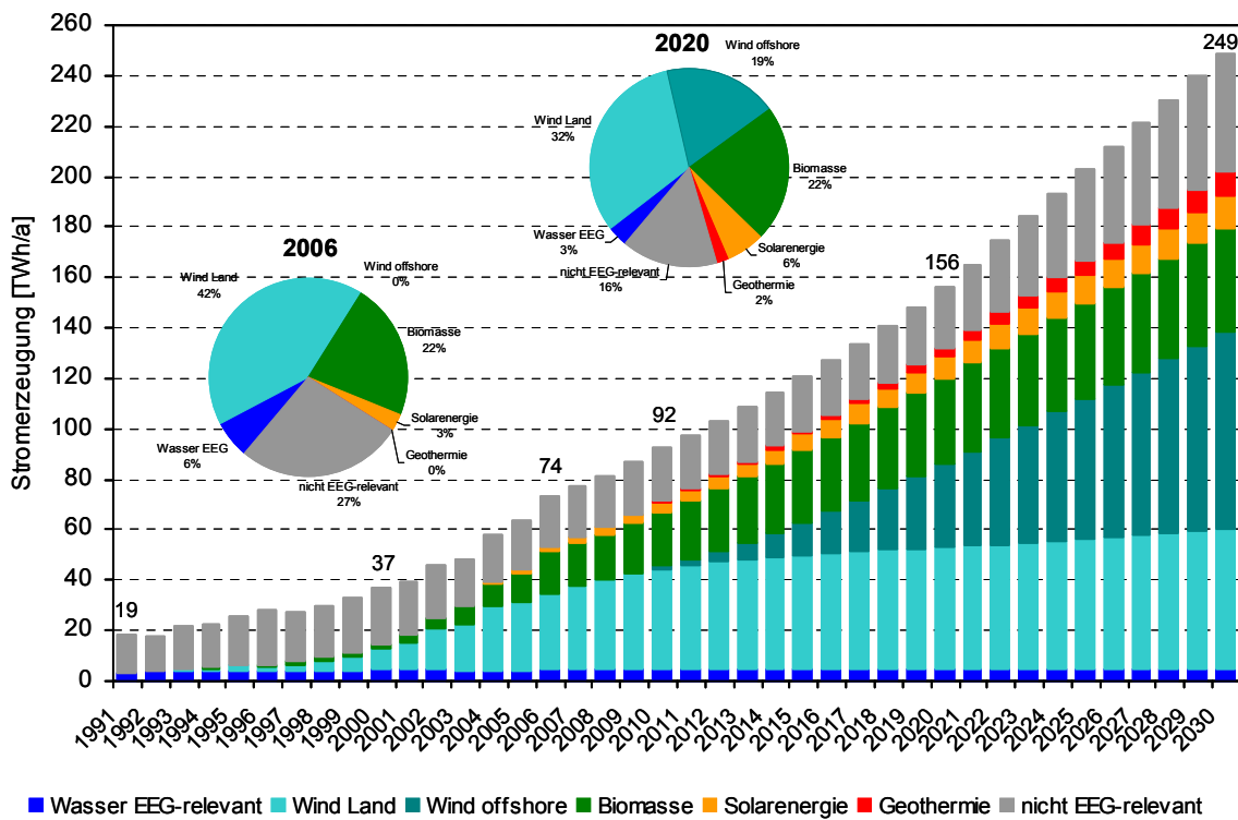
Abb. 14-2: Entwicklung der Stromerzeugung aus Erneuerbaren Energien von 1991 bis 2030 gemäß Leitstudie [5]
