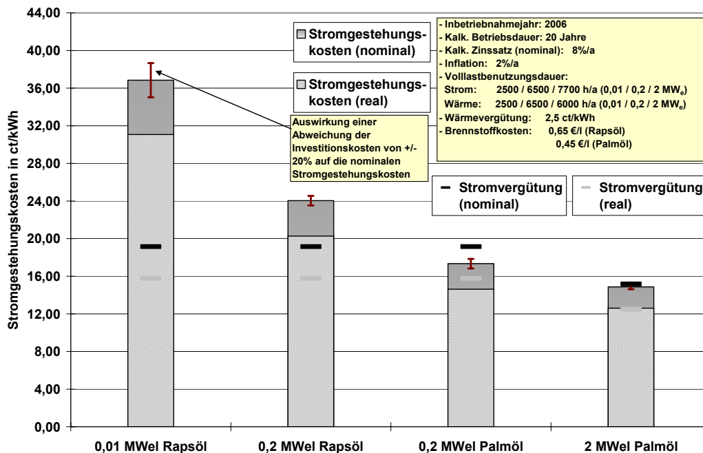
Abb. 8-6: Orientierungswerte für reale und nominale Stromgestehungskosten für Neuanlagen (Inbetriebnahmejahr 2006) gegenüber der mittleren Vergütung (real und nominal) von Pflanzenöl-BHKW-Anlagen nach ZSW et al. 2007 12 [1]
