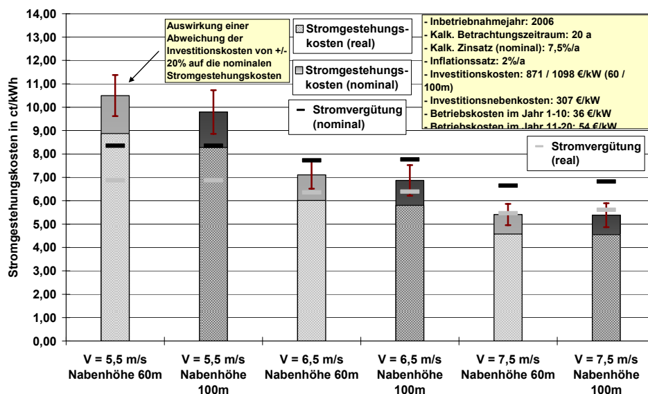
Abb. 10-2: Orientierungswerte für reale und nominale Stromgestehungskosten für Neuanlagen (Inbetriebnahmejahr 2006) gegenüber der mittleren Vergütung (real und nominal) von Windenergieanlagen der Leistungsklassen von 1,3 bis 1,9 MW nach ZSW et al. 2007 14 [1]
