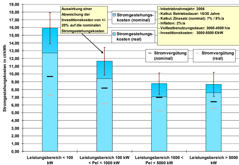
Abb. 6-2: Orientierungswerte für reale und nominale Stromgestehungskosten für Neuanlagen (Inbetriebnahmejahr 2006) gegenüber der mittleren Vergütung (real und nominal) von Wasserkraftanlagen nach ZSW et al. 2007 3 [1]
