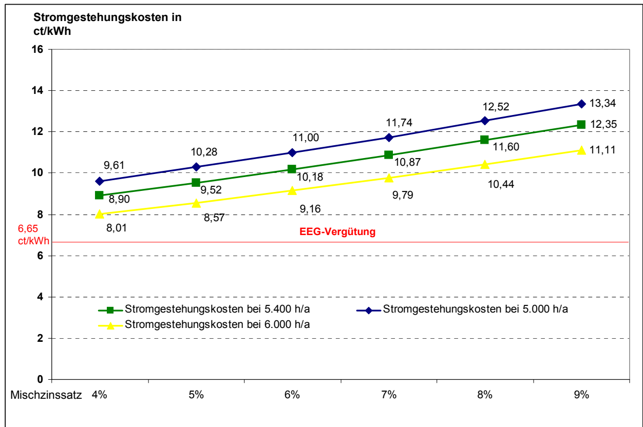
Abb. 6-3: Stromgestehungskosten bei Wasserkraftwerken von 2,5 MW in Abhängigkeit vom Zinssatz in ct/kWh nach IE/Prognos 2006 [14]
