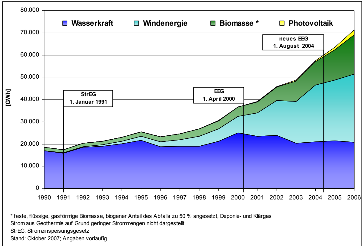
Abb. 3-4: Beitrag der Erneuerbaren Energien zur Stromerzeugung 1990 bis 2006 [2, 4]
