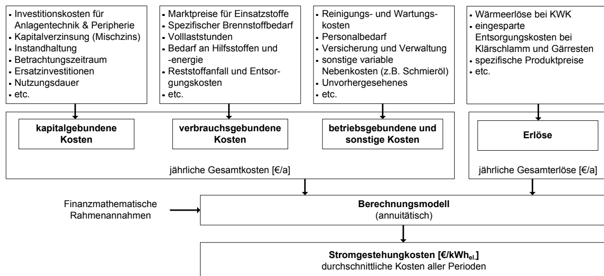
Abb. 15-2: Methodik und Eingangsgrößen für die Berechnung der Stromgestehungskosten
