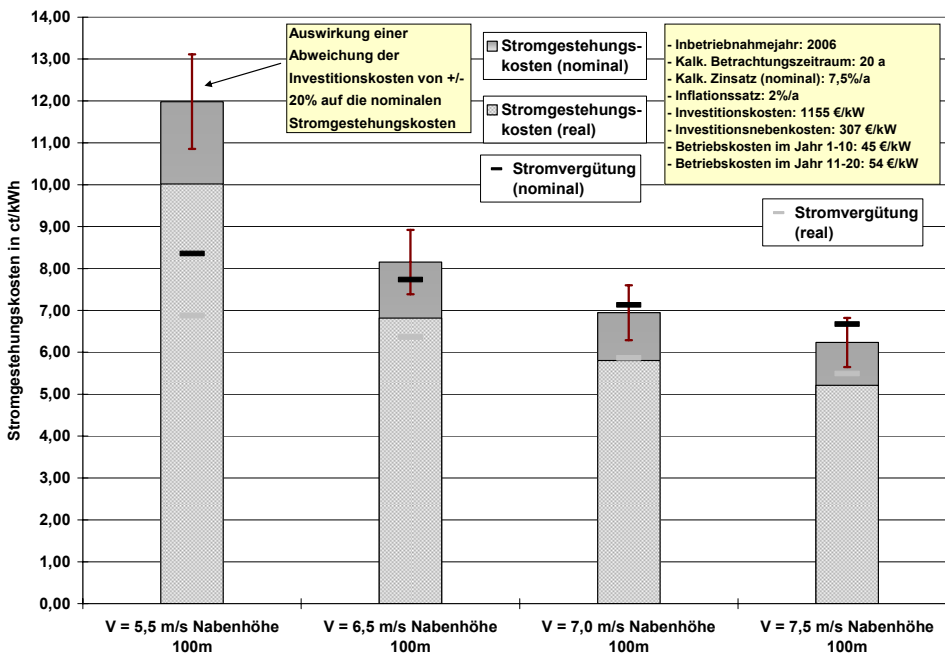
Abb. 10-4: Orientierungswerte für reale und nominale Stromgestehungskosten für Neuanlagen (Inbetriebnahmejahr 2006) gegenüber der mittleren Vergütung (real und nominal) von Windenergieanlagen der Leistungsklasse über 3,0 MW nach ZSW et al. 2007 16 [1]
