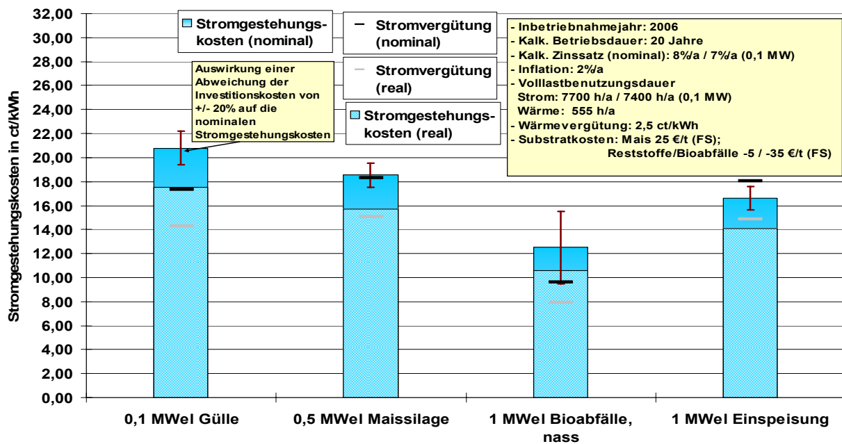
Abb. 8-3: Orientierungswerte für reale und nominale Stromgestehungskosten für Neuanlagen (Inbetriebnahmejahr 2006) gegenüber der mittleren Vergütung (real und nominal; bei Einsatz von Maissilage inklusive Technologiebonus) von Biogasanlagen im Basisfall nach ZSW et al. 2007 10 [1]
