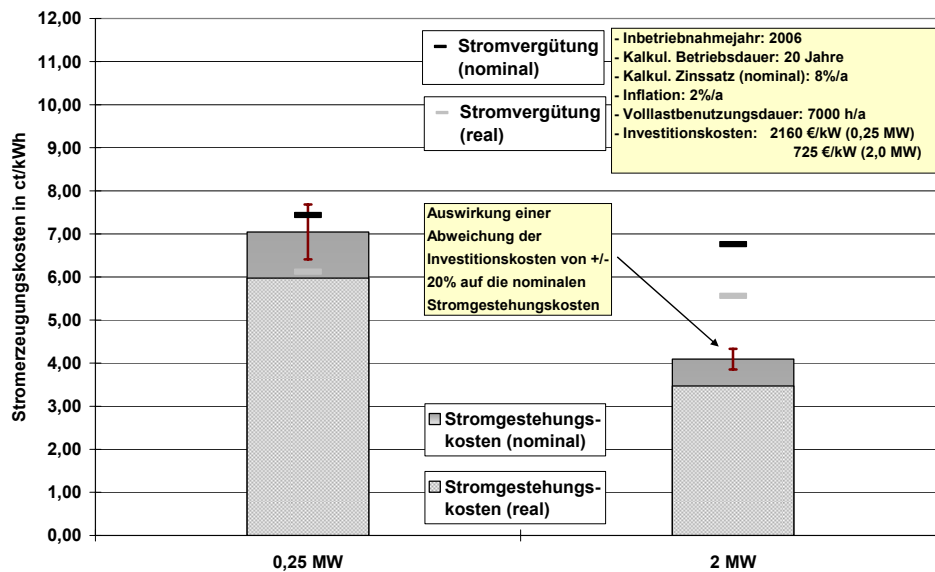
Abb. 7-1: Orientierungswerte für reale und nominale Stromgestehungskosten für Neuanlagen (Inbetriebnahmejahr 2006) gegenüber der mittleren Vergütung (real und nominal) von Deponiegasanlagen (Basisfall) nach ZSW et al. 2007 4 [1]
