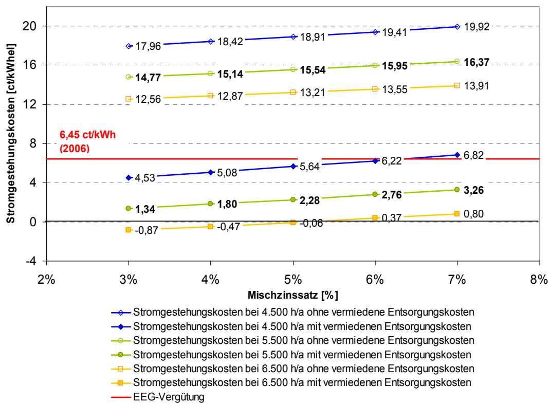
Abb. 7-3: Stromgestehungskosten bei Klärgas von 0,5 MW e in Abhängigkeit vom Zinssatz in ct/kWh nach IE/Prognos 2006 [14]
