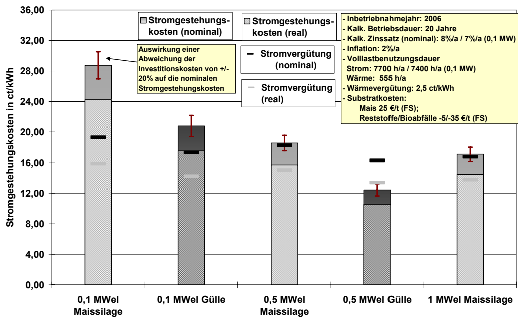
Abb. 8-4: Orientierungswerte für reale und nominale Stromgestehungskosten für Neuanlagen (Inbetriebnahmejahr 2006) gegenüber der mittleren Vergütung (real und nominal; bei 100 % Maissilage inklusive Technologiebonus) von Biogasanlagen beim Einsatz von 100 % Maissilage bzw. 90 % Gülle, 10 % Maissilage (Wirkung des NawaRo-Bonus) nach ZSW et al. 2007 11 [1]
