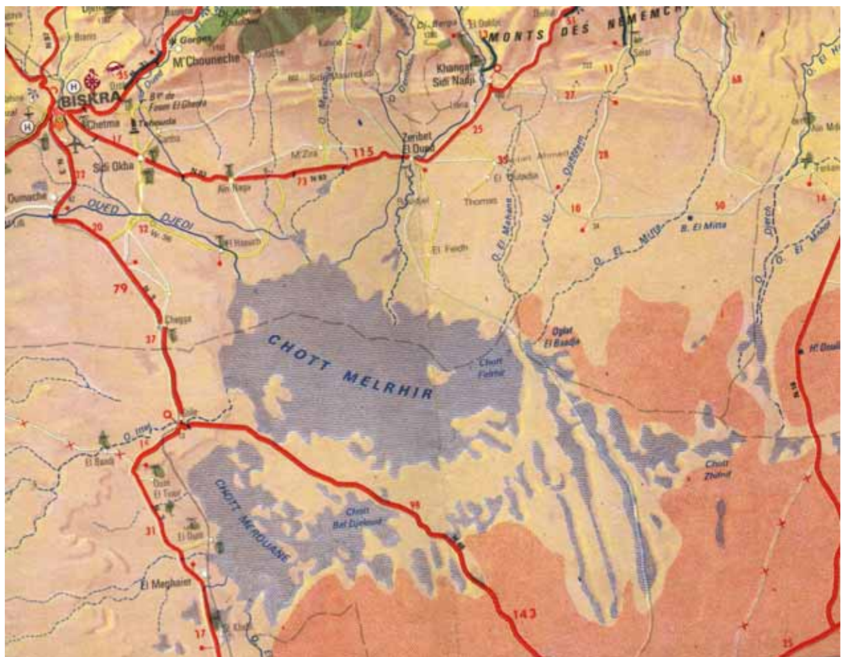
Fig. 1- Situation géographique du chott Melghir.
