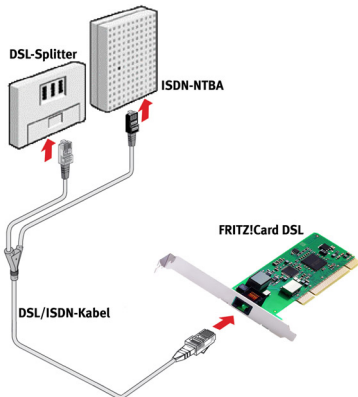
Anschluss von FRITZ!Card DSL an DSL und ISDN
