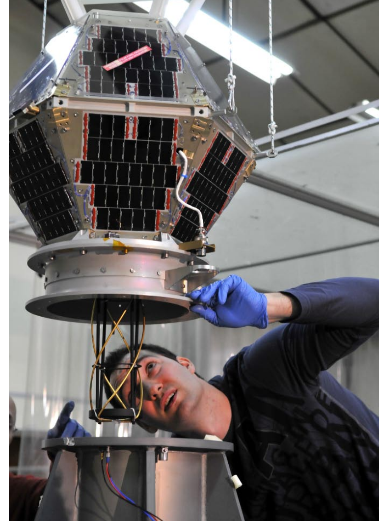
Preparación para las pruebas estructurales Getting ready for the structural tests
