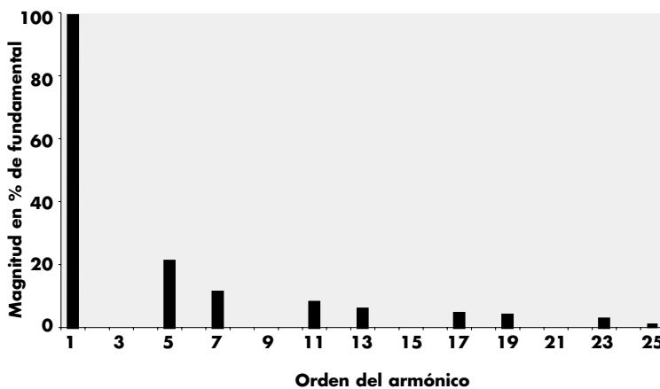
Figura 6 - Espectro armónico de un puente de seis pulsos
