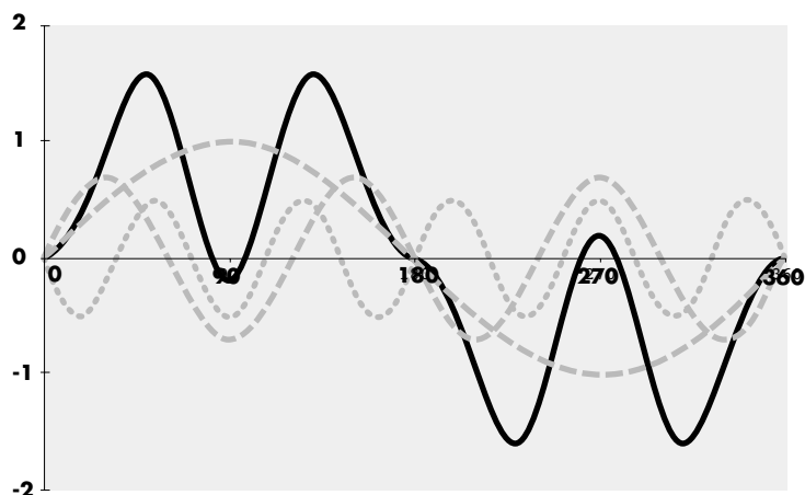
Figura 2 - Forma de onda de corriente distorsionada
