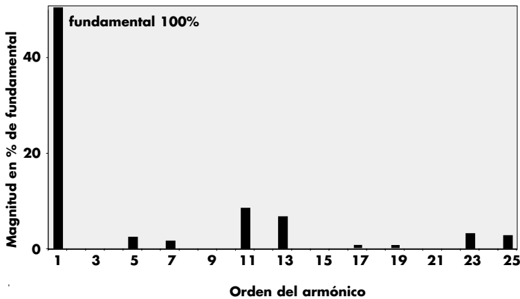
Figura 8 - Espectro armónico típico de un puente de doce pulsos
