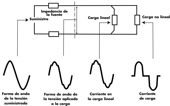
Figura 15 - Distorsión de la onda de tensión causada por una carga no lineal
