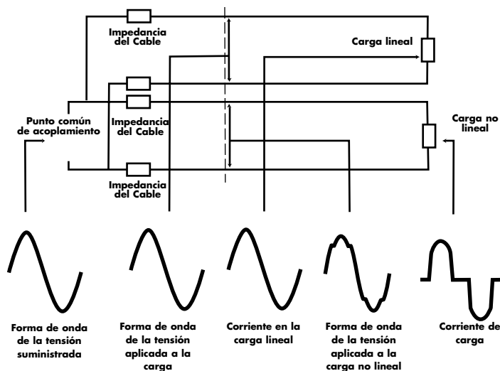
Figura 16 - Separación de las cargas lineales de las no lineales
