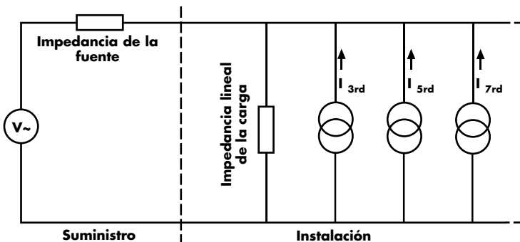
Figura 11 - Circuito equivalente de una carga no lineal
