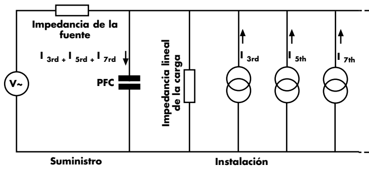
Figura 14 - Circuito equivalente de una carga no lineal con un condensador para la corrección del factor de potencia
