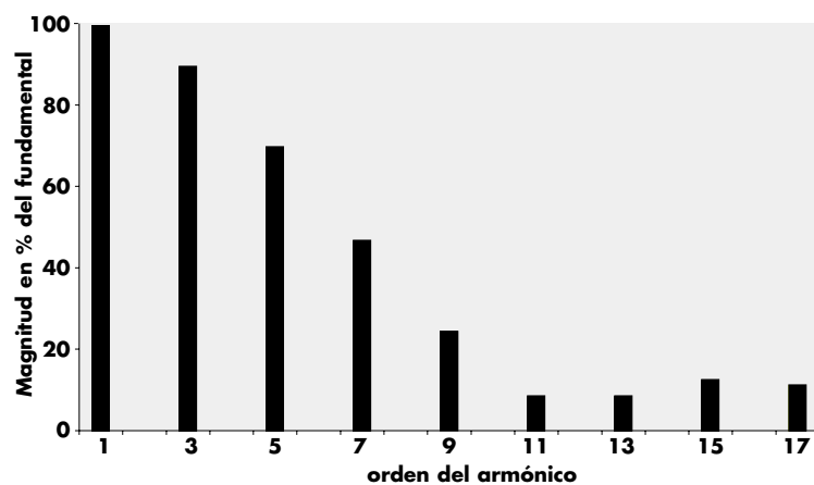
Figura 6 - Espectro armónico de un PC típico
