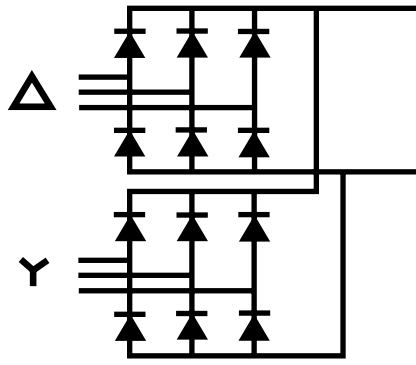
Figura 7 - Puente de doce pulsos
