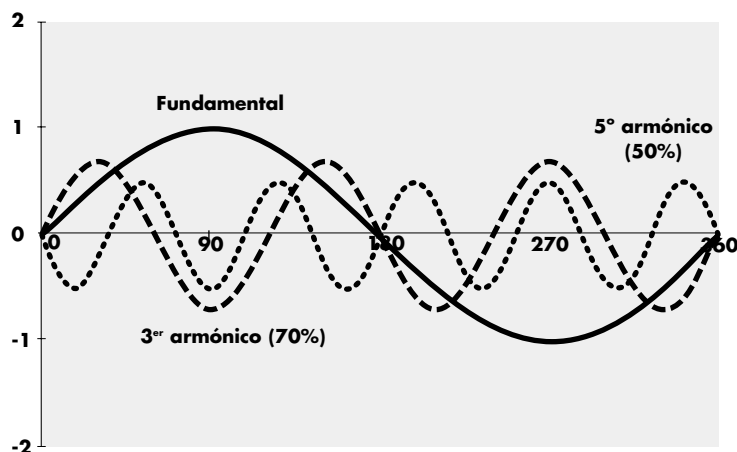
Figura 1 - Onda fundamental con 3º y 5º armónicos
