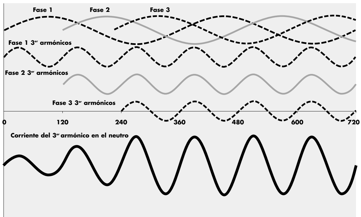
Figura 12 - Suma de las tres corrientes triple-N en el neutro
