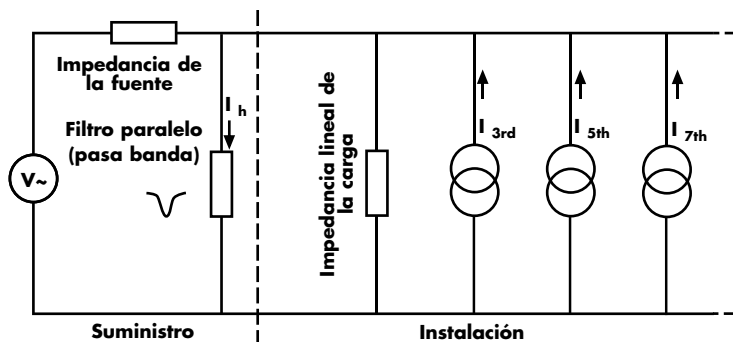
Figura 17 - Filtro pasivo de armónicos en paralelo con la carga
