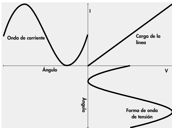
Figura 9 - Forma de onda en una carga lineal
