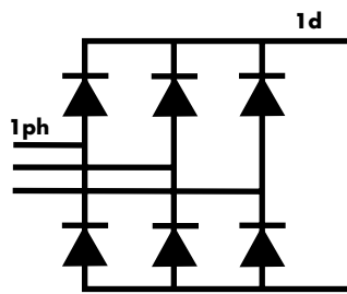
Figura 5 - Puente trifásico o de seis pulsos
