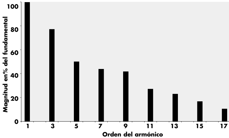
Figura 4 - Espectro armónico de una lámpara CFL
