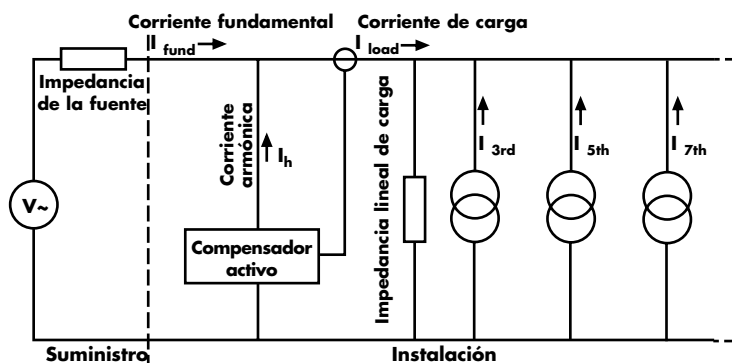
Figura 20 - Compensador activo de armónicos
