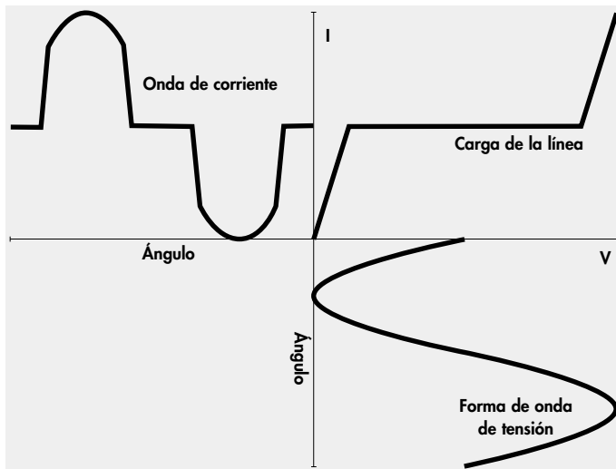
Figura 10 - Forma de onda de una carga no lineal
