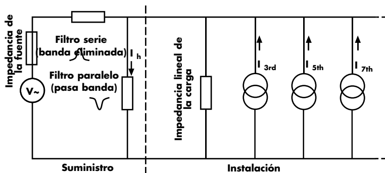
Figura 18 - Filtro pasivo de armónicos en serie y paralelo con la carga
