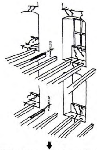
Sprickbildningens system: fönsterbröstningarna och den skevande karmen tar som svagaste element mellan murpelarna upp spänningarna i grunden. Sprickorna uppträder helt naturligt i detta område.
