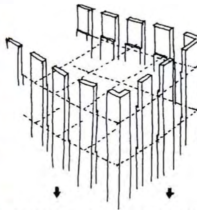
En flervåningsbyggnad av äldre modell skildrad som en serie murpelare sammanhållna av bjälklagens sega dragankarjärnsystem. Eventuella sättningar kan och får förekomma individuellt pelarna emellan.
