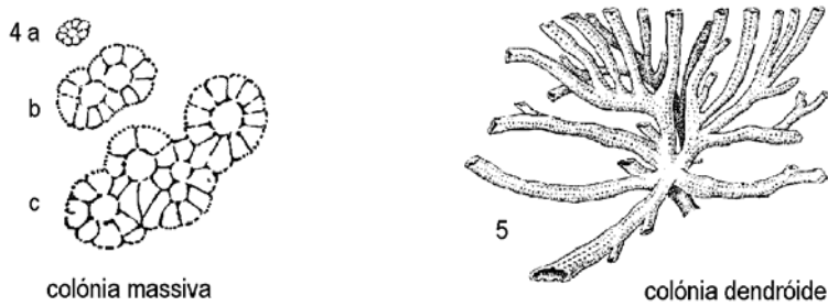
Fig. 2.2 Aspecto exterior de algumas formas típicas de arqueociatos solitários e coloniais. 1 - Dokidocyathus ; 2 - Okulitchicyathus ; 3 - Kotuyicyathus ; 4a-c - Ajacicyathus , cortes transversais sucessivos; 5 - Archaeolythus . Adaptado de diversos autores in HILL (1972).
