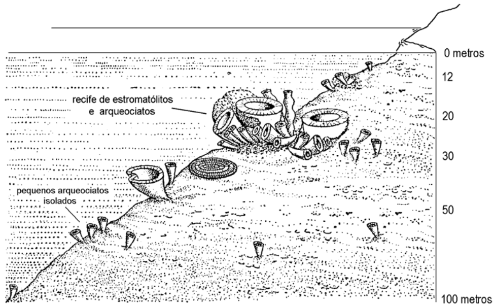
Fig. 2.3 Distribuição batimétrica dos arqueociatos e sua relação com a formação de recifes de estromatólitos e arqueociatos. Adaptado de ZHURAVLEVA (1960, in HILL, 1972).
