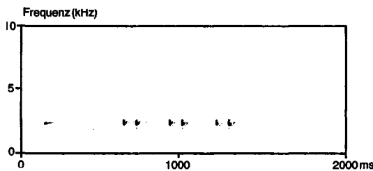
Abb. 9. Sonogramme von/sonograms of a) Mantidactylus aglavei (Ankeniheny) b) Mantidactylus fimbriatus (Andasibe) c) Mantidactylus fimbriatus (Marojezy) d) Mantidactylus phantasticus (An'Ala) e) Mantidactylus phantasticus (Andasibe).
