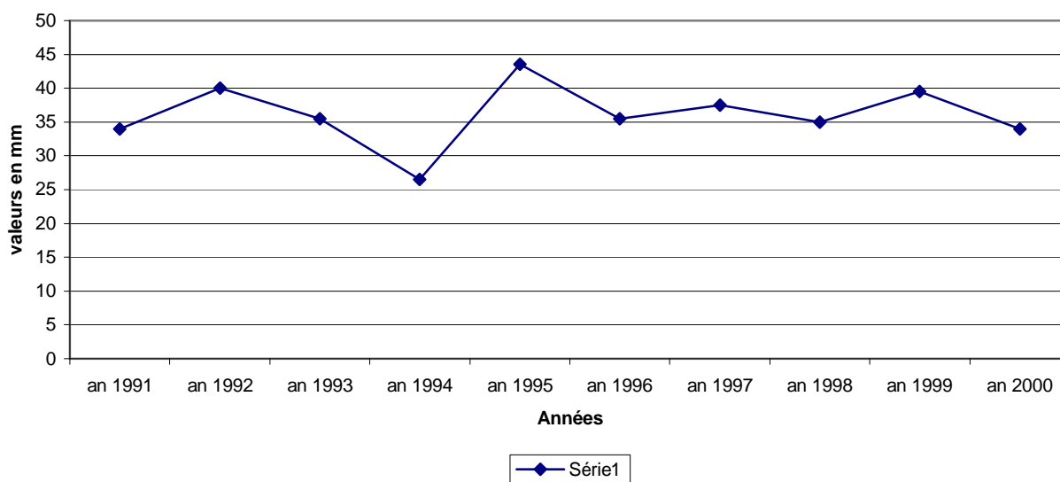
Evolution de l'humidité moyenne (période 1991-2000)
