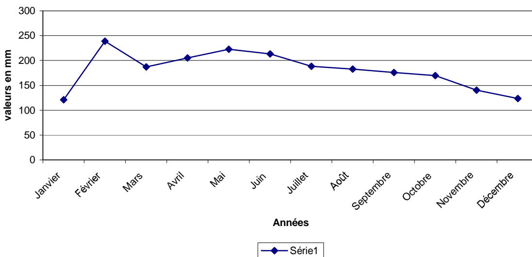
Moyenne mensuelle de l'évapotranspiration (période 1983-1992)
