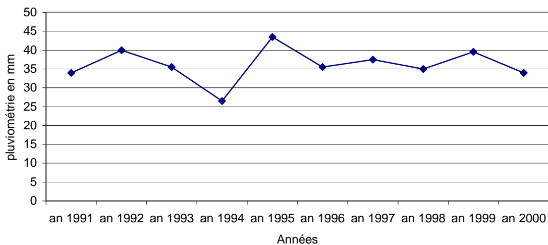
Pluviométrie moyenne annuelle période 1950-1999
