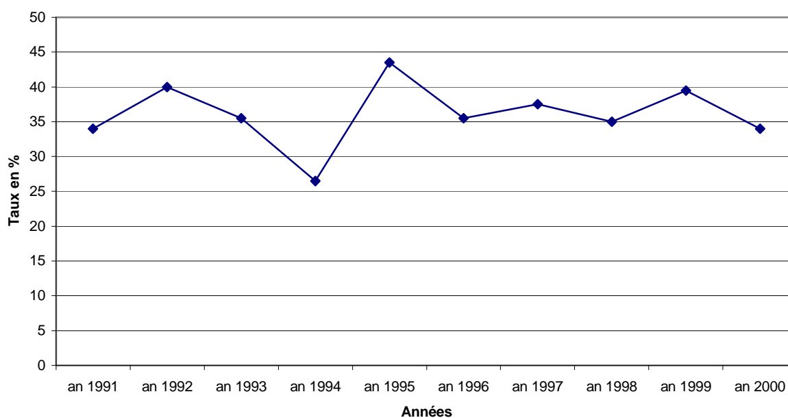
Taux d'humidité moyenne période 1991-2000
