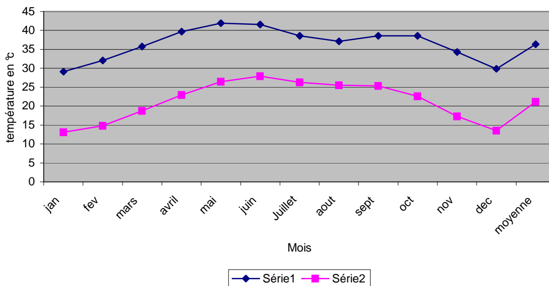
Evolution de la température (période 1971-2000)
