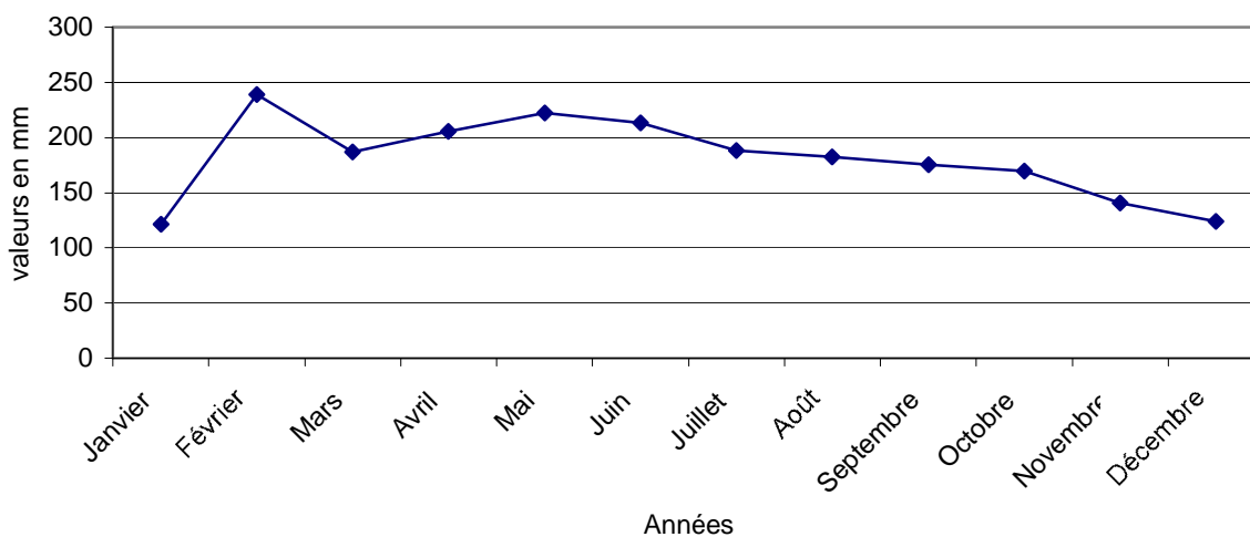
Moyenne mensuelle de l'évapotranspiration (période 1983-1992)
