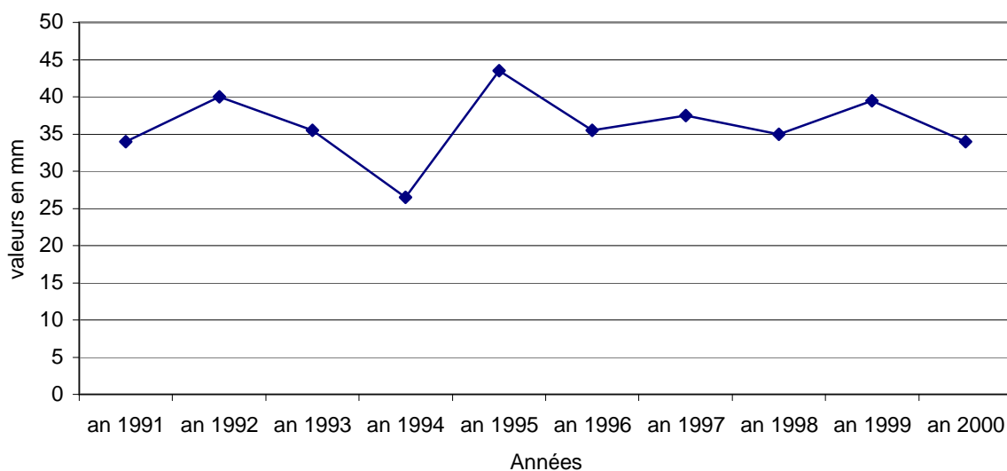
Evolution de l'humidité moyenne (période 1991-2000)
