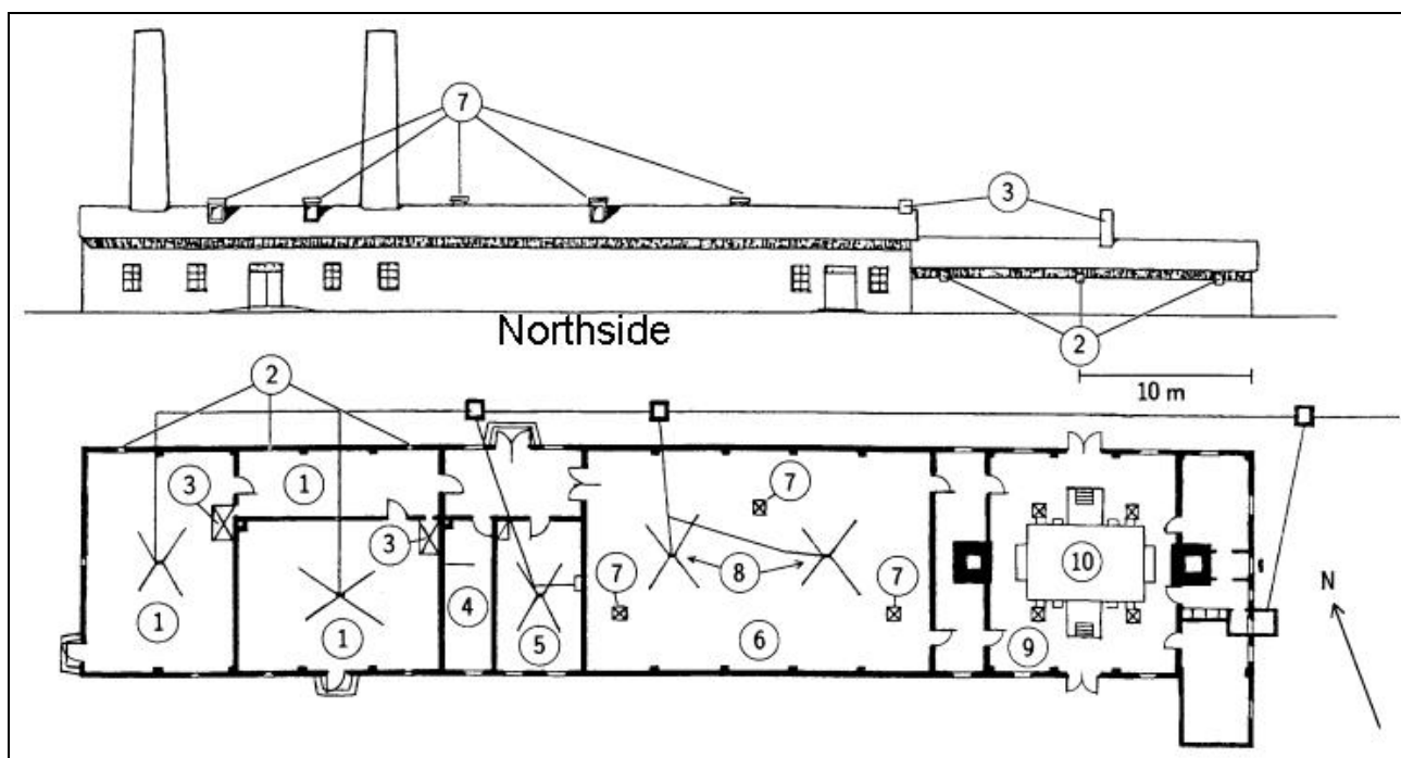
Рис. 123. Вид с севера и поэтажный план крематориев IV и V (зеркально симметричных) из лагеря Освенцим II (Биркенау).
