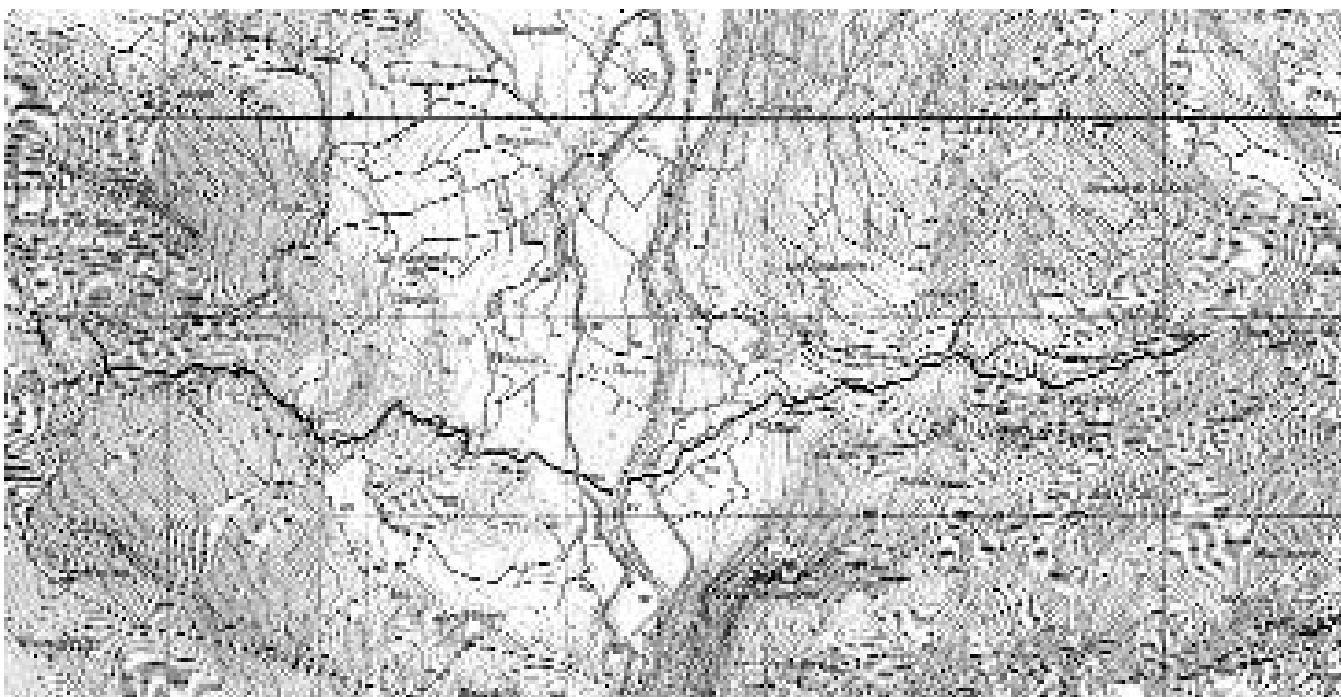
Els traços continus indiquen els trajectes naturals de les aigües de les fonts de Bordonera i de Codonyes (barrancs de Fontanet i l'Obac, respectivament). Els traços discontinus assenyalen les principals canalitzacions (A. Fiol)
