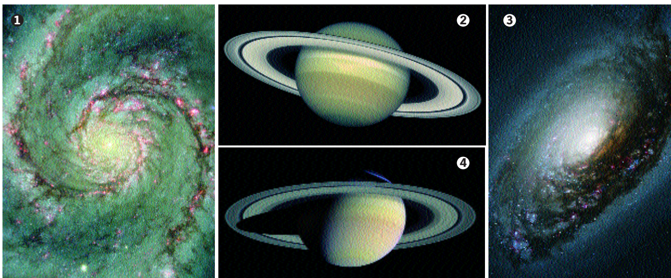
1.- La M-51, anomenada galàxia del remolí, es troba a 35 milions d'anys-llum, dins la constel·lació Canes Venatici. 2.- Foto telescòpica de Saturn, planeta que, juntament amb Mercuri, Venus, Mart i Júpiter, és visible a simple vista els mesos de primavera. 3.- La galàxia M-64, anomenada la de l'ull negre, és una de les més brillants del firmament i pertany a la constel·lació Coma Berenice. 4.- És una alternativa a la 33Cel02 (igual peu de foto), tria la millor.
