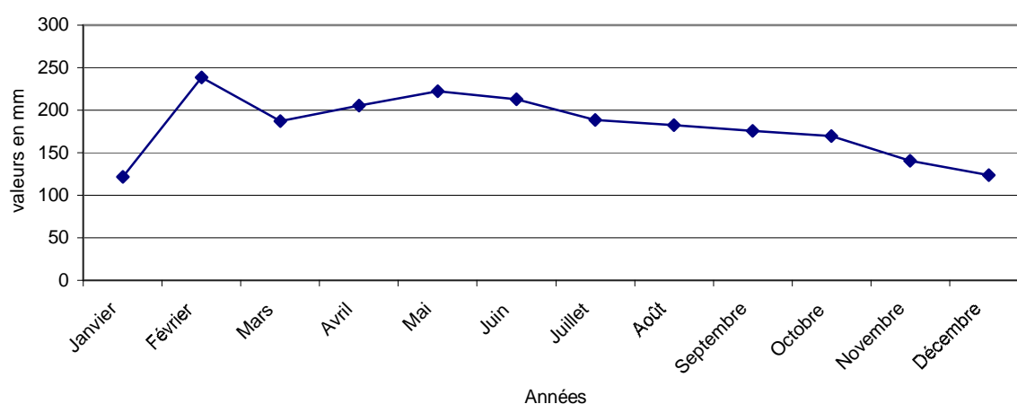
Moyenne mensuelle de l'évapotranspiration (période 1983-1992)
