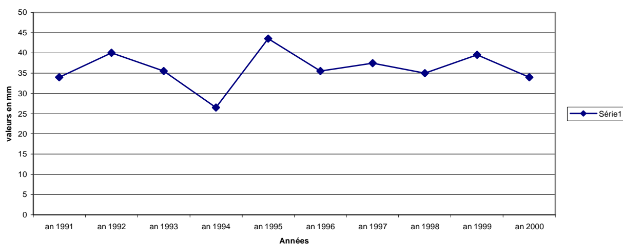
Evolution de l'humidité moyenne (période 1991-2000)
