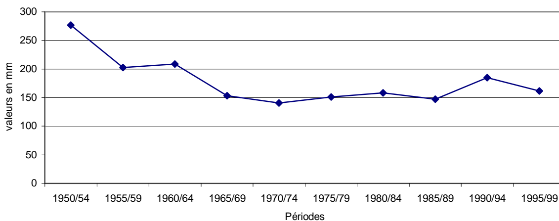
Pluviométries moyennes quinquennale de la période (1950-1999)
