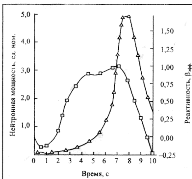
Рис. 16.1. Зависимость реактивности и нейтронной мощности от времени на начальной фазе развития аварии: \square — реактивность; \triangle — нейтронная мощность.
