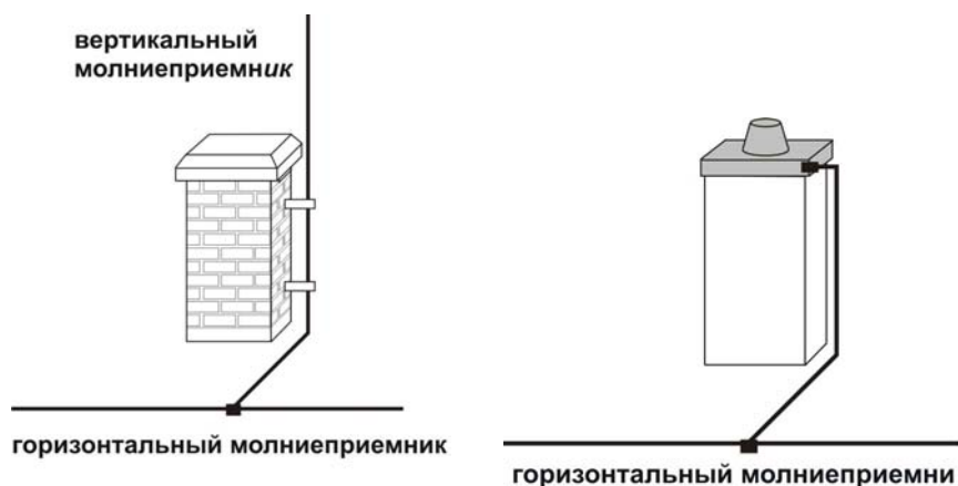
Рис. 17. Примеры защиты печных труб
