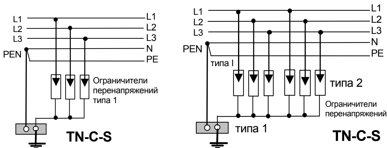
Рис. 21. Исключение расцепляющих элементов: а) схема ограничителей типа 1 с низким уровнем напряжения защиты, б) схемы соединения ограничителей типа 1 с низким уровнем напряжения защиты и ограничителей типа 2
