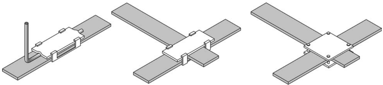
Рис.45. Различные примеры исполнения соединений элементов заземляющей системы
