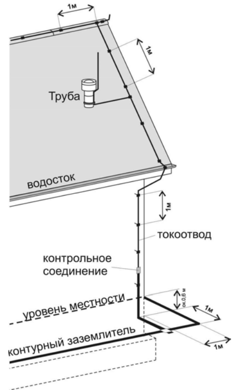
Рис. 42. Контурный заземлитель в строительном объекте a)общий вид, b) соединение заземлителя с заземляющим проводником
