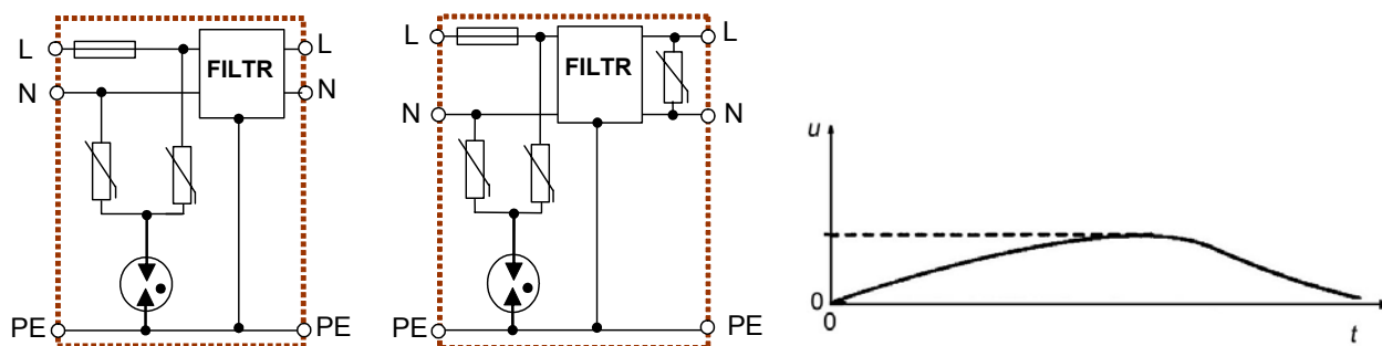
Рис. 23. Ограничитель перенапряжений типа 3 класса III с дополнительным фильтром, а, б) схемы систем ограничителей перенапряжений, в) временная диаграмма напряжения на выходе ограничителей
