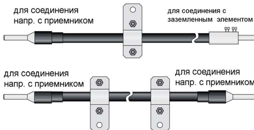
Рис. 24. Готовые токоотводы в изоляции высокого напряжения с различными концами и скобами для монтажа.
