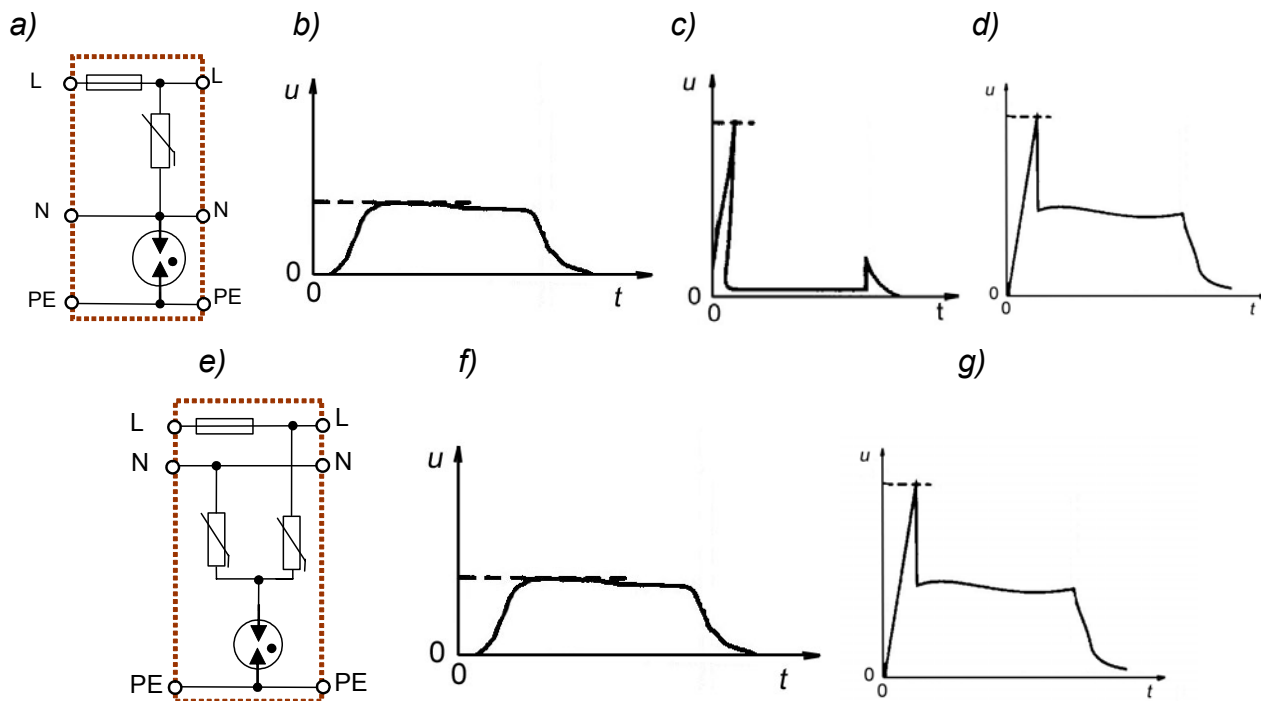
Рис.22. Ограничители перенапряжений типа 3; а),е)схемы типовых ограничителей, б),f ) напряжение между проводниками L и N, с ) напряжение между проводниками N и PE, d) напряжение между проводниками L и PE, г) напряжение между проводниками L и PE, а также N и PE.,
