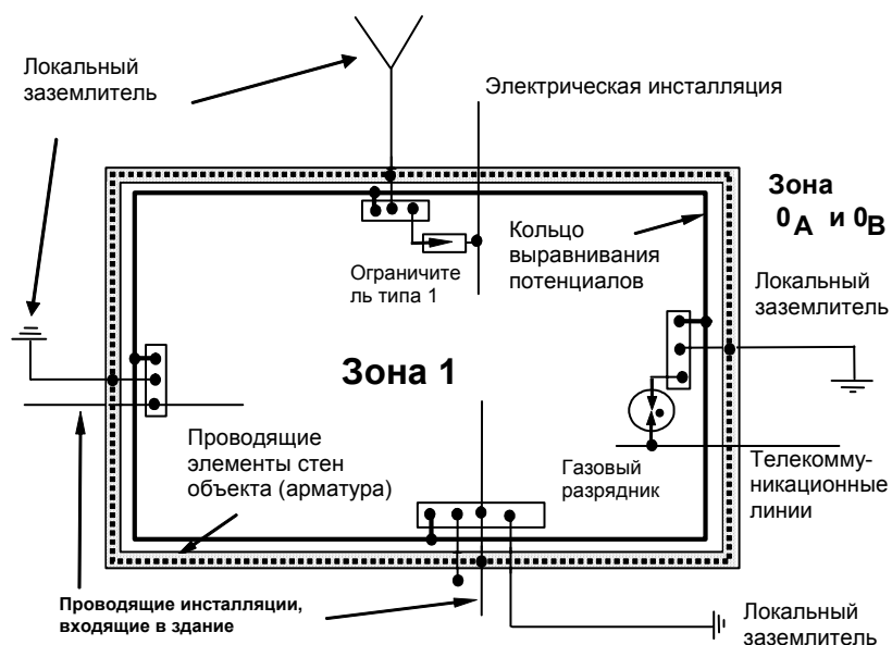
Рис. 52. Соединение шин между собой проводником, проложенным внутри или снаружи объекта
