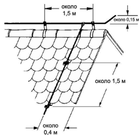
Рис. 28. Молниеприемники на двухскатных крышах. Размещение кронштейнов и примеры монтажа
