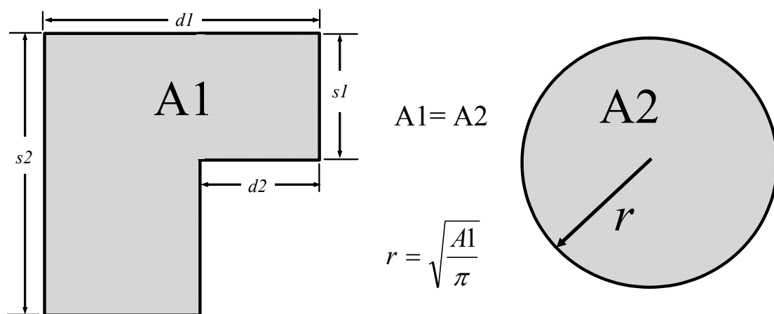
Рис 49. Определение заместительного радиуса r
