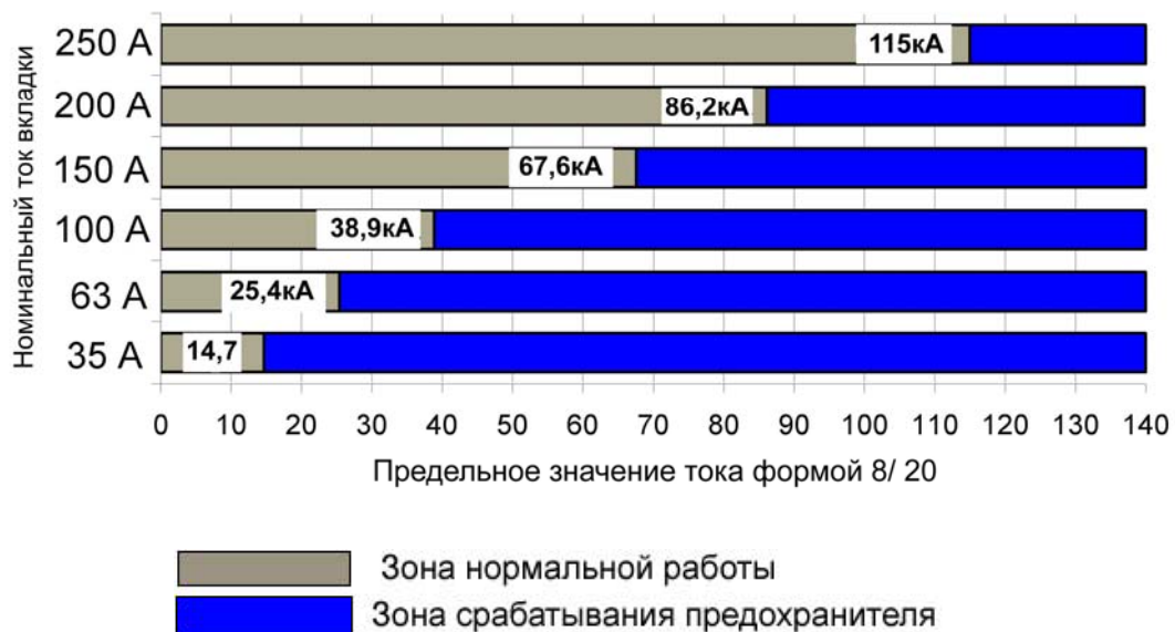
Рис. 16. Воздействие на предохранитель импульсного тока 8/ 20
