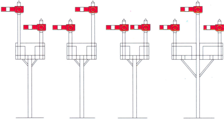
Tipi più comuni di segnali semaforici a candelieri
