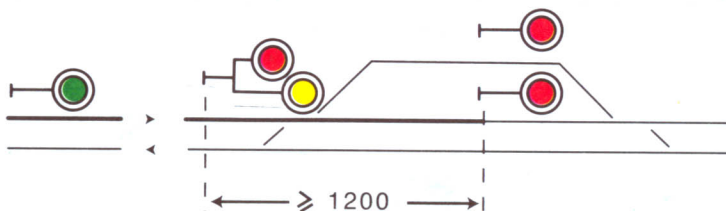
Ingresso in binario di corretto tracciato e fermata in stazione quando la distanza fra il segnale di protezione ed il segnale di partenza sia uguale o superiore a m. 1200.
