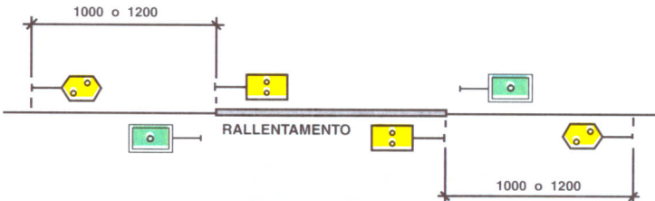
Rallentamento su linea a semplice binario
