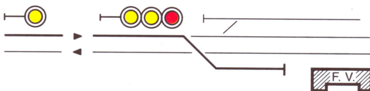
Ingresso in binario deviato tronco di limitata lunghezza.
