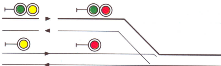
Transito in deviata su bivio preso di calcio.
