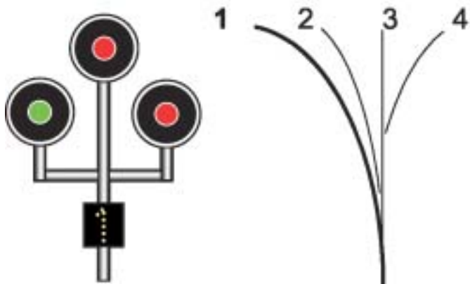
Segnale a candeliere integrato da indicatore, a via libera per la direzione 1.
