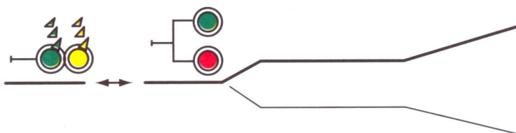
Transito su bivio simmetrico (riduzione di velocità a 60 km/h).
