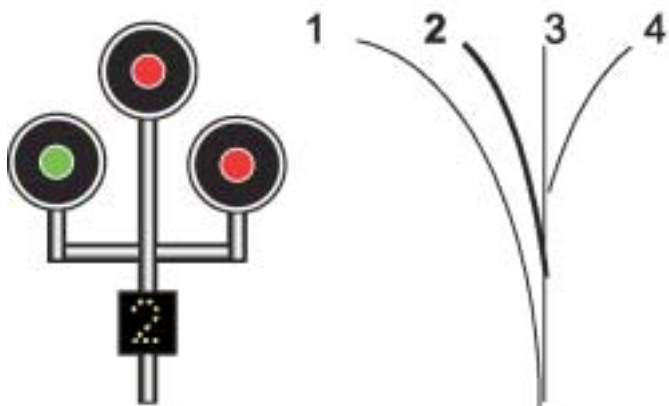
Segnale a candeliere integrato da indicatore, a via libera per la direzione 2.
