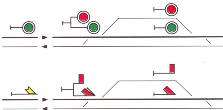
Transito su binario di corretto tracciato.
