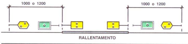
Rallentamento su linea a doppio binario interessante un solo binario
