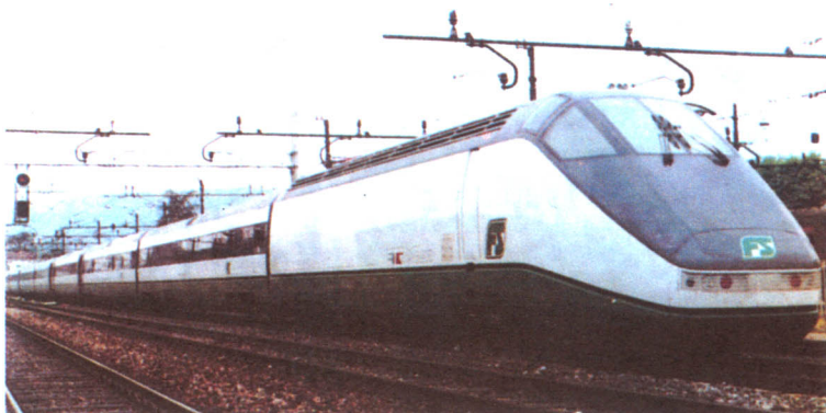
Configurazione di testa e di coda dell'ETR 500
