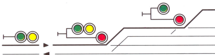
Transito per itinerario con due diramazioni successive aventi entrambe lo scambio disposto per il ramo deviato (riduzione velocità a 30 km/h).
