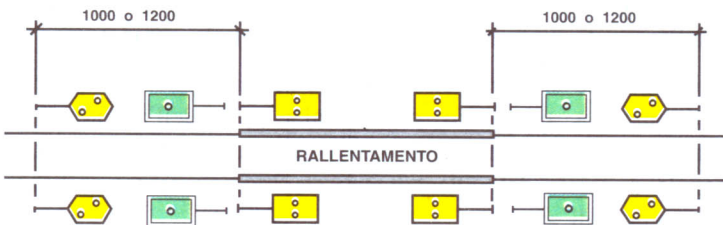
Rallentamento su linea a doppio binario interessante ambedue i binari
