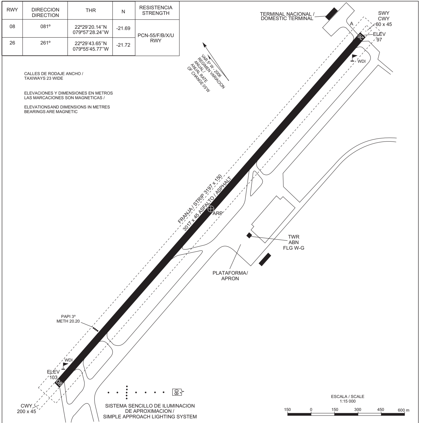
SEÑALES Y AYUDAS LUMINOSAS RWY 08/26 Y CALLES DE RODAJE DE SALIDA / MARKING AND LIGHTING AIDS RWY 08/26 AND EXIT TAXIWAYS
