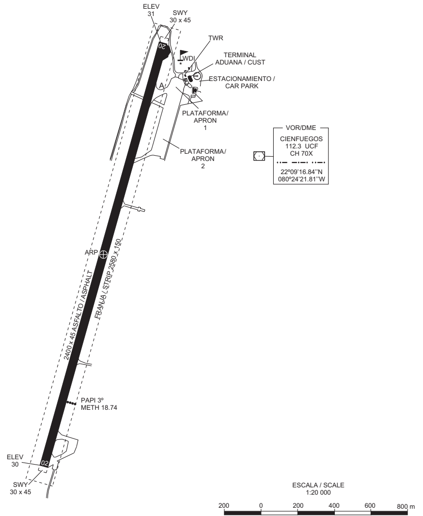
SEÑALES Y AYUDAS LUMINOSAS RWY 02/20 Y CALLES DE RODAJE DE SALIDA / MARKING AND LIGHTING AIDS RWY 02/20 AND EXIT TAXIWAYS
