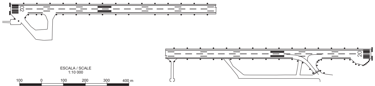
SEÑALES Y AYUDAS LUMINOSAS RWY 02/20 Y CALLES DE RODAJE DE SALIDA / MARKING AND LIGHTING AIDS RWY 02/20 AND EXIT TAXIWAYS
