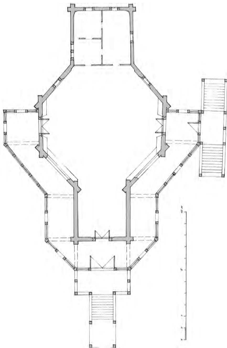
Рис. 6. Реконструкция плана Сретено-Михайловской церкви
