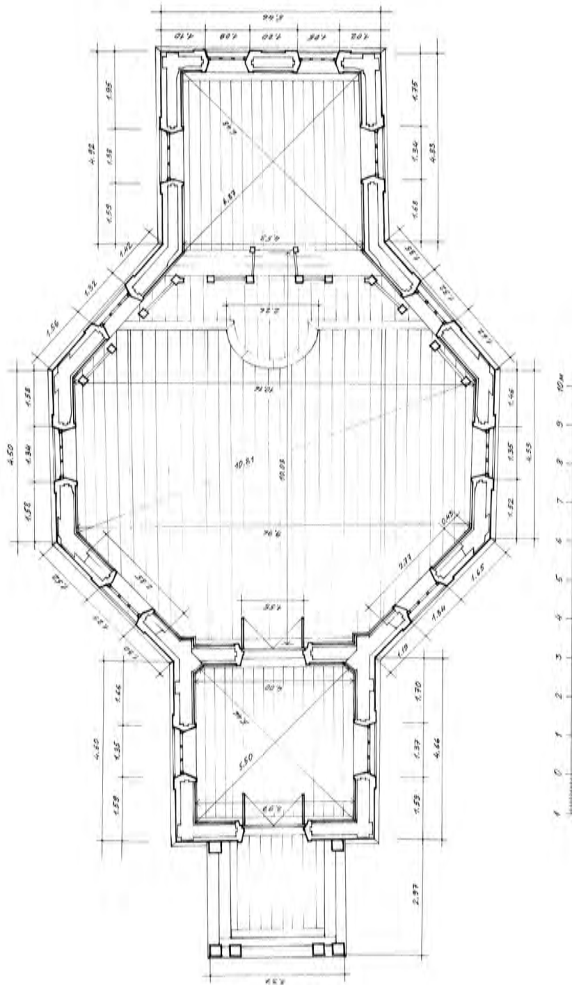
Рис. 2. План Сретено-Михайловской церкви. Обмеры А.Б.Бодэ и Г.Е.Дионисьевой, 2010 г.
