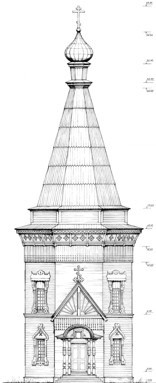
Рис. 3. Западный фасад. Обмеры А.Б.Бодэ и Г.Е.Дионисьевой, 2010 г.
