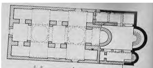
Η Μονή του Αποστόλου Βαρνάβα στη Σαλαμίνα και η κάτοψή της.
