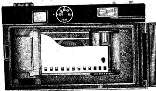
Рис. 5. Фотоаппарат с заряженной кассетой.
