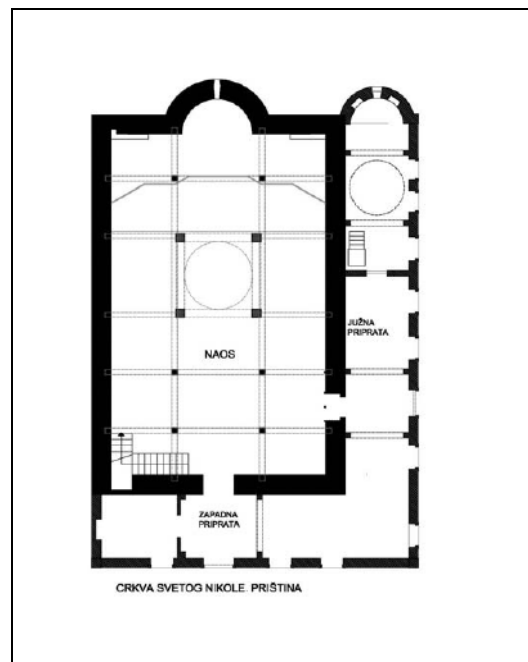
основа цркве
