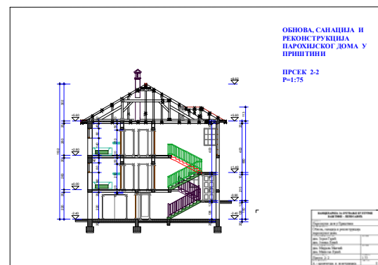
пресек
