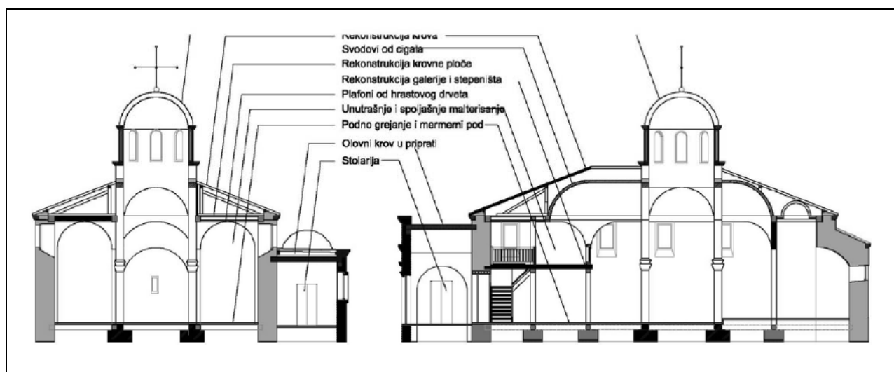
поречни и подужни пресек
