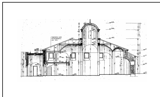
црква Светог Николе – оидужни пресек
