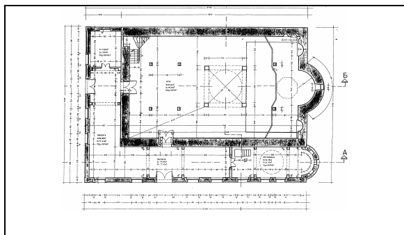
црква Светог Николе – основа приземља
