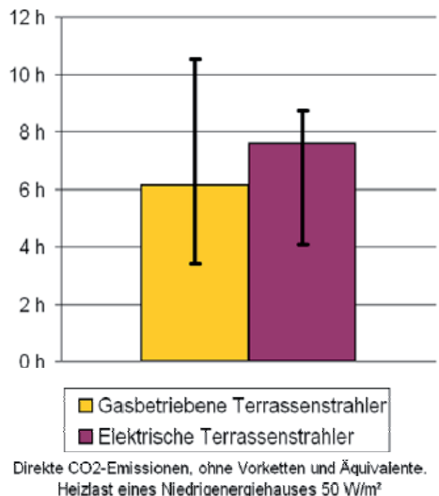
Abbildung 4: Heizdauer eines Heizstrahlers für einen gleich großen Raum eines Niedrigenergiehauses bei gleichem CO 2 -Ausstoß
