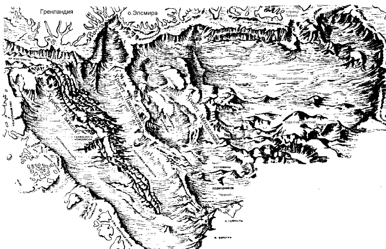
Карта подводных хребтов арктической области
