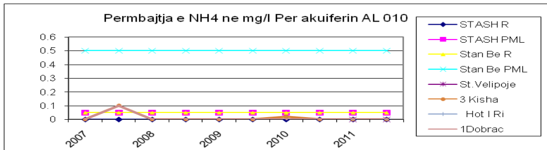
Fig nr. 2- Përmbajtja e \text{NH}_4 për akuiferin AL 010 2007-2011
