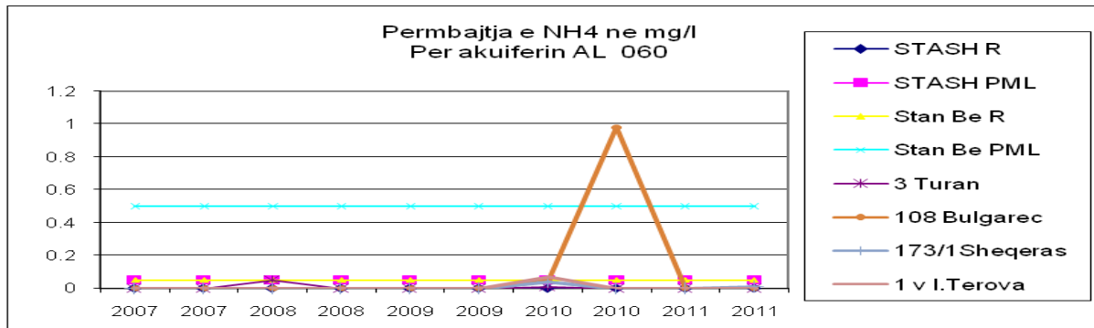
Fig.nr.27- Përmbajtja e NH 4 për akuiferin AL 060,2007-2011
