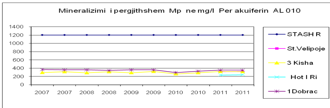
Fig. nr.1- Mineralizimi i përgjithshëm për akuiferin AL 010 2007-2011
