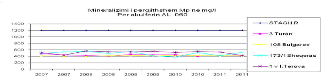
Fig. nr.26- Mineralizimi i përgjithshëm për akuiferin AL 060, 2007-2011
