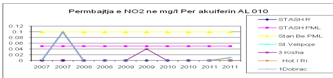
Fig. nr.3 - Përmbajtja e \text{NO}_2 për akuiferin AL 010 2007-2011
