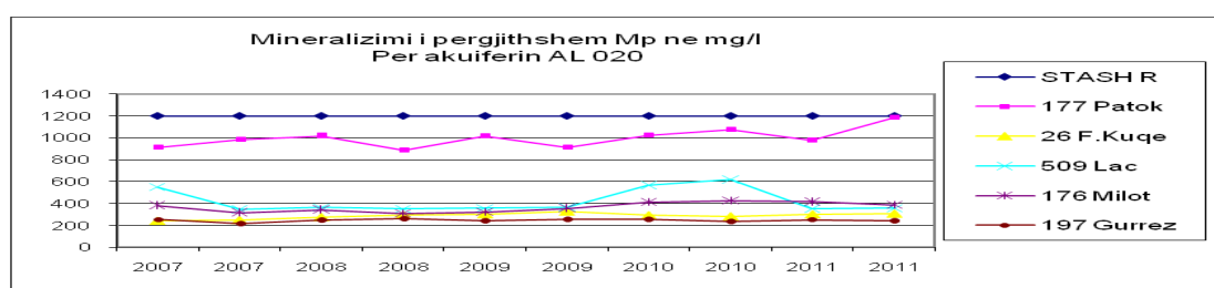
Fig. nr.10 Mineralizimi i përgjithshëm për akuiferin AL 020, 2007-2011
