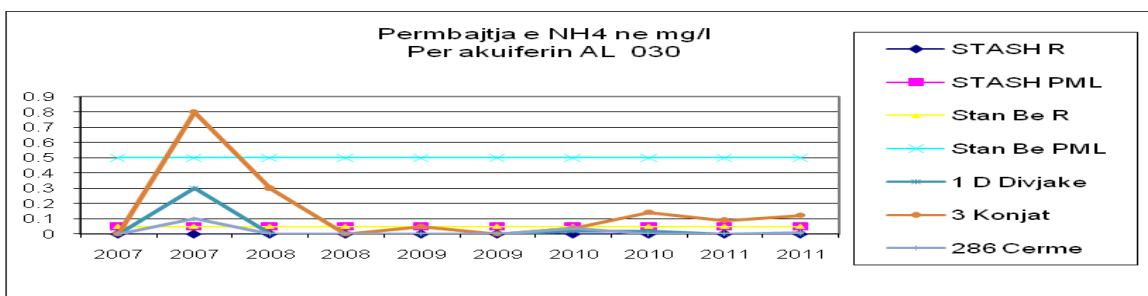
Fig.nr.24- Përmbajtja e \text{NH}_4 për akuiferin AL 030, 2007-2011
