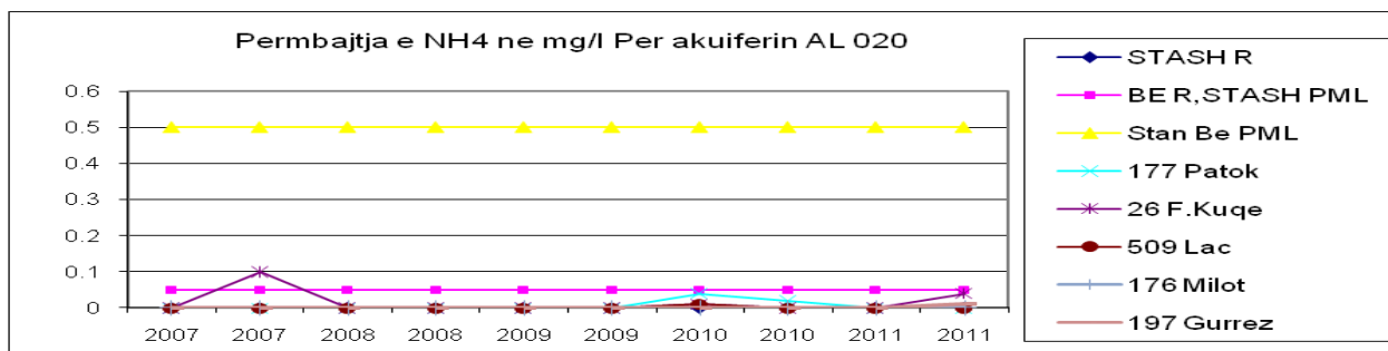
Fig. nr. 11- Permbajtja e NH 4 per akuiferin AL 020, 2007-2011
