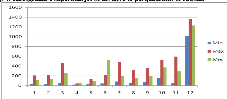
Fig. 4. Histograma e shpërndarjes së niveleve të përqendrimit të radonit
