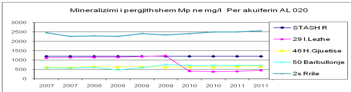
Fig. nr.4 - Mineralizimi i përgjithshëm për akuiferin AL 020, 2007-2011
