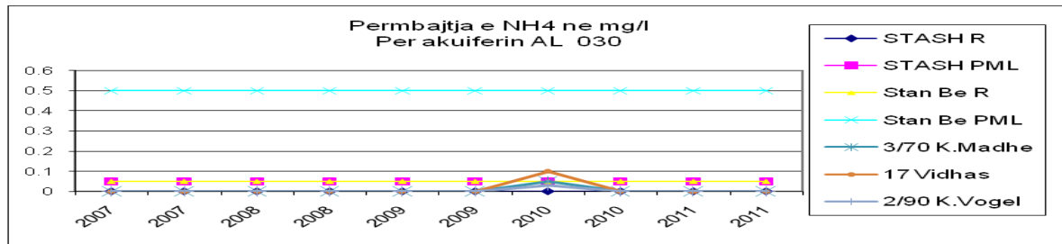
Fig. nr.22- Përmbajtja e NH 4 për akuiferin AL 030,2007-2011
