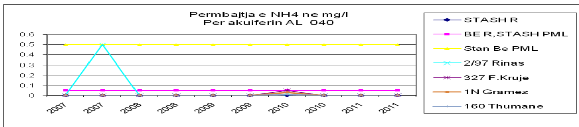
Fig.nr.19 - Përmbajtja e NH_4 për akuiferin AL 040, 2007-2011
