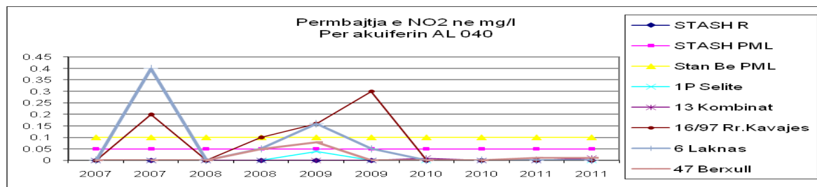
Fig.nr.17- Përmbajtja e \text{NO}_2 për akuiferin AL 040,2007-2011
