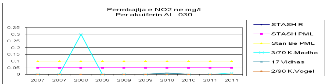
Fig. nr.23 Përmbajtja e NO 2 për akuiferin AL 030,2007-2011
