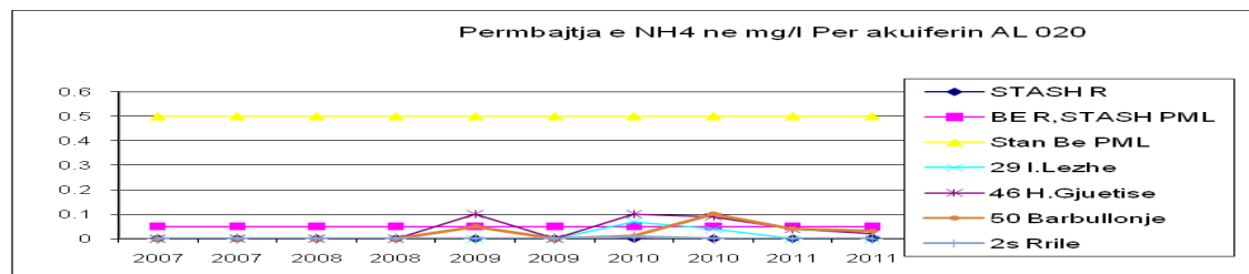
Fig. nr.5 - Përmbajtja e NH_4 për akuiferin AL 020, 2007-2011
