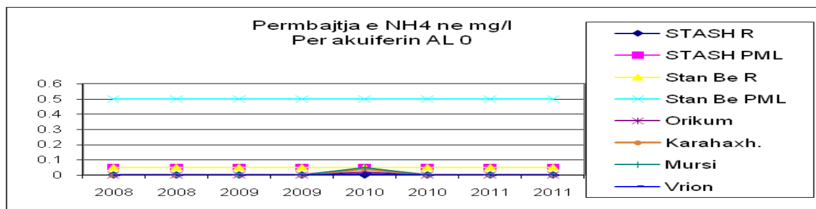
Fig.nr.33- Përmbajtja e NH 4 për akuiferin AL 070
