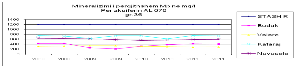
Fig. nr.29- Mineralizimi i përgjithshëm për akuiferin. AL 070,2007-2011
