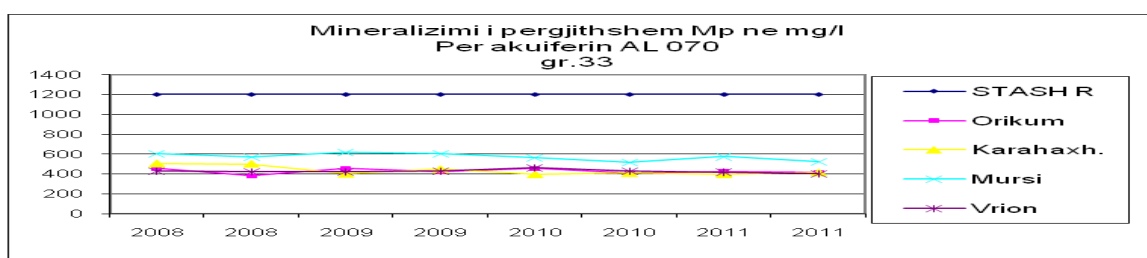
Fig. nr.32 Mineralizimi i përgjithshëm për akuiferin. AL 070
