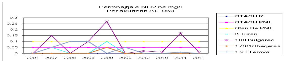
Fig. nr.28- Përmbajtja e NO 2 për akuiferin AL 060, 2007-2011
