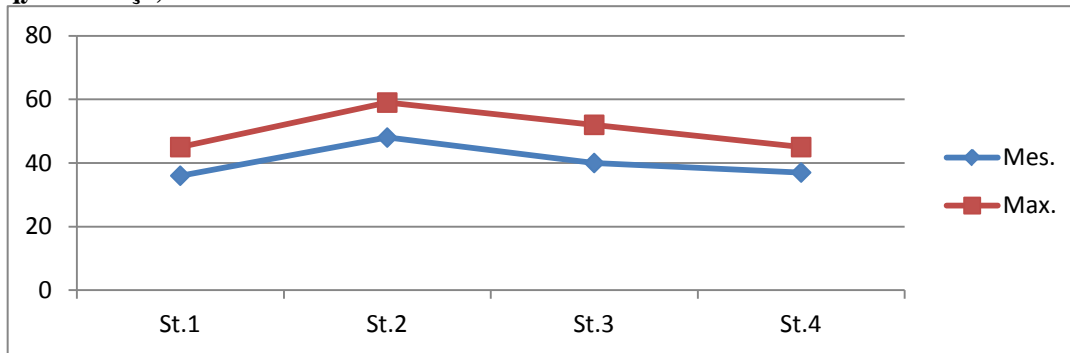
Graf. 7. Përqendrimit mesatare dhe maksimale të mesatarizuara, të niveleve të radonit në ujë, qyteti Korçë, viti 2011
