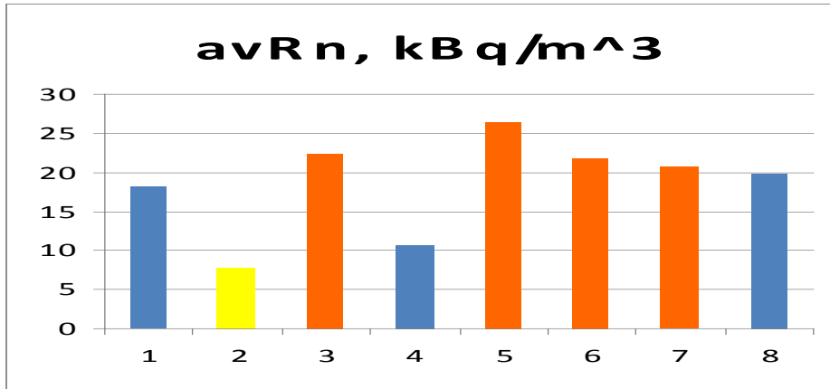
Fig.1. Histograma e shpërndarjes së niveleve të radonit në tokë
