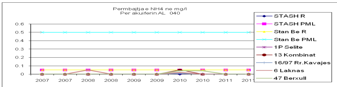
Fig. nr.16- Përmbajtja e \text{NH}_4 për akuiferin AL 040, 2007-2012
