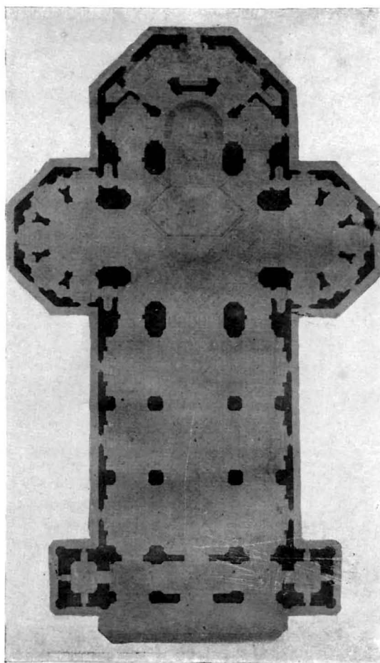
PROGETTO ALVINO, pianta.
