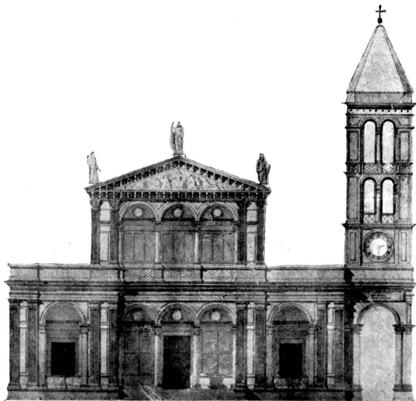
PROGETTO SAPONIERI (Prospetto).
