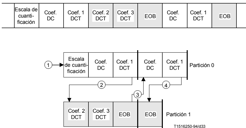
Figura 7-17 – Un segmento de un tren de bits con dos particiones, con punto de corte de prioridad puesto a 64 [un par (pasada, nivel)]. Se muestran las dos particiones con flechas que indican cómo el decodificador tiene que conmutar entre particiones
