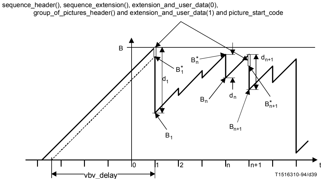
Figura C.1 – Ocupación de la memoria tampón VBV – Funcionamiento a velocidad binaria constante
