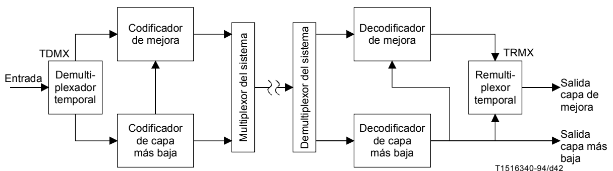
Figura D.1 – Estructura de un códec de dos capas para escalonabilidad temporal
