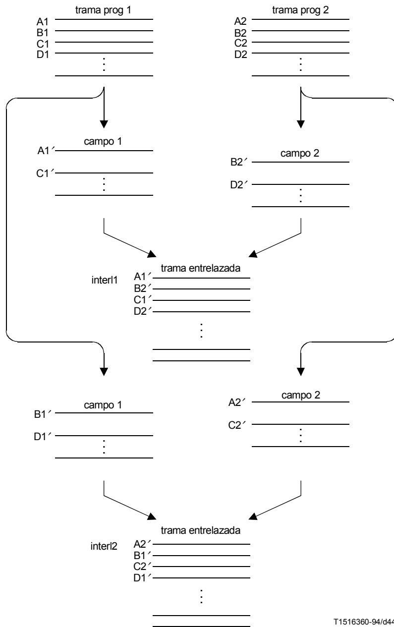
Figura D.3 – Conversión de trama progresiva a dos tramas entrelazadas
