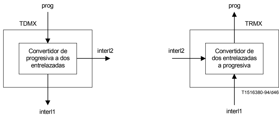
Figura D.5 – Demultiplexador temporal y remultiplexador temporal para trama progresiva – Escalonabilidad temporal de entrelazada a entrelazada
