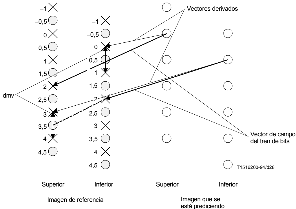
Figura 7-12 – Escalonamiento de vectores de movimiento para predicción dual-prima
