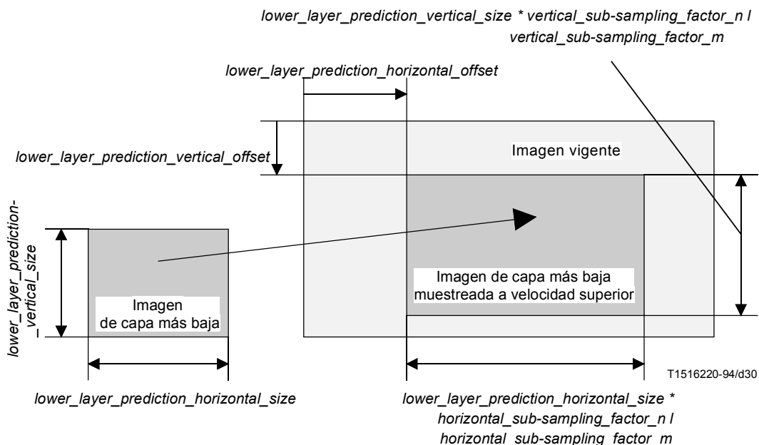
Figura 7-14 – Formación de la predicción "espacial" por interpolación de la imagen de capa más baja
