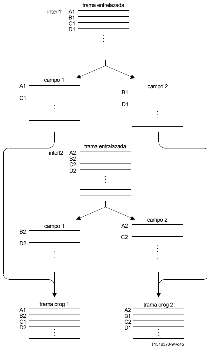
Figura D.4 – Conversión de dos tramas entrelazadas a trama progresiva
