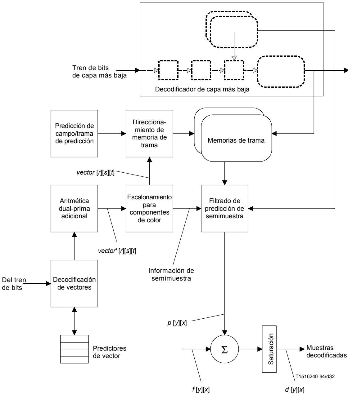
Figura 7-16 – Proceso de compensación de movimiento simplificado para la capa de mejora cuando se utiliza escalonabilidad temporal
