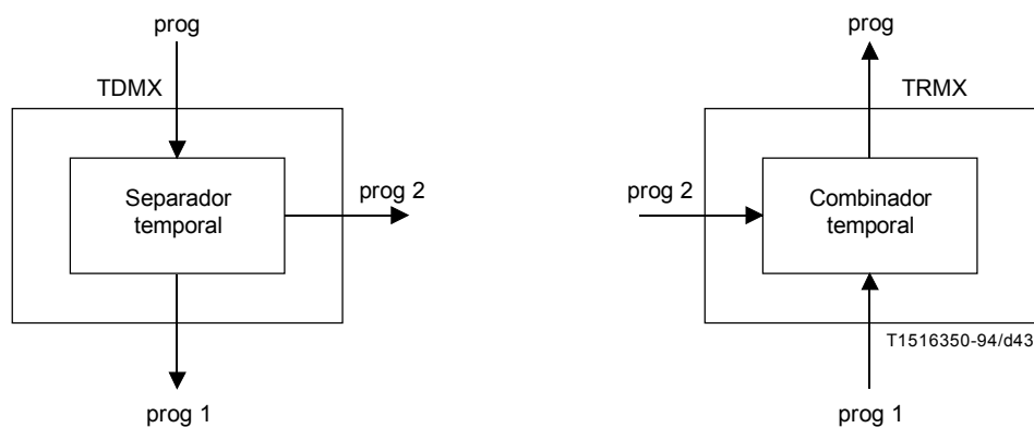
Figura D.2 – Demultiplexador y remultiplexador temporales para vídeo progresivo – Escalonabilidad temporal progresiva a progresiva
