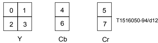
Figura 6-11 – Estructura de macrobloque de 4:2:2
