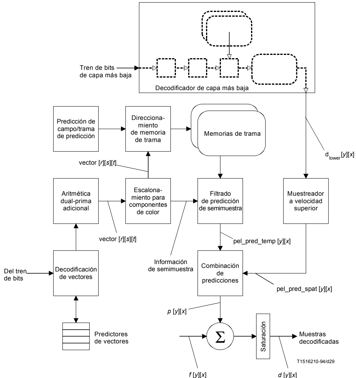
Figura 7-13 – Proceso de compensación de movimiento simplificado para escalabilidad espacial
