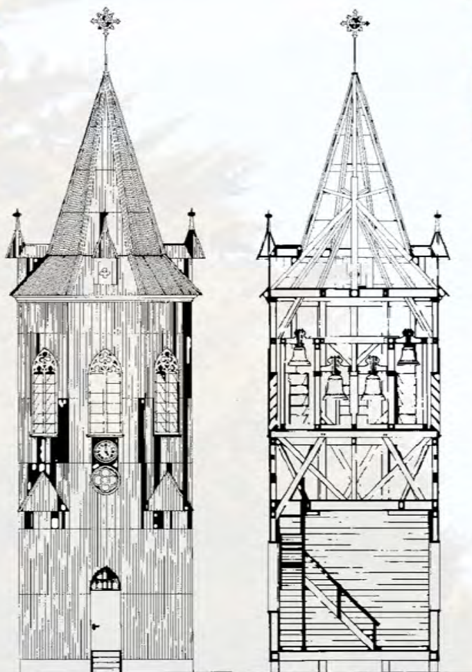
ELEVACIÓN FRONTAL
