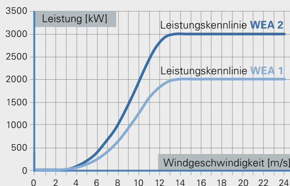
Abb. 10: Anlagenspezifische Leistungskennlinien von WEA 1 und WEA 2
