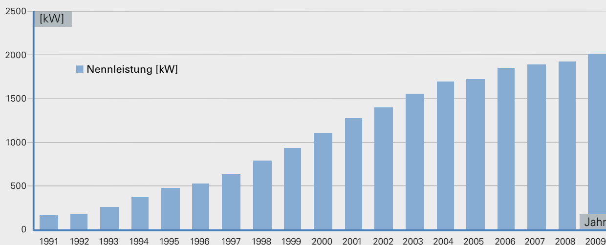
Abb 8: Entwicklung der mittleren Nennleistung [kW] von Windenergieanlagen in Deutschland (Quelle: DEWI 2009)
