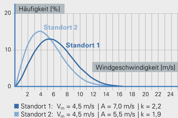
Abb. 9: Häufigkeitsverteilung der Windgeschwindigkeit für zwei unterschiedliche Standorte mit gleicher mittlerer Windgeschwindigkeit
