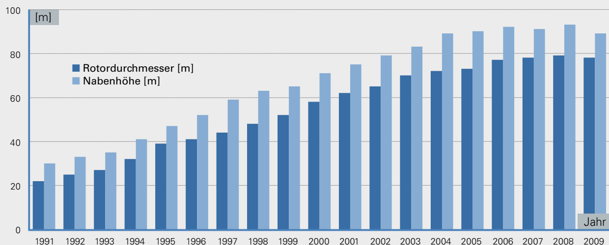
Abb 7: Entwicklung der Rotordurchmesser und Nabenhöhen von Windenergieanlagen in Deutschland (Quelle: Windenergie Report Deutschland)
