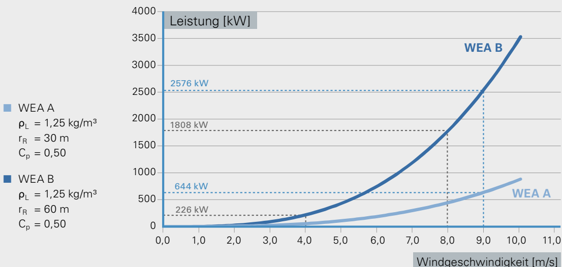
Abb. 6: Zusammenhang zwischen der Windgeschwindigkeit, dem Rotorradius und der Leistung für zwei Windenergieanlagen WEA A und WEA B
