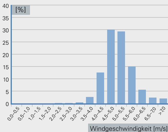
Abb. 5: Prozentuale Verteilung der mittleren jährlichen Windgeschwindigkeiten in Bayern, berechnet für 140 m Höhe (Zeitraum 1971 – 2000)
