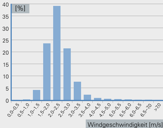
Abb. 3: Prozentuale Verteilung der mittleren jährlichen Windgeschwindigkeiten in Bayern, berechnet für 10 m Höhe (Zeitraum 1971 – 2000)
