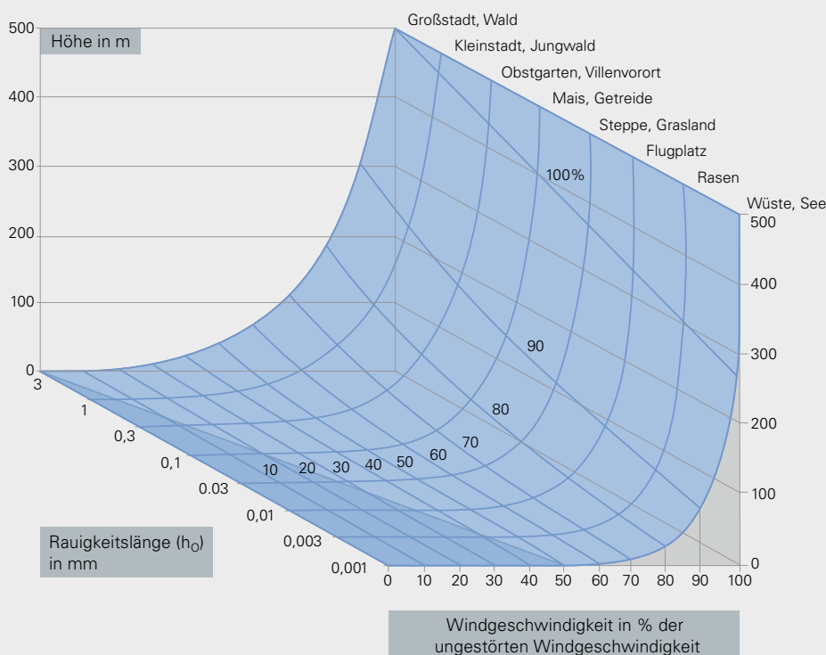
Abb. 1: Abhängigkeit der Windgeschwindigkeit von der Höhe und der Landoberfläche
