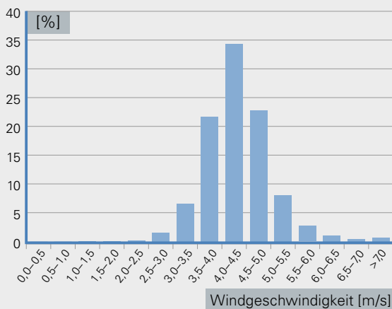
Abb. 4: Prozentuale Verteilung der mittleren jährlichen Windgeschwindigkeiten in Bayern, berechnet für 80 m Höhe (Zeitraum 1971 – 2000)
