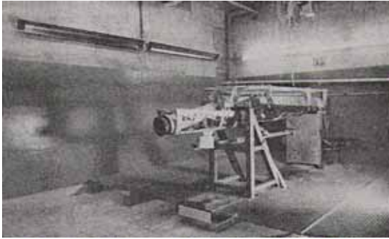
Raketentriebwerk „SEPR“ auf dem Prüfstand
