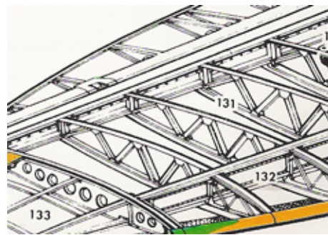
Rippen aus gepressten Blechen
