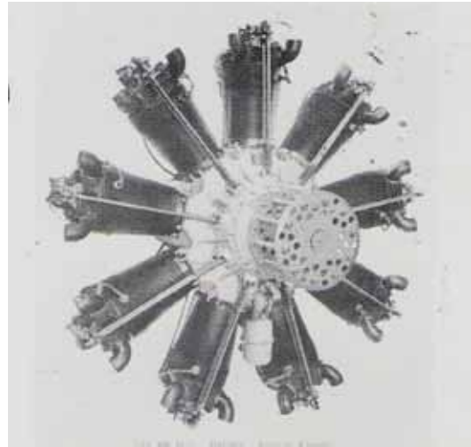
„Jupiter“ 9 AB: 420 PS. (Potez L-25 A-2). Von der Firma Saurer in Lizenz gebaut.
