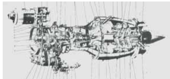
„Artouste“ III, Schnitt.
