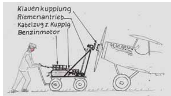
„Anlasswagen“ („Patent“ Ing. Burkhardt)
