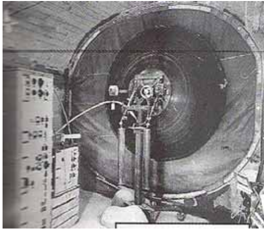
1957: Richtstrahlanlage BBC. Blick von der Kaverne aus auf die Hinterseite der Parabolantenne
