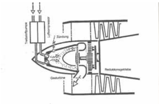
„Hunter“, Plessey-Starterturbinen
