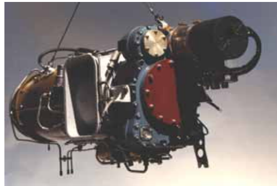
„Artouste“ III B: 550 PS. („Alouette III“)
