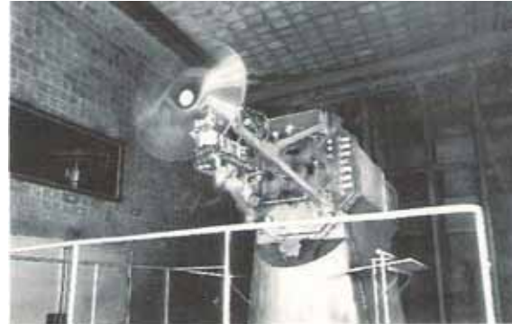
Hirth HM-504 auf dem Prüfstand
