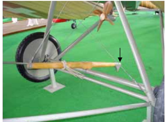
DH-1: Vom Pilotensitz aus per Kabel bedienter „Bremshebel“.
