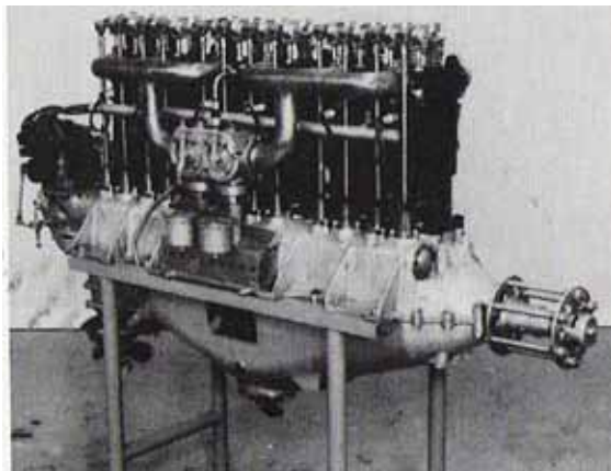
Argus AS II: 120 PS (Flugzeug Wild). Lizenzbau bei der Firma Gebr. Bühler, Uzwil.
