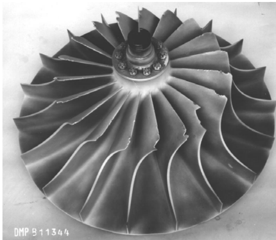
„Ghost“: Impeller, beschädigt durch eingedrungene Fremdkörper ...
