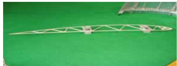
Rippe aus Alu-Röhrchen aufgebaut (D-27)
