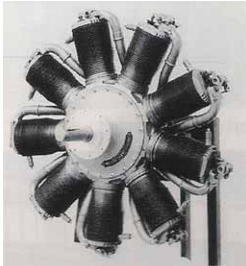
Le Rhône JB: Umlaufmotor, 110 PS (Blériot) Der Motor dreht samt Propeller um die fest stehende Kurbelwelle.
