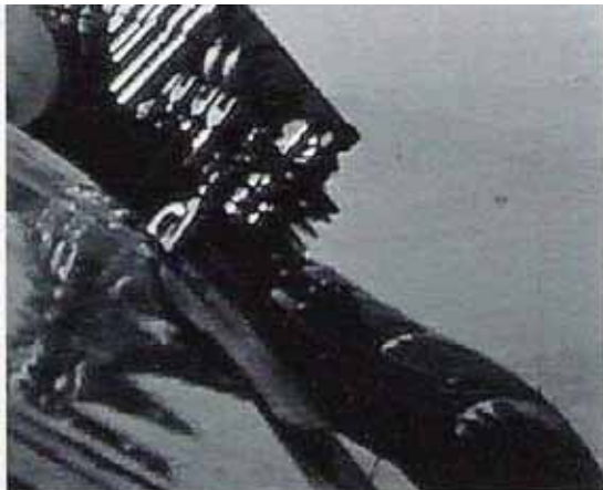
DH-5: Die offenen, im Luftstrom liegenden Kipphebel des LFW (vom Pilotensitz aus gesehen)
