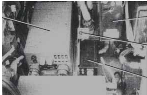
IFF, Freund-Feind-Erkennungsgerät (Transponder) Eingebaut in der Elektronikbucht
