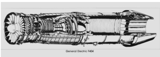
F 404: Schnitt
