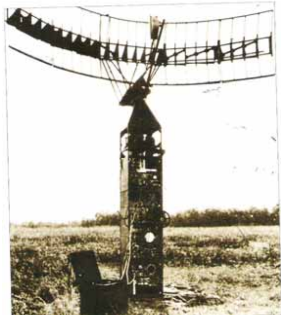
1950: Radaranlage Bendix LGR-1
