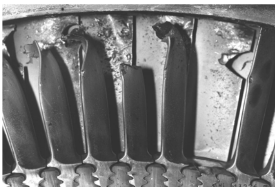
„Ghost“: ... und in der Folge beschädigte Turbinenschaufeln.
