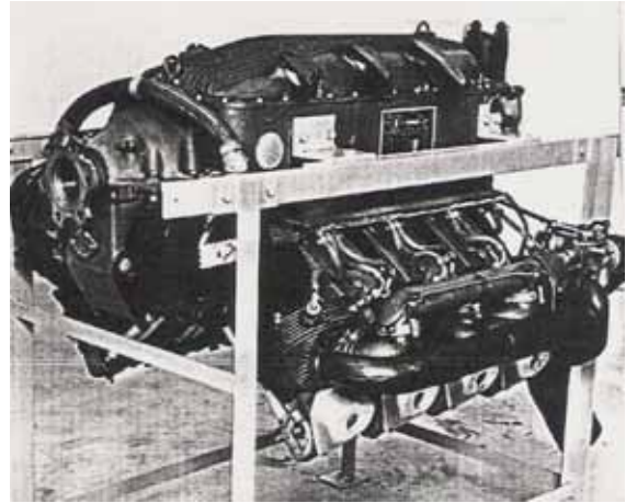
Argus AS-10: 220 PS. (ME- 108 „Taifun“ und Fieseler „Storch“)
