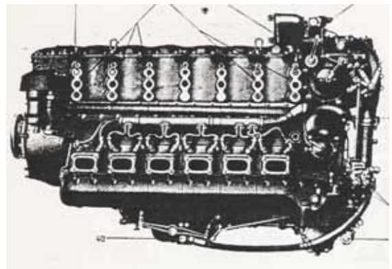
„Jumo“ 210: 680 PS. (Me -109D „David“)
