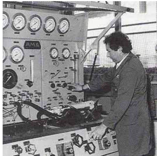
Prüfung eines Hydraulikgerätes auf dem Prüfstand
