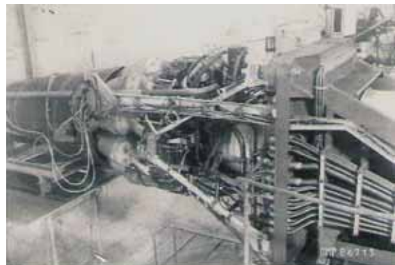
Motorenprüfstand mit Ghost
