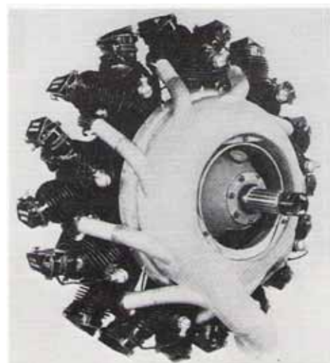
Wright „Whirlwind“ R-975: 250 PS (D-26)
