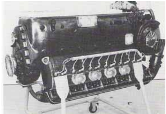
DB- 601 Aa: 1100 PS (Me -109E)
