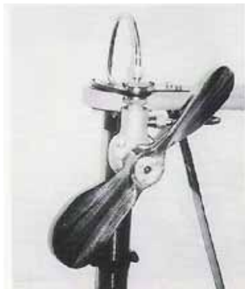
Blériot: Luftgetriebene Benzinpumpe (vom Rumpftank zum Flügeltank).
