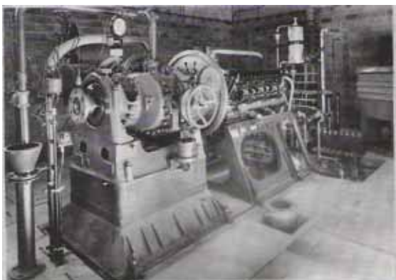
HS-51 auf der Wasserbremse
