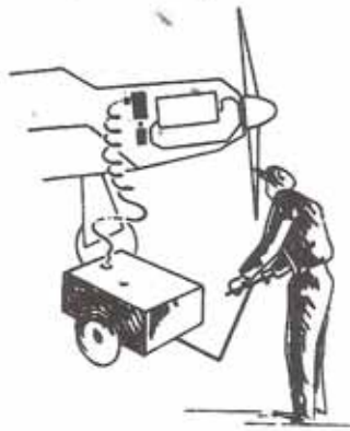
Anlassen elektrisch ab Batteriewagen
