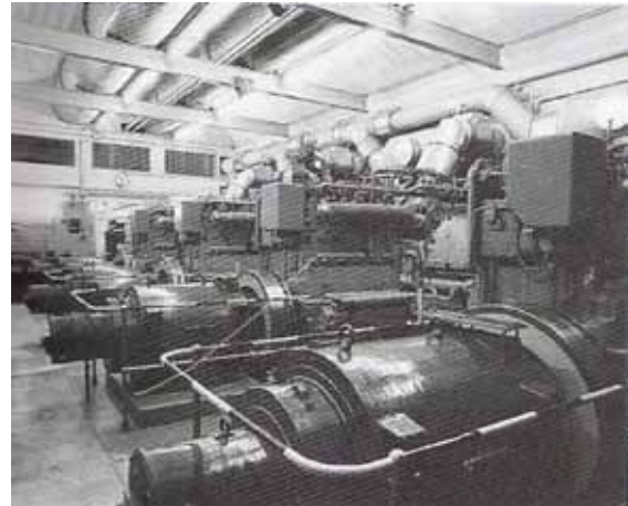
Notstromanlage auf einem Radarberg: Diese muss bei Stromausfall den unterbrochenslosen Betrieb gewährleisten
