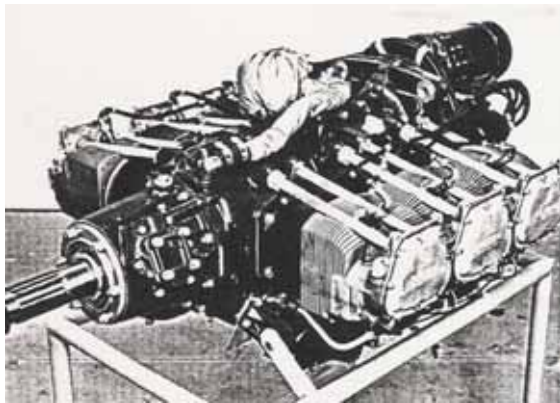
Lycoming GSO-480: 320PS (Do-27und PC6). Beim Flz PC-6 wurden später die GSO-480 durch die Propellerturbine P+W PTA-27 ersetzt. (siehe Seite 13).
