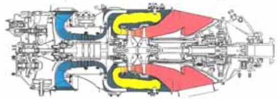
PTA-27. Schnitt
