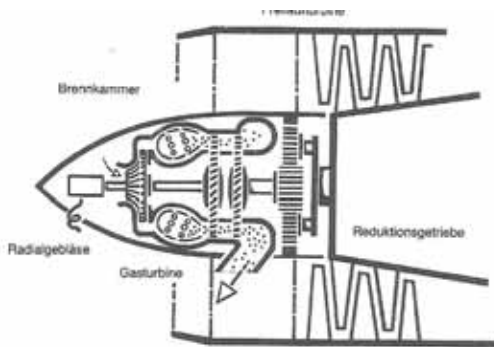
Mirage III S . „Noelle“- Starterturbine. Sie lief mit normalem Flugpetrol
