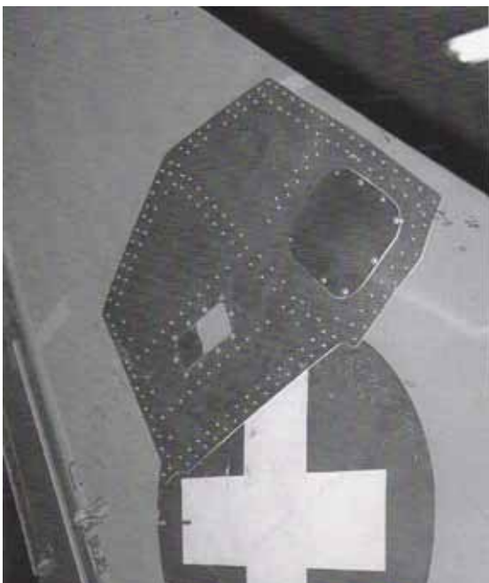
Reparatur an der Kielfläche eines Flugzeugs „Hunter“ durch die Truppe
