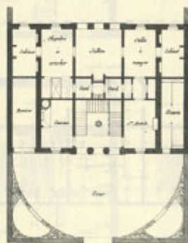
Plan au niveau de la Rue.
