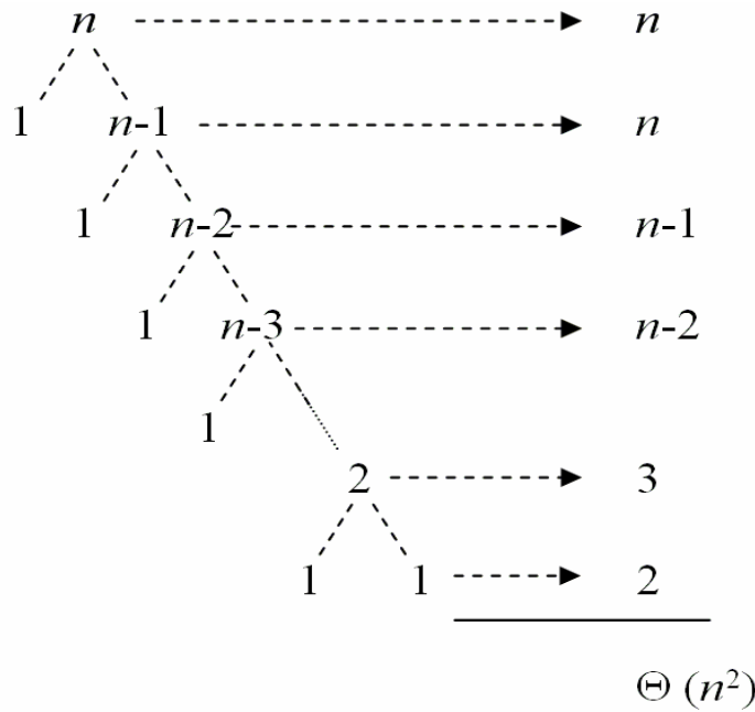
Рис. 2.9. Приклад незбалансованого розбиття
