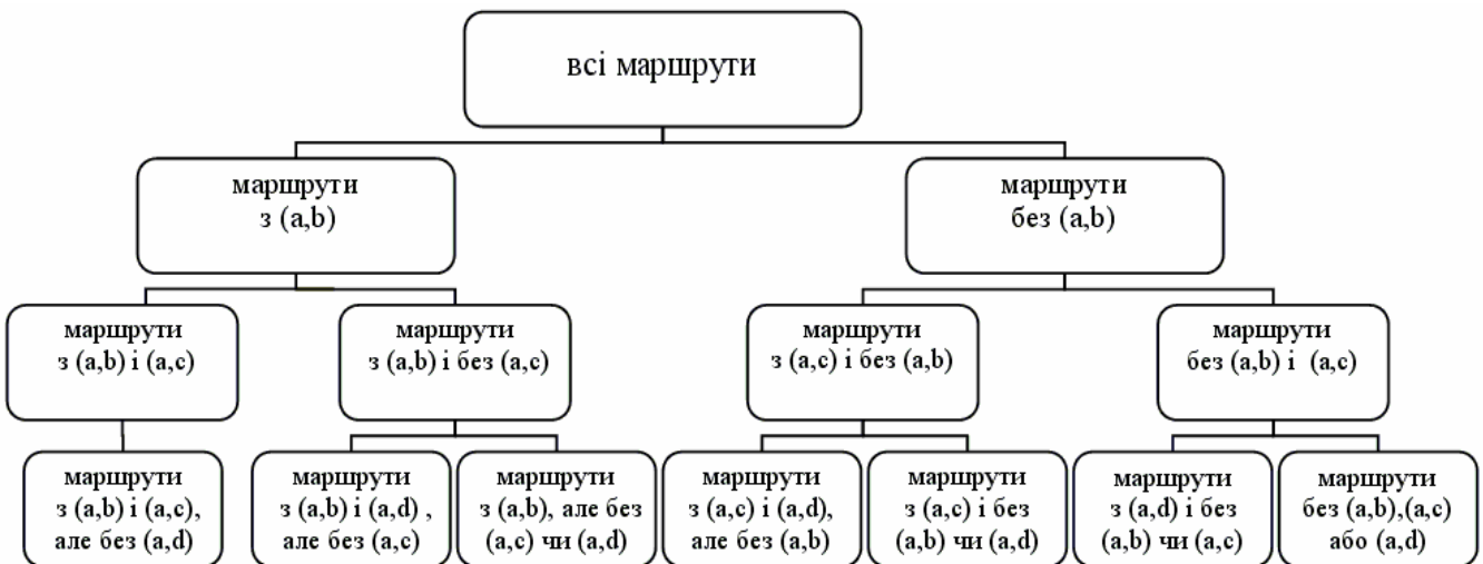
Рис. 2.12. Фрагмент дерева рішень повним переглядом для задачі комівояжера
