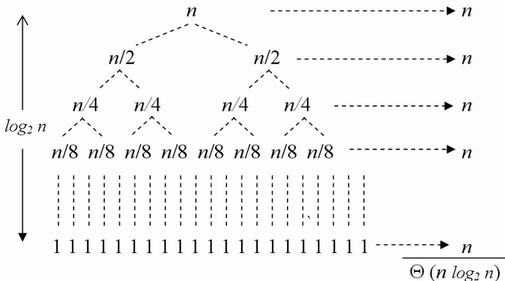
Рис. 2.10. Приклад збалансованого розбиття
