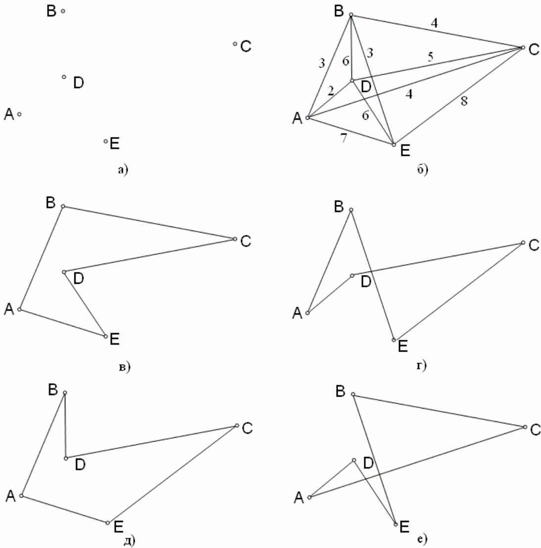
Рис. 2.11. Приклади побудови маршрутів для задачі комівояжера
