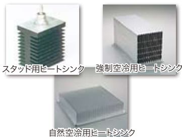
自然空冷用ヒートシンク
