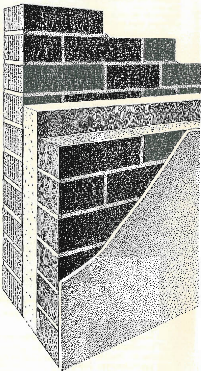
Den högisolrande kanalväggen består utifrån sett av 1/2 -sten fasadtegel, plastad platta eller matta av mineralull samt en inre bärande väggdel av vanligt murtegel som putsas. Tjockleken hos den inre väggdelen får givetvis anpassas med hänsyn till påkänningarna i varje särskilt fall. I t. ex. ett normalt 3-våningshus utföres den inre väggdelen av 1/2 -sten tegel i översta våningen och i de två nedersta våningarna är det vanligen tillräckligt med en 14 cm tjock väggdel.
