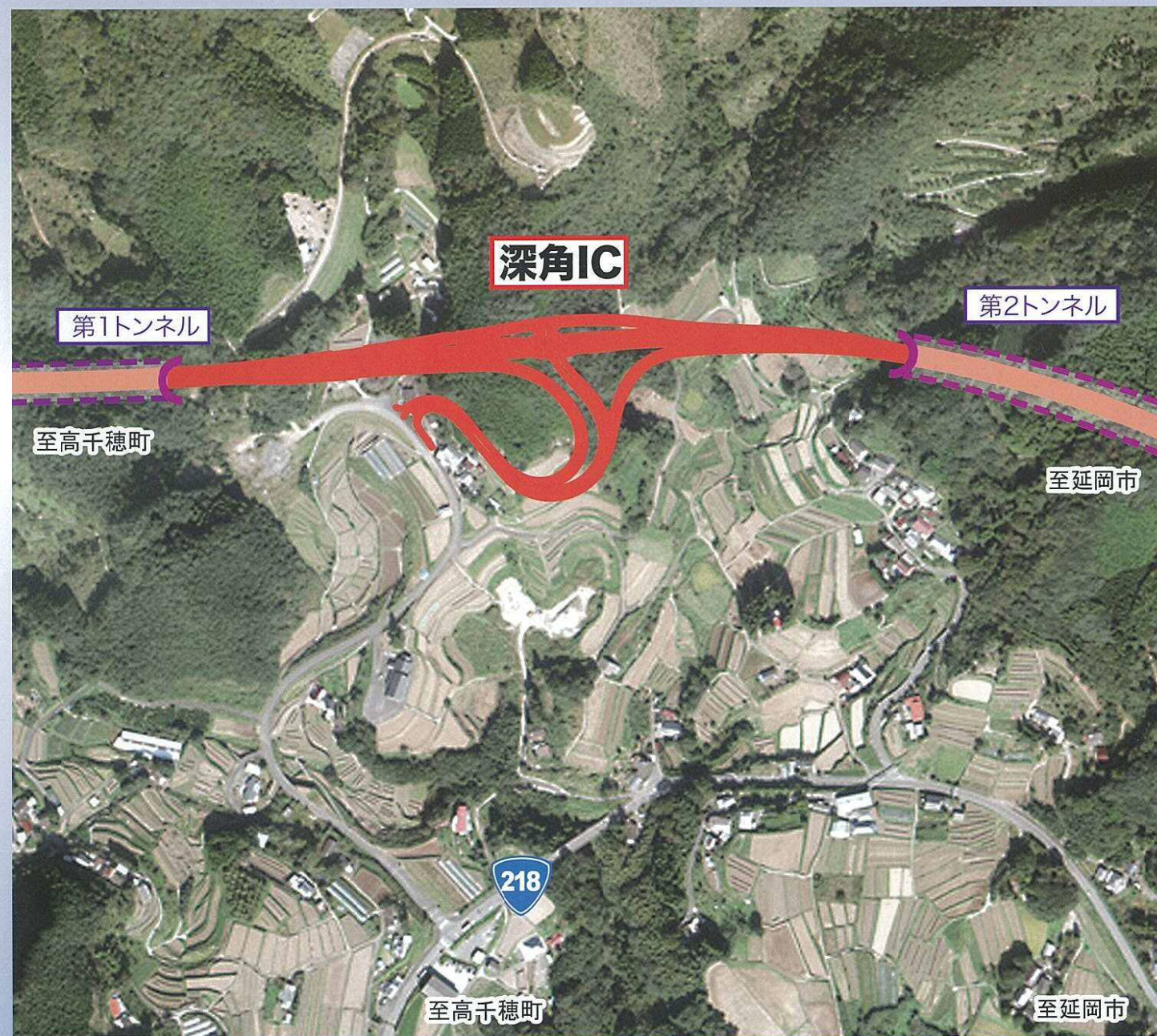
完成予想イメージ図 (航空写真:平成23年3月5日撮影) ※IC名、トンネル名は仮称
