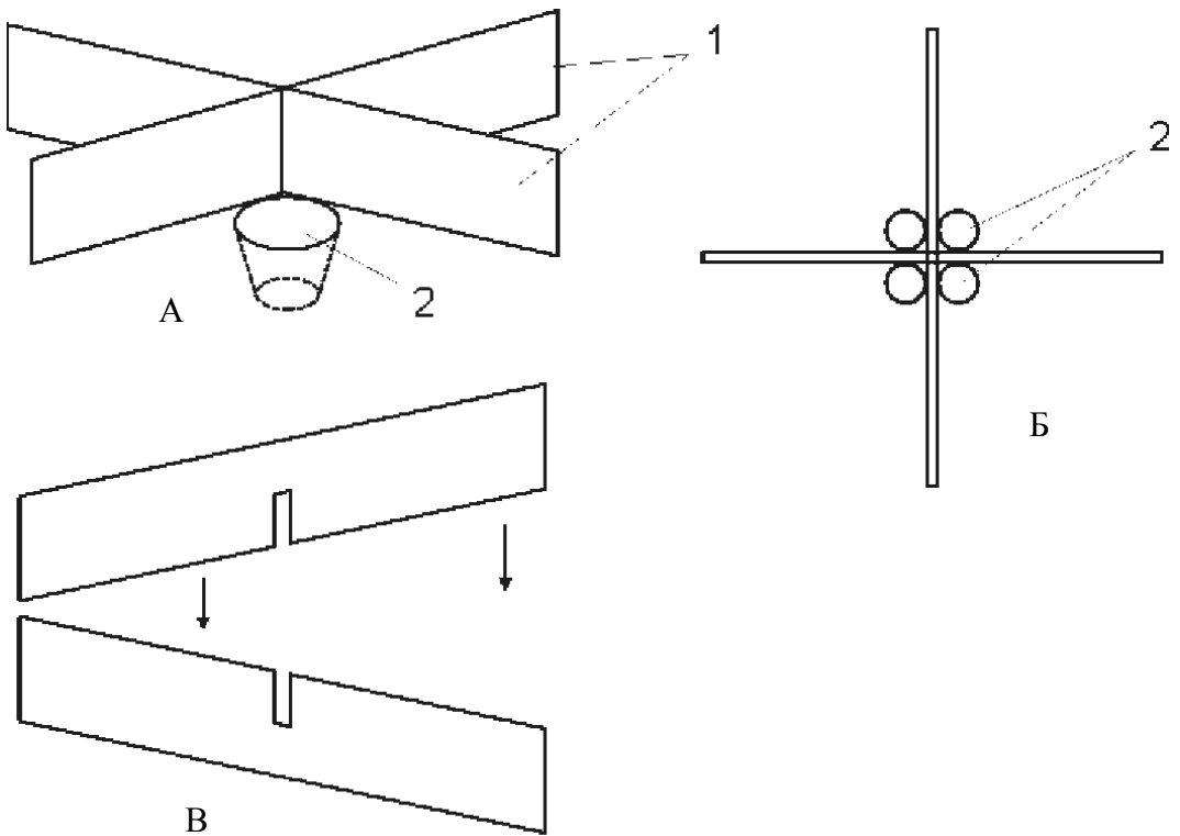
Рис. 17. Чотирьохсекторна міграційна пастка (за Цуриков, Цуриков, 2001)
