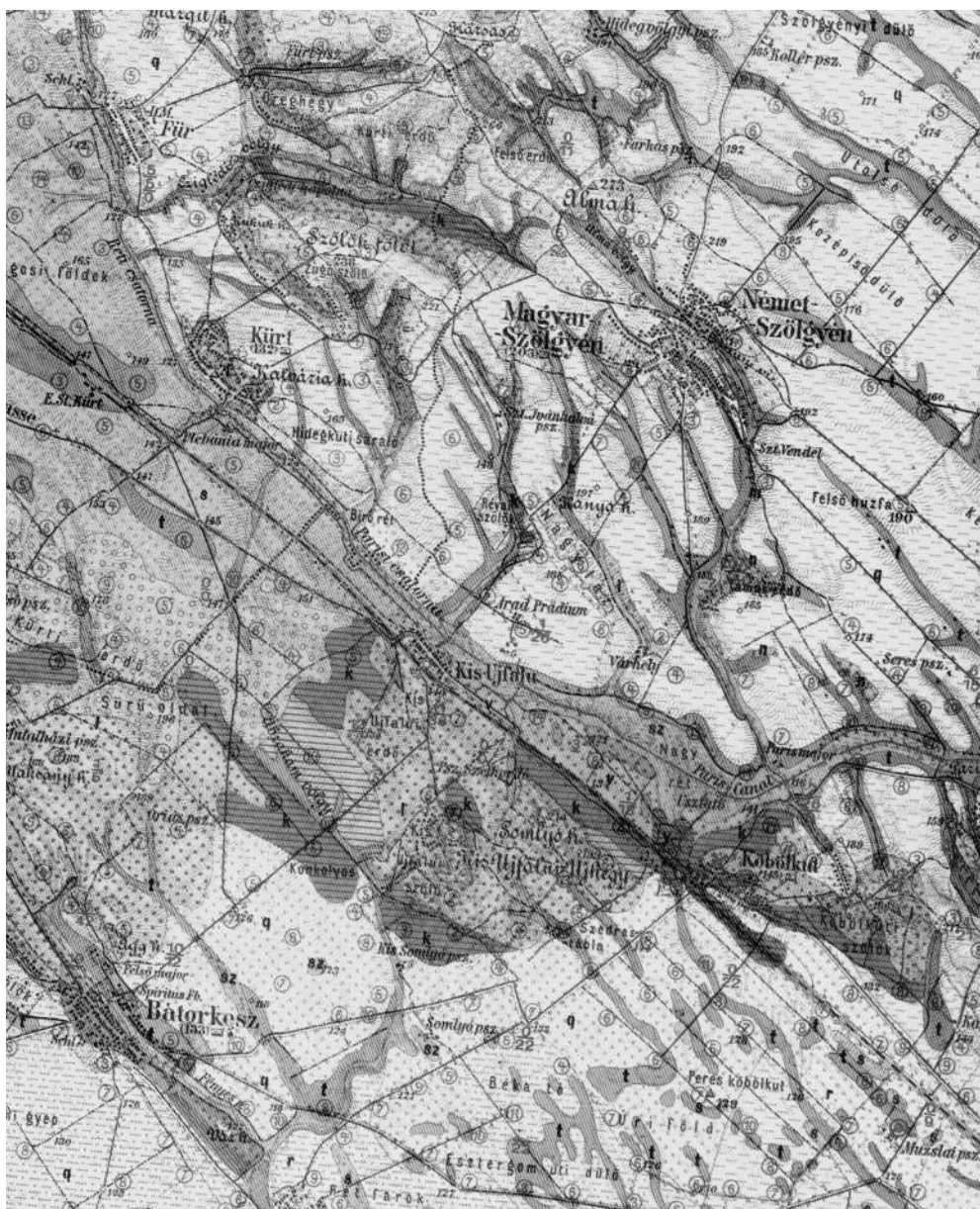
A környék földtani térképe
