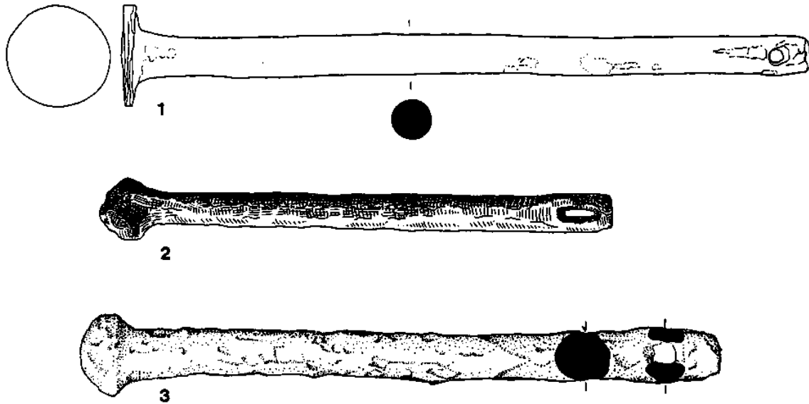
Abb. 165 Reibnägel: 1 Verna (I/64). - 2 Manching. - 3 Étival-Clairefontaine/La Pierre d'Appel. - M = ca. 1 : 2.
