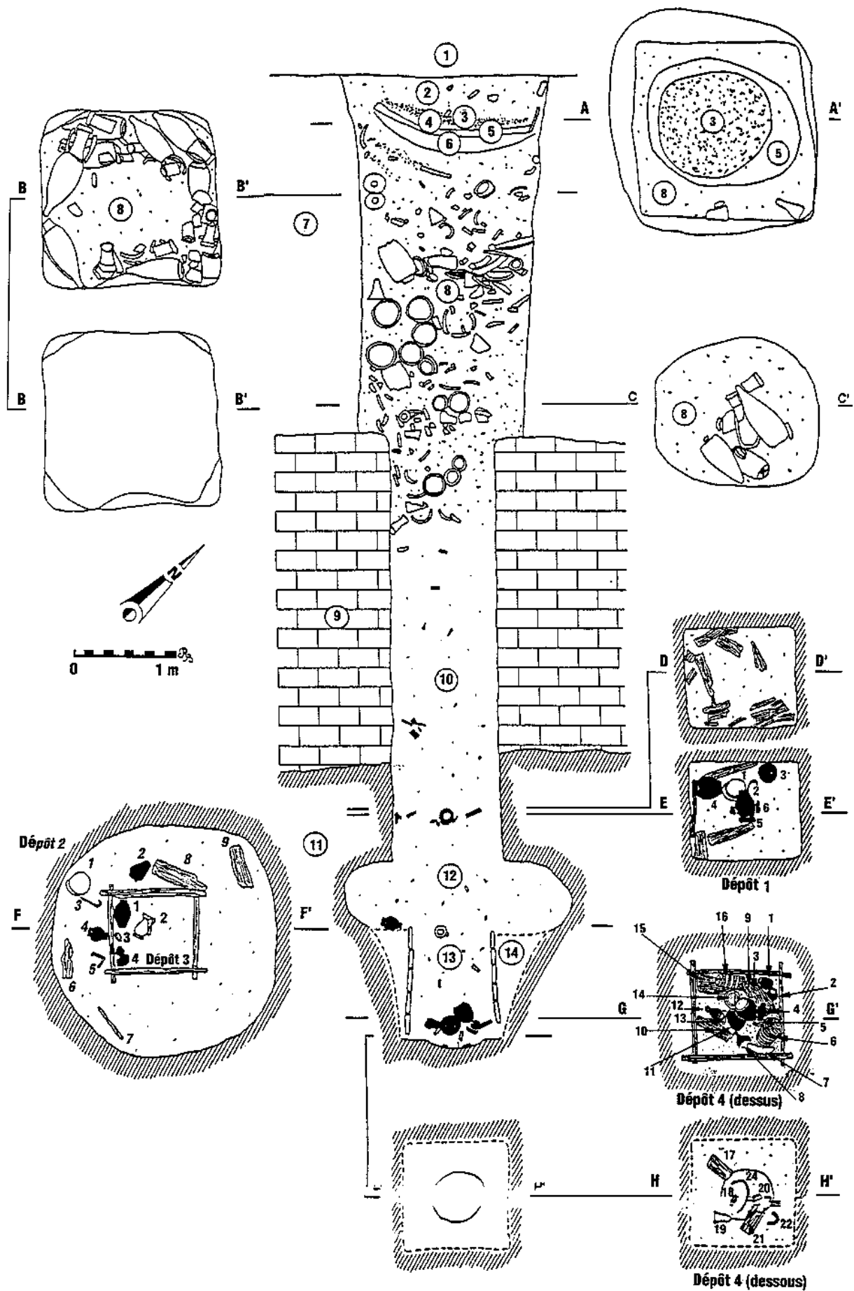
Abb. 231 Agen, L'Ermitage. Schacht st. 41 von 1993. (Zeichnung R. Boudet). - Nach Boudet, Rituels 82.
