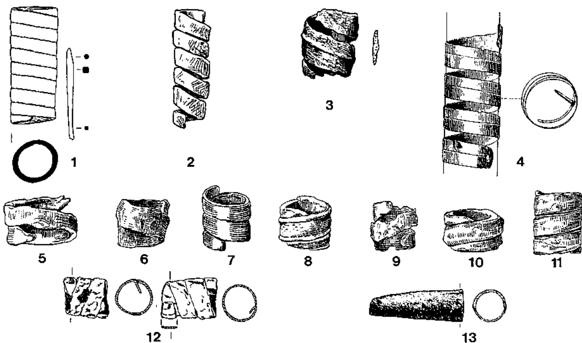
Abb. 206 Spiralen von Treibstacheln: 1 Estinnes (I/1). - 2 Armentières-sur-Ourcq (I/43). - 3 Kappel. - 4 Llyn Cerrig Bach. Spiralen unbekannter Verwendung: 5-11 Manching. - 12 Wederath Grab 391. Spitze: 13 Wederath Grab 1615 (I/38). - (Nachweis Anm. 838-839). - M = ca. 1 : 2.
