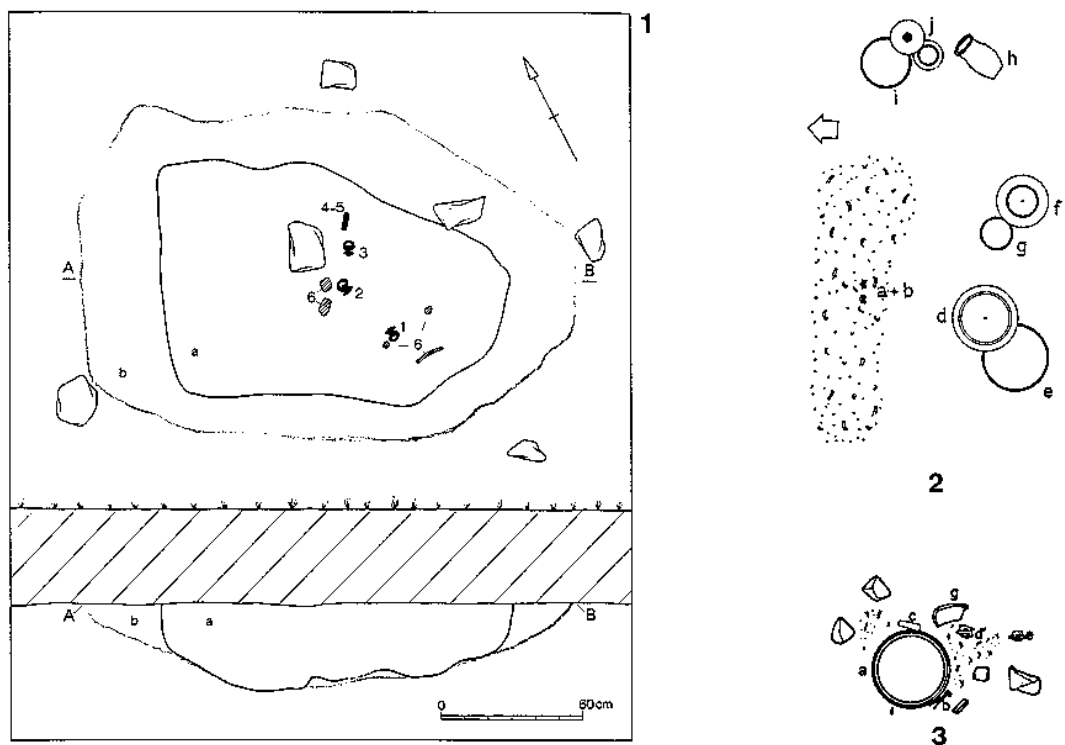
Abb. 225 Befundpläne: 1 Estinnes (I/1). - 2 Frohnhausen (I/13). - 3 Grab 1615 (I/38). - 2-3 M = ca. 1 : 20.
