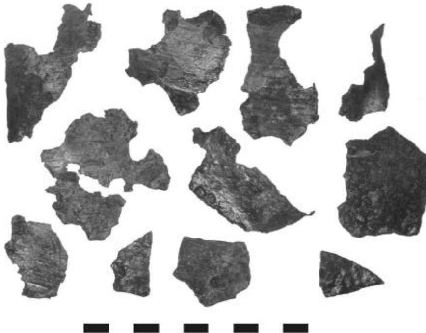
Abb. 49 Boé, Wagengrab. Bronzeblechfragmente (Auswahl) mit Treibspuren (Foto).
