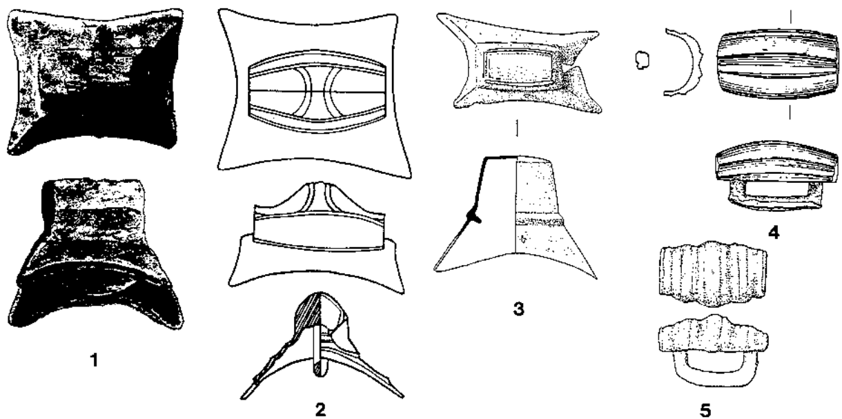
Abb. 191 Jochaufsätze der frühen Kaiserzeit: 1 Mont Beuvray/Bibracte (o. M.). - 2 Aulnay. - 3 Besançon. - 4 Kalkriese. - 5 Magdalensberg (Nachweise vgl. Anm. 765-769). - M = ca. 1 : 2.
