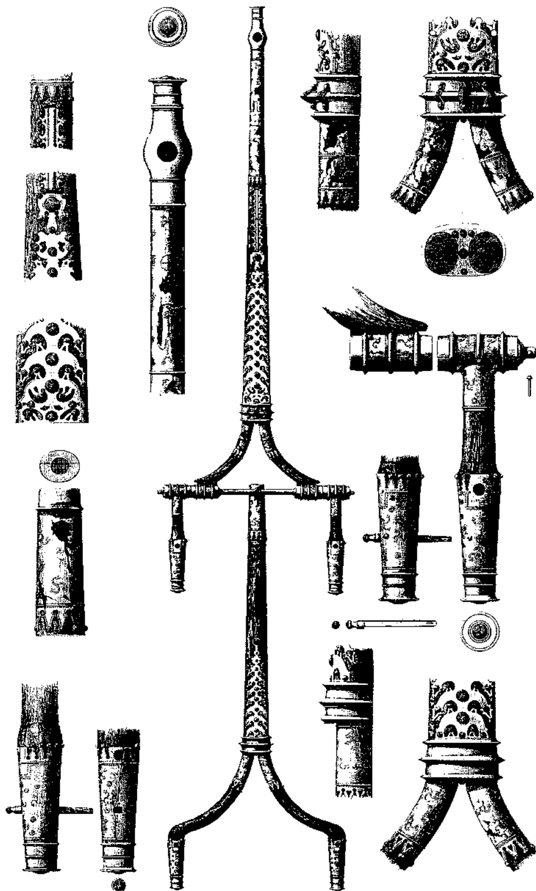
Abb. 88 Dejbjerg. Keltischer Wagen. Zugarmkonstruktion (nach Petersen, Vognfundene).
