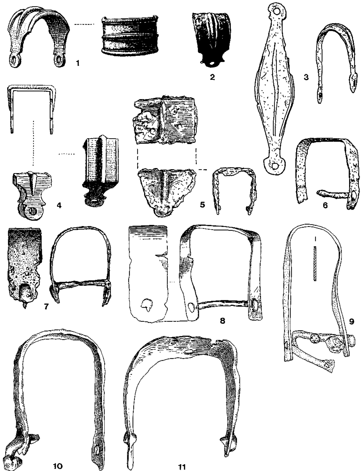
Abb. 126 Felgenklammern Typ Stradonice: 1 Dejbjerg. - 2 Stradonice. - 3 Amot. - Typ Husby: 4 Dejbjerg. - 5 Husby. - Bandförmige Felgenklammern: 6 Brzeźniak. - 7 Bern/Tiefenau. - 8 Numantia. - 9 Sanzeno. - 10-11 Manching. - (Nachweise vgl. Tab. 13). - M = ca. 1 : 2
