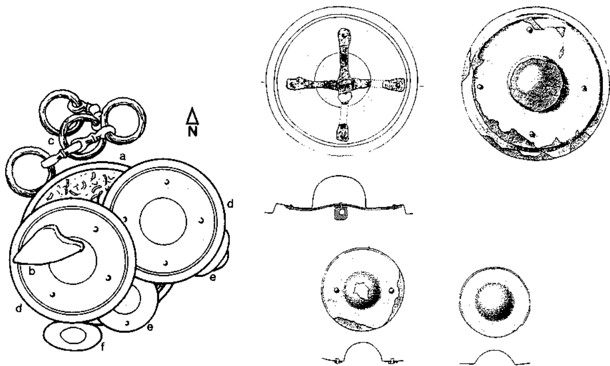
Abb. 196 Bronzephaleren mit Eisenbändern aus Wederath Grab 1445 (exemplarisch; nach Müller-Karpe). - Phaleren M = ca. 1 : 4; Befundplan M = ca. 1 : 5.
