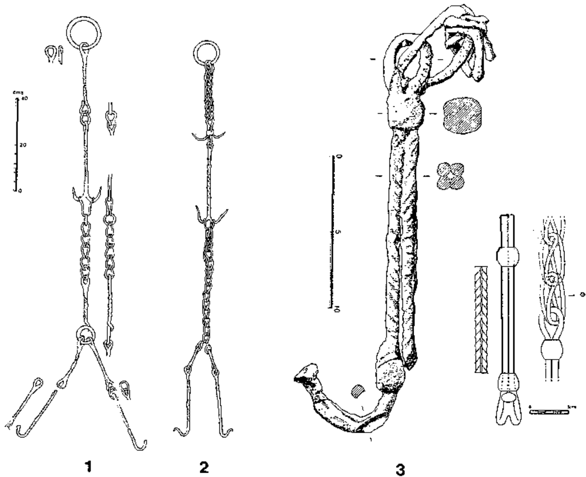
Abb. 47 Kesselgehänge aus England in Fuchsschwanztechnik: 1 Butley. - 2 'East Anglia' . - 3 Danebury (Nach Manning, Cauldron Chains 137 Abb. 3, 2-3; Cunliffe/Poole, Danebury /5 346 Abb. 7. 21).
