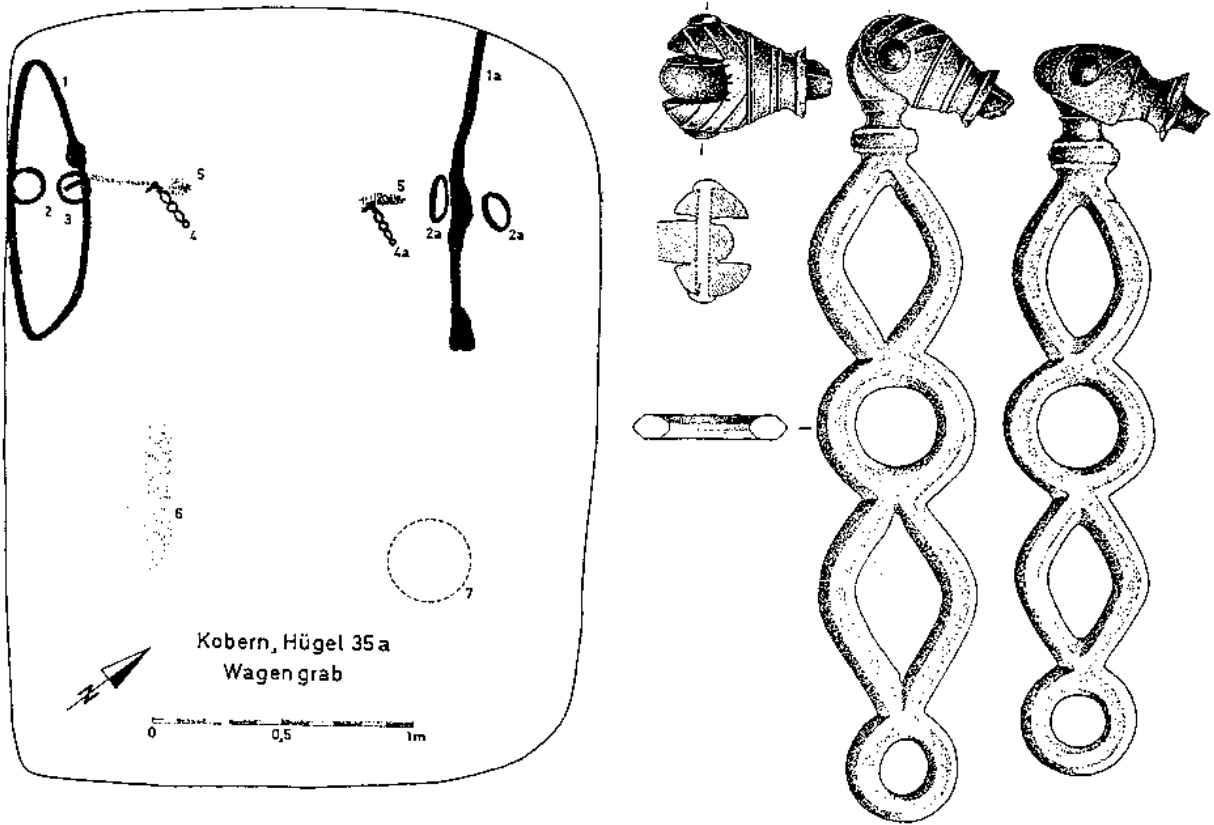
Abb. 151 Kobern/Chorsang Hügel 35a (Kr. Mayen-Koblenz, D). - (Nadeln) Ausgrabungen). - Doppelösenstifte M = ca. 1 : 2. - Befund M = ca. 1 : 30.
