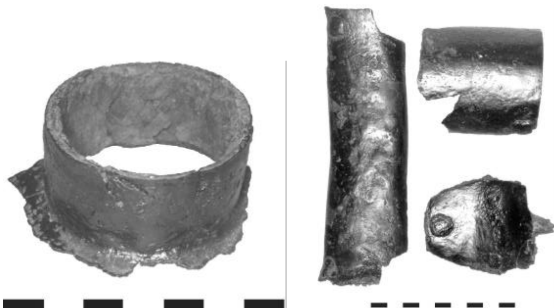
Abb. 99/100 Boé, Wagengrab. Ring vom Deichselscharnier. - Gewölbte Eisenbleche mit Nagelungen (Foto).
