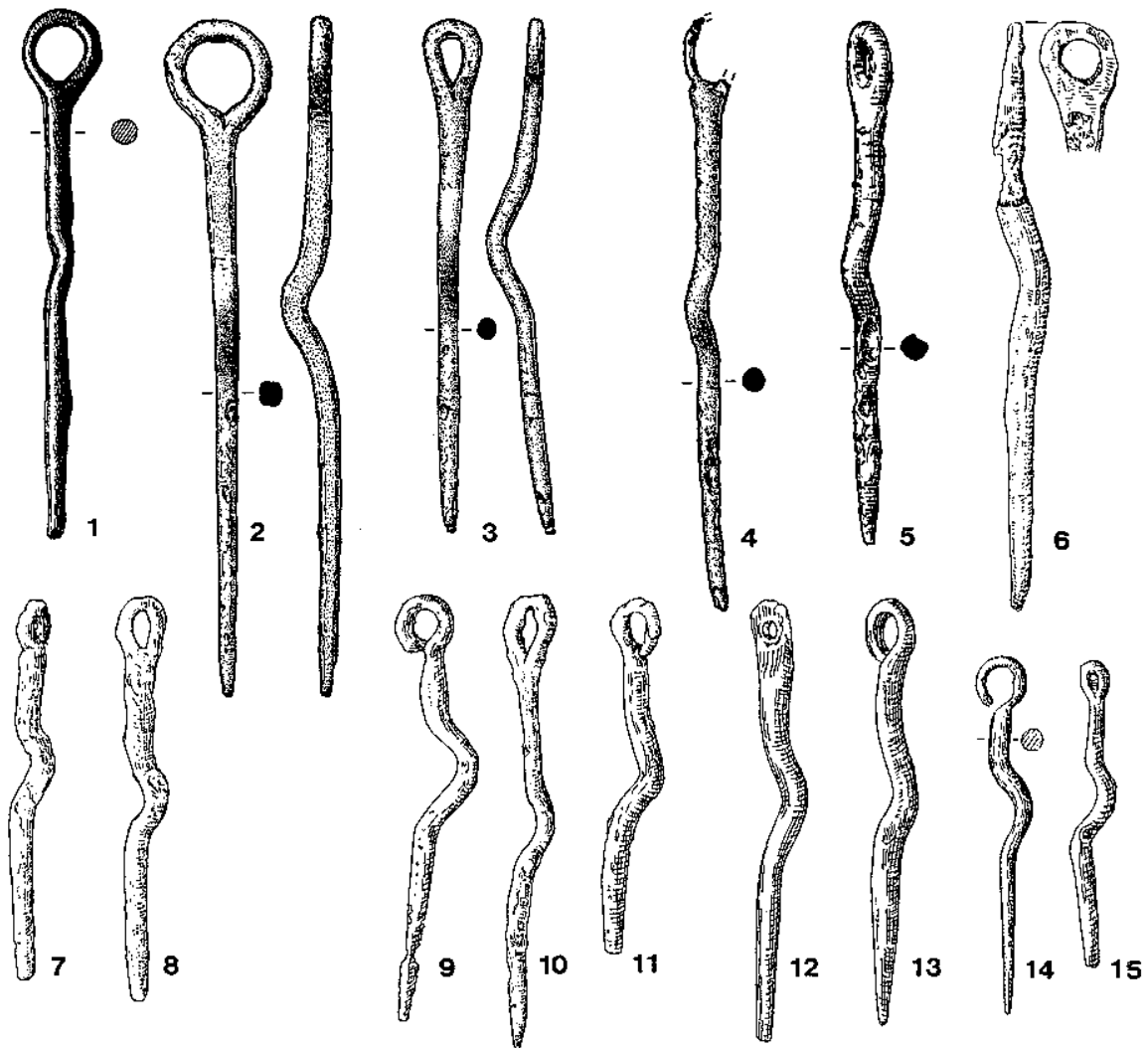
Abb. 160 Gekröpfte Ösenstifte (Eisen): 1 Enkirch (I/12). - 2-5 Bern/Tiefenau. - 6-15 Manching. - M = ca. 1 : 2.
