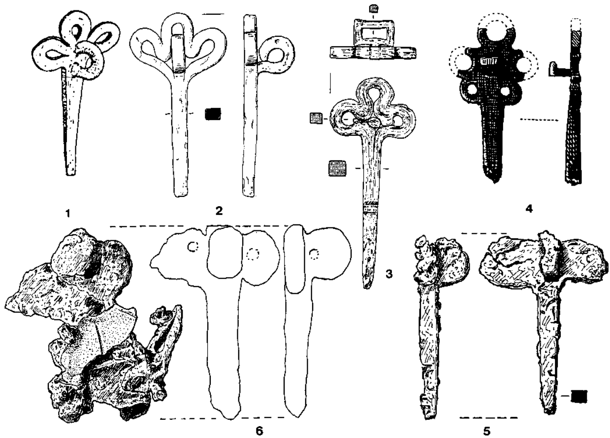
Abb. 141 Achsnägel mit mehrfachem Schlaufenkopf und geradem Stift: 1 Brzeźniak (I/73, ohne Maßstab). - 2 Graitschen b. Bürgel/Alter Gleisberg. - 3 Karlstein. - 4 Dejbjerg. - 5-6 Husby (I/25). - (Nachweise vgl. Tab. 20). - M = ca. 1 : 2.
