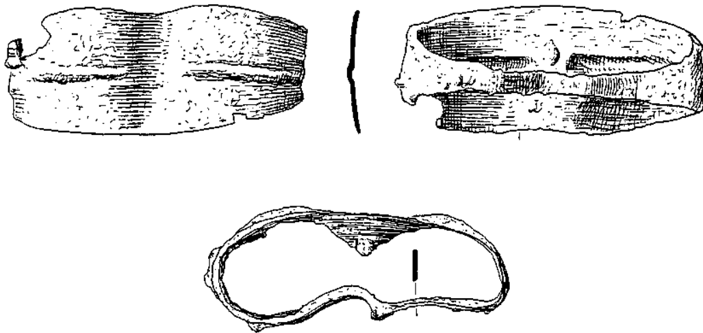
Abb. 164 Deichsel- oder Langfuhrmanschette aus Husby (I/25). - M = ca. 1 : 2.
