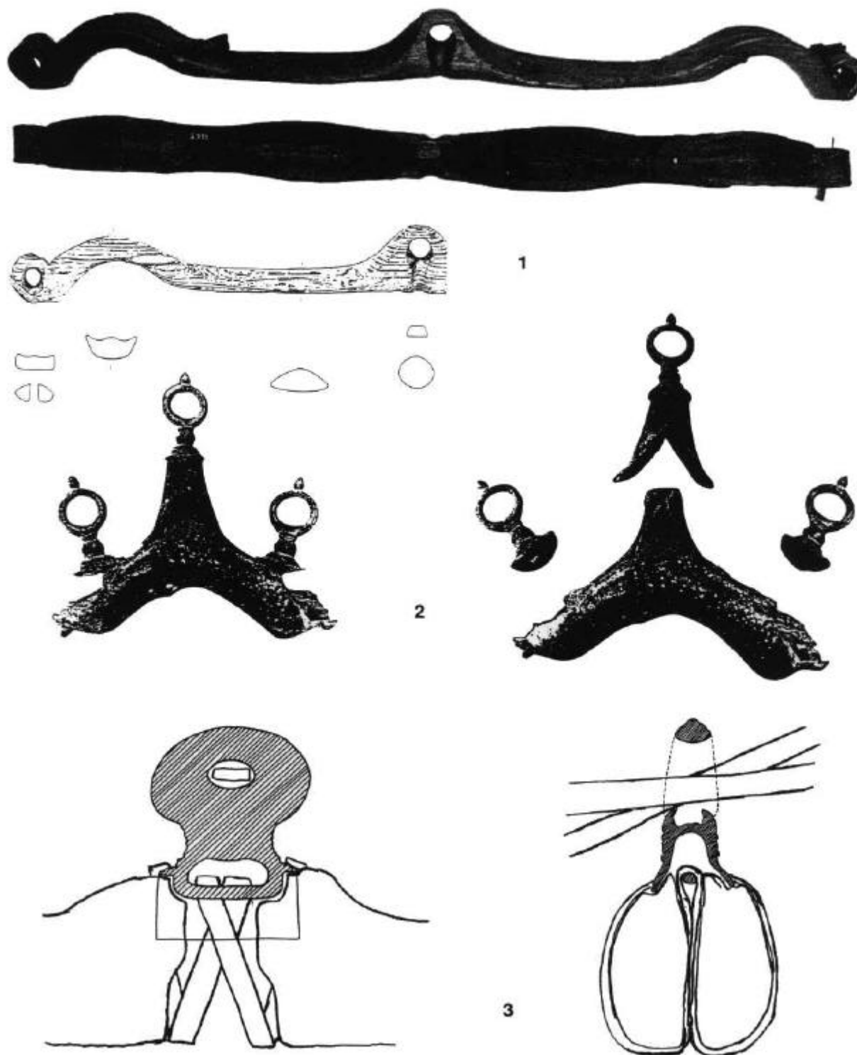
Abb. 172 1 Holzjoch aus Lundgaardshede/Bredmose (DK) (a M = ca. 1 : 7,5; b M = ca. 1 : 8; Nachweis vgl. Tab. 30). - 2 Zsámbék (Kom. Pest, H) (Nach Alföldi/Radnóti, Zügelringe). - 3 Versuch einer Darstellung der Befestigung und Riemenführung bei einem latènezeitlichen Führungsring.
