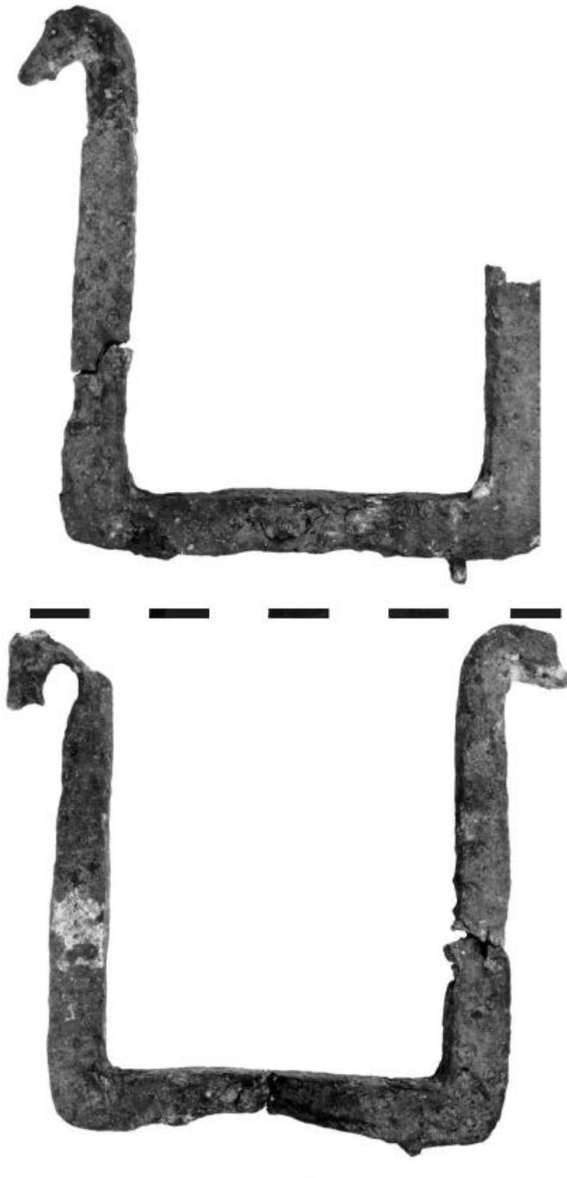
Abb. 50 Boé, Wagenrab. Feuerböcke (Foto: V. Iserhardt, RGZM; Einheit des Maßstabes 20 cm).
