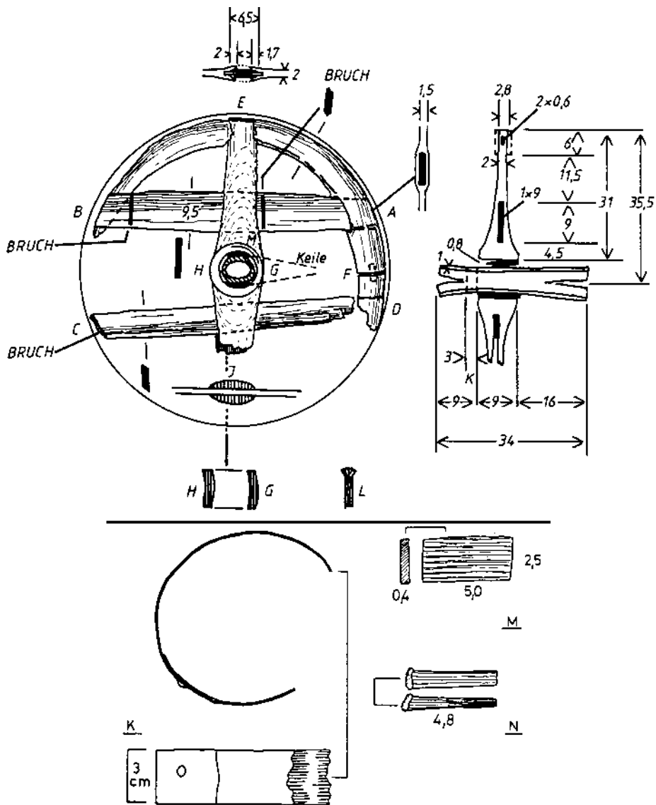
Abb. 128 Strebenrad aus Olympia (nach Hayen, Holz).
