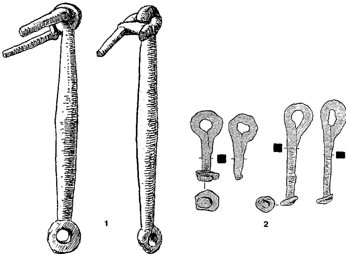
Abb. 152 1 Doppelösenstifte aus Armsheim (Kr. Mainz-Bingen, D). - 2 Ösenstifte aus Prunay (Dép. Marne, F). - M = ca. 1 : 2.
