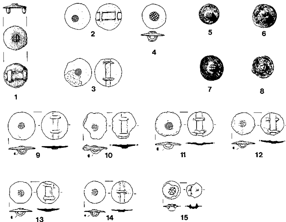
Abb. 203 Ösenskeiben mit Email: 1 Manching. - 2-4 Magdalensberg. - 5-8 Stradonice/Hradiště. - 9 Ljubljana, Gornji trg 30. - 10 Dunaj/Gradišče. - 11 Novo mesto/Okrajno glavarstvo. - 12 Mihovo/Trnišča. - 13 Pečovnik/Vipota. - 14 Vir pri Šteti/Cvinger. - 15 Celje. - (Nachweise vgl. Tab. 45). - M = ca. 1 : 2.
