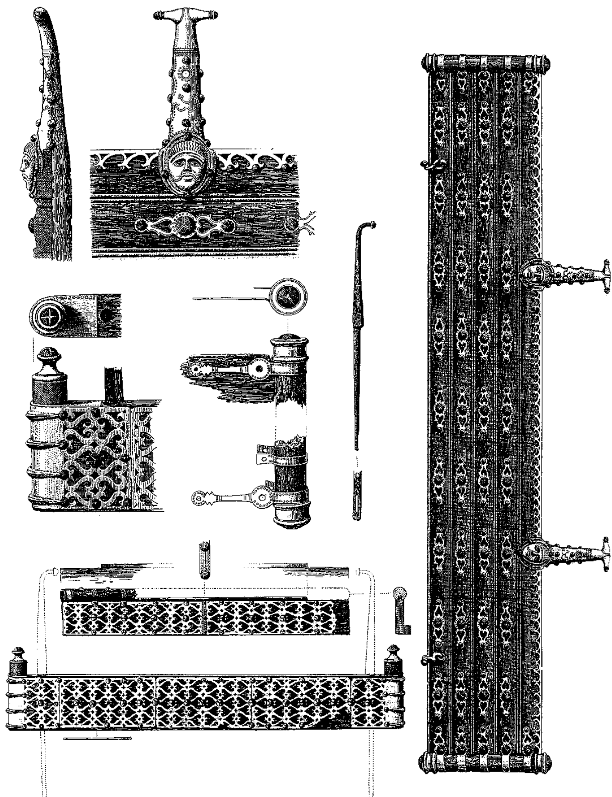
Abb. 87 Dejbjerg. Keltischer Wagen. Reste des Wagenkastens. - (Nach Petrusen fundene).
