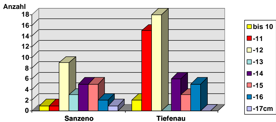
Abb. 130 Diagramm der Durchmesserverteilung bei Naberringen aus Sanzeno (nach Nothdurfter, Eisenfunde) und Bern/Tiefenau (nach Müller, Massenfund).
