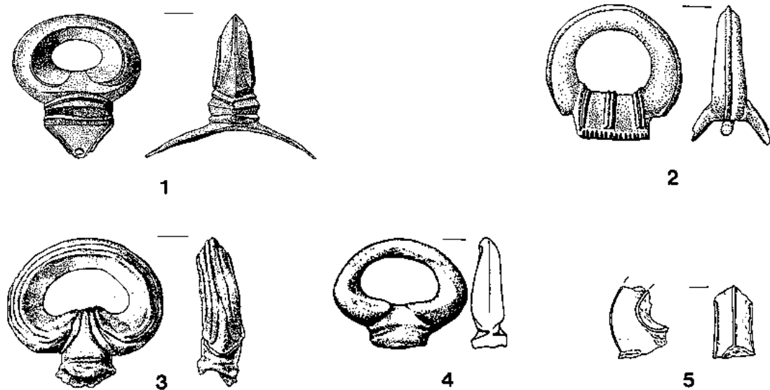
Abb. 179 Führungsringe Sondertypen und Typ Estinnes/Kappel/Grabenstetten: 1-2 Manching. 3 Biebertal-Fellingshausen/Dünsberg. - 4 Dambron/La Fosse Dieppe. - 5 Römhild/Steinsburg. - (Nachweise vgl. Tab. 36). - M = ca. 1 : 2.
