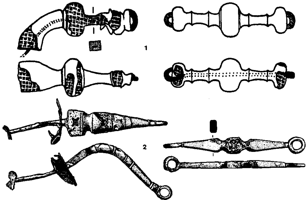
Abb. 156 Ösenknäufe und Doppelösenstift (Eisen und Bronze): 1 Tremblois-les-Rocrois/1939 (I/63). - 2 Bern/Tiefenau (nach Müller, Massenfund). - M = ca. 1 : 2.
