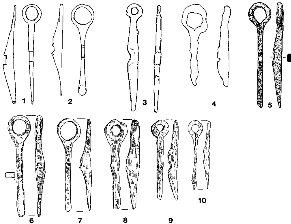
Abb. 158 Ösenstifte mit Einkerbung (Eisen): 1-2 Brežice Grab 6 (I/78). - 3 Brežice Grab 55 (I/79). - 4 Nanterre (I/57). - 5 Bern/Tiefenau. - 6-10 Manching. - (Nachweis Anm. 641). - M = ca. 1 : 2.
