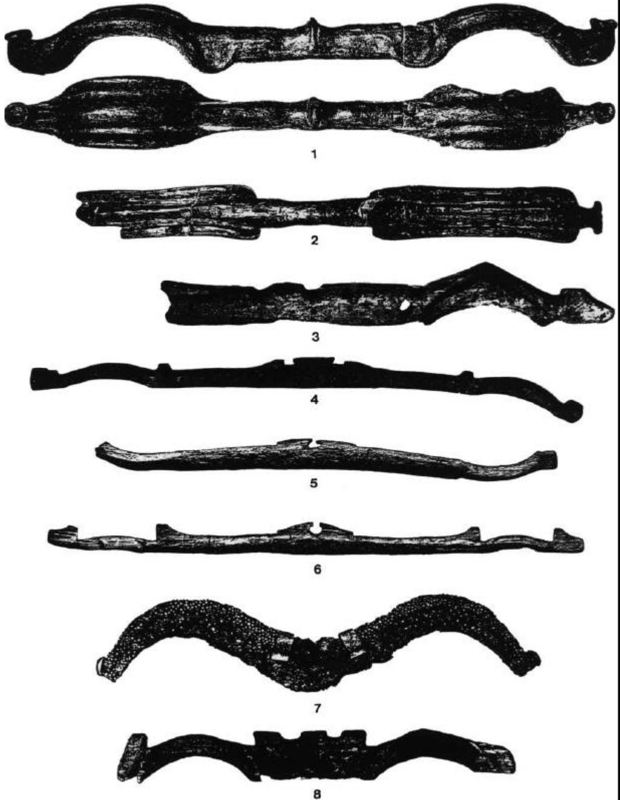
Abb. 171 Holzjoche: 1 La Tène (M = ca. 1 : 7). - 2 La Tène (M = ca. 1 : 6). - 3 Unterlübbe (M = ca. 1 : 6). - 4 Ezinge (L. 1,28m). - 5 Finderup (L. 1,40 m). - 6 Dejbjerg (L. 1, 80 m). - 7 Kelheim (L. 0,94 m). - 8 Annaberg (L. 0,93 m). - (Nachweise siehe Tab. 30).
