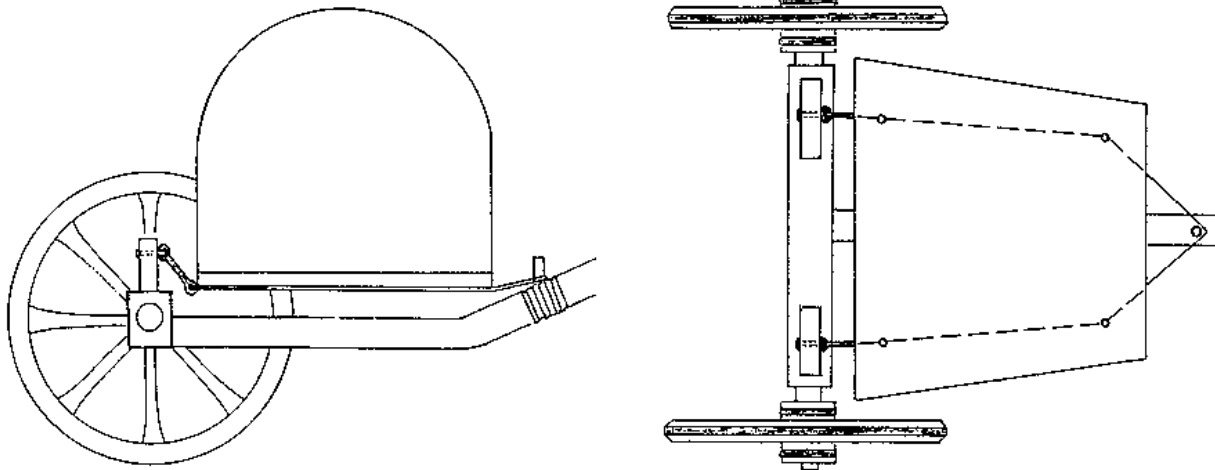
Abb. 209 Rekonstruktion des zweirädrigen Wagens mit Doppelösenstiften der Stufe Lt A von Grosbous-Vichten (L). - Nach Metzler, Gräberfeld.
