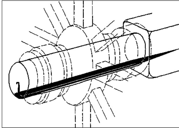
Abb. 136 Schematischer Rekonstruktionsvorschlag. Der Achsschenkelbeschlag ist in den Achsschenkel eingelassen. Seine Spitze steckt im Achsblock, während das andere, hakenförmige Ende am Kopf des Achsschenkels befestigt ist. - (Nach Müller, Massenfund 55 Abb. 26).
