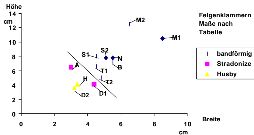
Abb. 127 Diagramm: Größe und Breite von Felgenklammern der jüngeren Latènezeit. (Nachweise vgl. Tab. 13).
