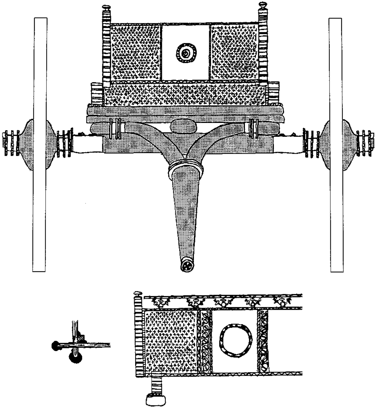
Abb. 120 Boé, Wagengrab. Versuch einer Rekonstruktionszeichnung der Vorderansicht des Wagens und der Seitenansicht des Wagenkastens. - M = ca. 1 : 10.
