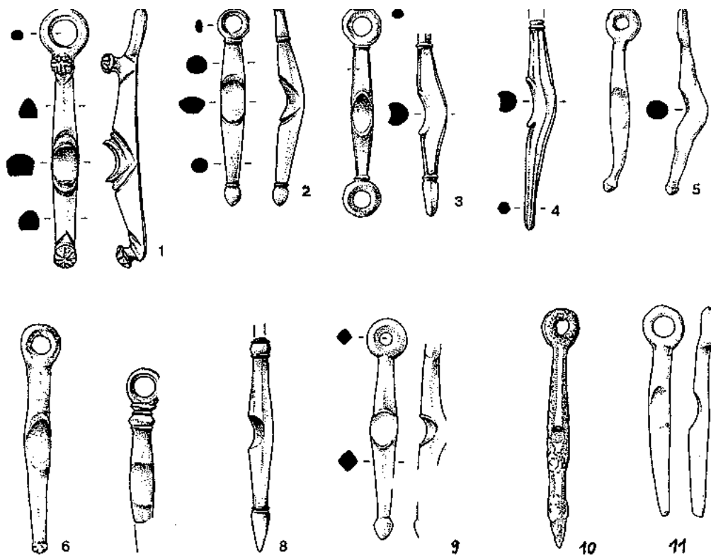
Abb. 159 Ösenstifte mit Einkerbung (Bronze): 1 Ptuj. - 2 Mihovo. - 3-4 Gracarca. - 5 Bern/Engelhalbinsel. - 6-9. Stradonice. - 10 Staré Hradisko. - 11 Wederath Grab 1726 (II/13). - (Nachweis Anm. 642). - M = ca. 1 : 2.
