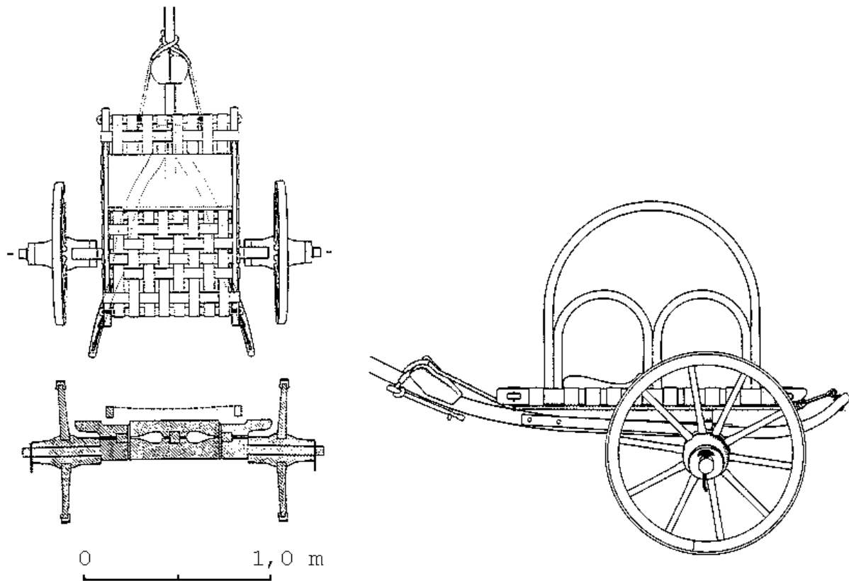
Abb. 210 Rekonstruktion eines zweirädrigen Wagens durch A. Furger Gunti unter Verwendung von Teilen aus La Tène (Kt. Neuchâtel, CH). - (Nach Furger-Gunti, Streitwagen).
