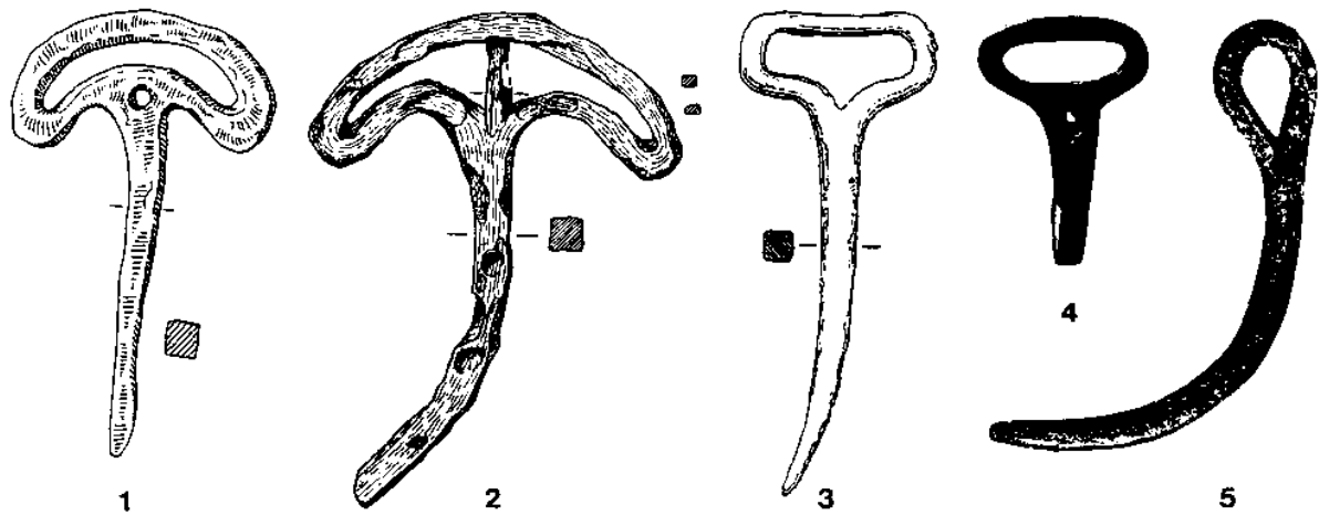
Abb. 142 Achsnägel mit einfachem Schlaufenkopf: 1 Manching. - 2 Basel-Gasfabrik. - 3 Numantia. - 4 Stradonice/Hradčt. - 5 La Tène. - (Nachweise vgl. Tab. 22). - M = ca. 1 : 2.
