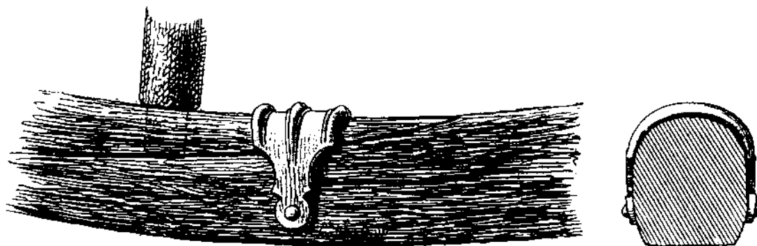
Abb. 125 Felgenklammer aus Dejbjerg . - (Nach Petersen, Vognfundene). - M = ca. 1 : 2.
