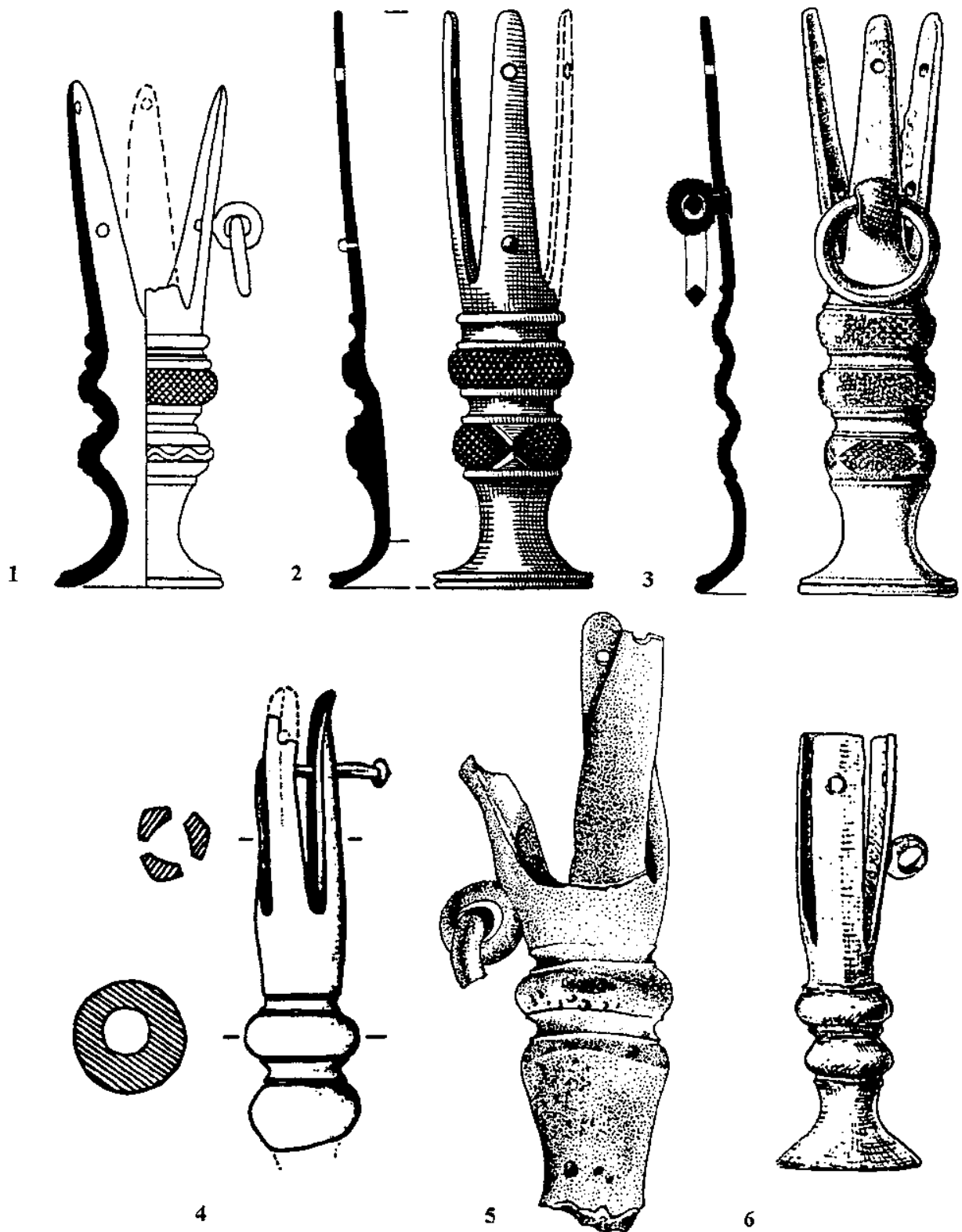
Abb. 64 Trinkhornendbeschläge: 1 Andernach (nach Bockius, Untersuchungen Taf. 26, 2). - 2 Schkopau Grab 5 (nach Schmidt/Nitzschke, Gräberfeld 103 Taf. 3 h). - 3 Vinji vrh (nach Božič, Kritisches 423 Abb. 1). - 4 Weingarten (nach Engels, Waffengräber 186 Abb. 3, 5). - 5 Mehrhoog Grab 4 (nach Janssen, Brandgräber Abb. 6). - 6 Kossebau (nach Hoffmann, Trinkhornbeschläge 36 Abb. 1 g). - M = ca. 1 : 1.
