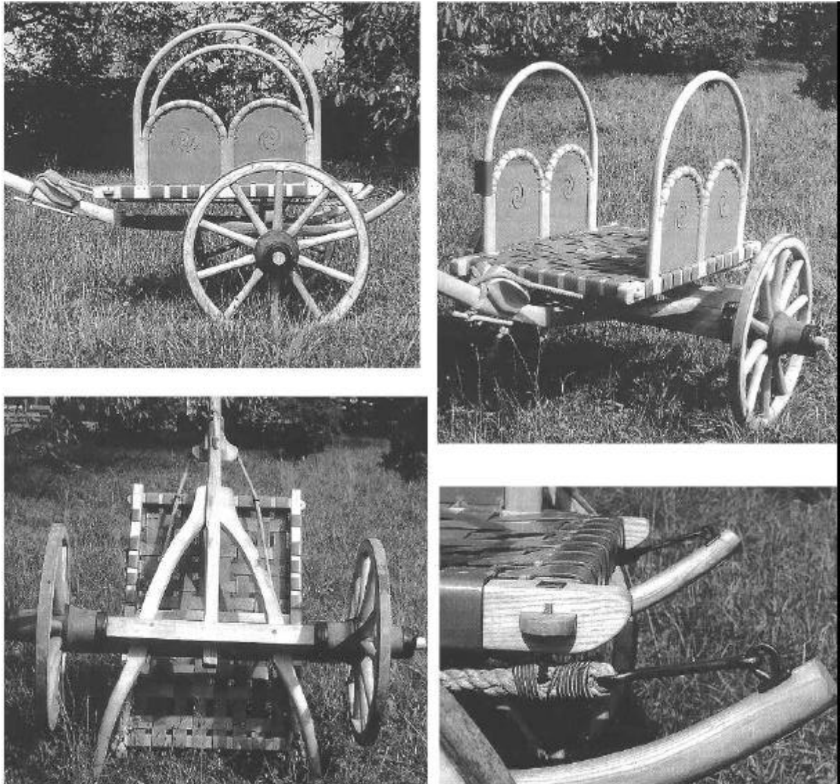
Abb. 211 Detailfotos der Rekonstruktion. - Nach Furger-Gunti, Streitwagen.
