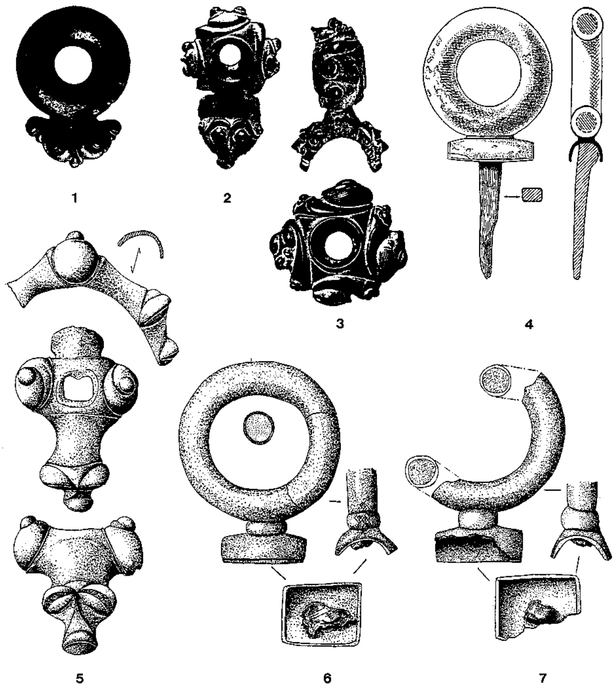
Abb. 174 Führungsringe: 1 Mezek (I/5). - 2-3 Paris (I/58). - 4 Leval-Trahegnies (I/2). - 5-7 Attichy (I/44). - M = ca. 1 : 2.
