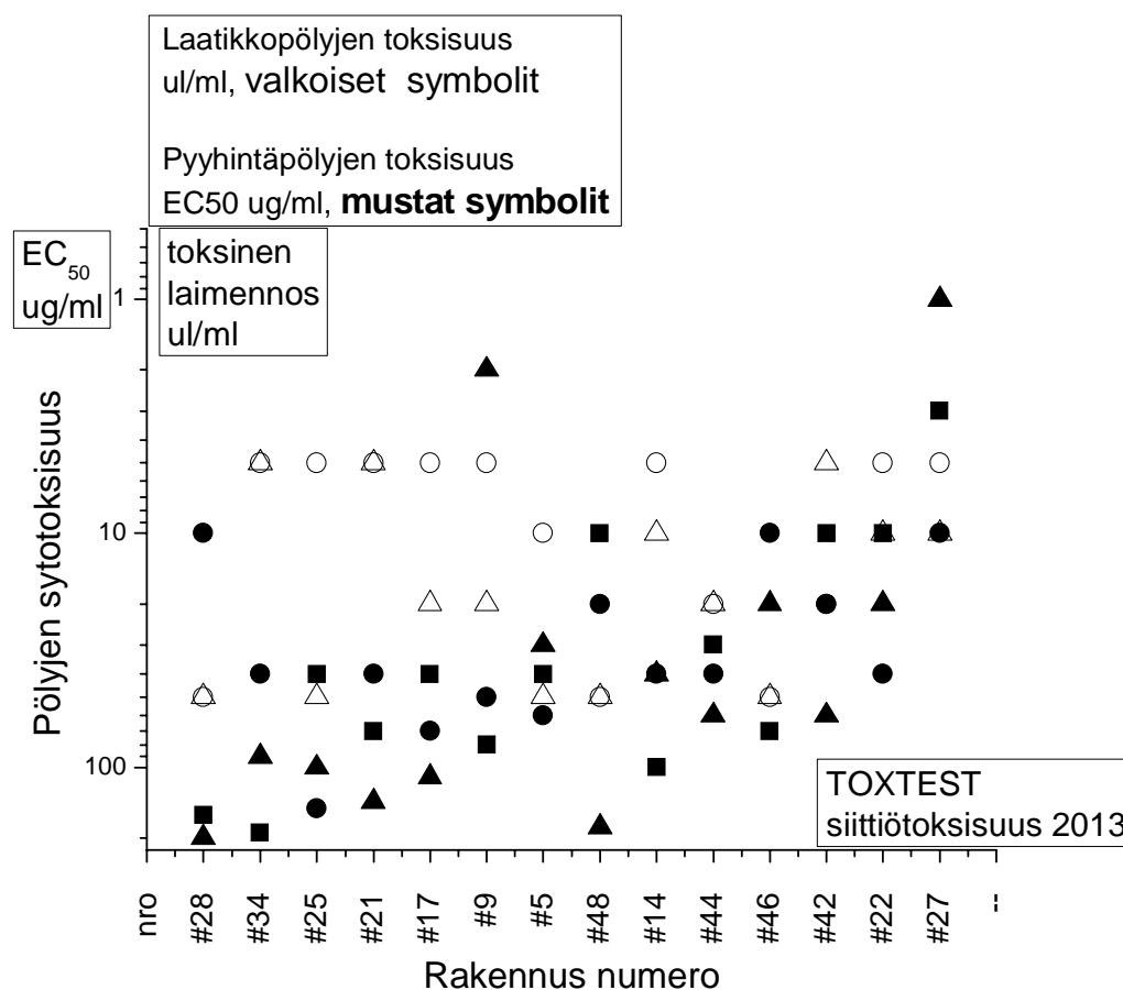
Kuva 4-11. Keräyslaatikkopölyn toksisuuden mittaaminen asunnoista (TOXTEST). Kuvassa mustat symbolit ovat niiden 14:n asuinrakennuksen keräyslaatikkopölyjen uutteen, joiden pyyhkäisy-pölyjen toksisuudet on näytetty siittiöille kuvassa 1-11, ja valobakteerille kuvassa 2-12. Keräyslaatikkopölyille (valkoiset symbolit) ei voitu laskea EC50 arvoja (ominaismyrkyllisyyttä, vasemmanpuolinen Y-akseli) koska punnitustietoja ei ollut. Tulokset on kuvassa näytetty tilavuusmittana: kuinka monta mikrolitraa kyseistä pölyuutetta voi laittaa per ml siittiösuspensiota. (oikeanpuolinen Y-akseli).
