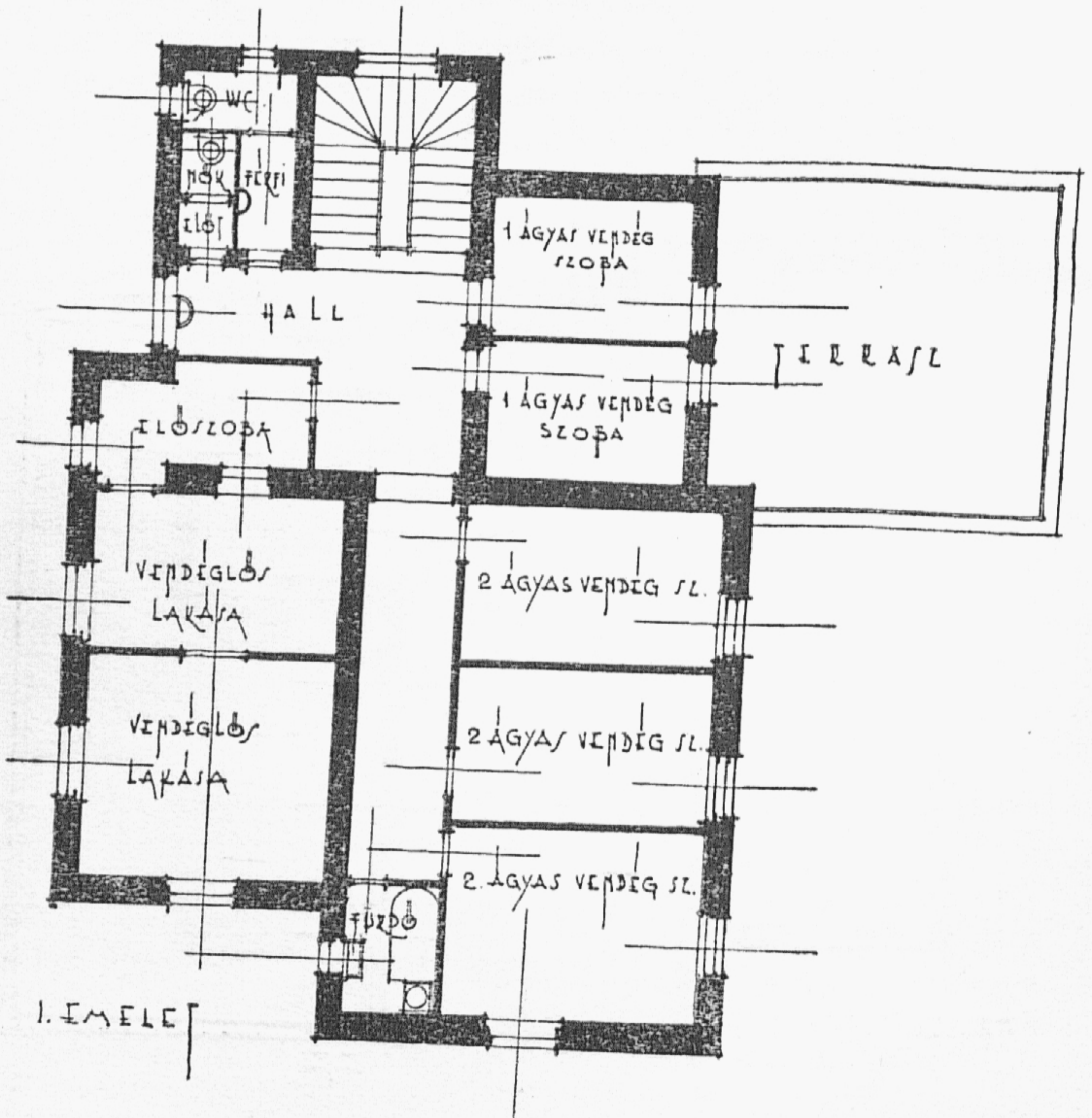
I. és II. emeleti alaprajz.
