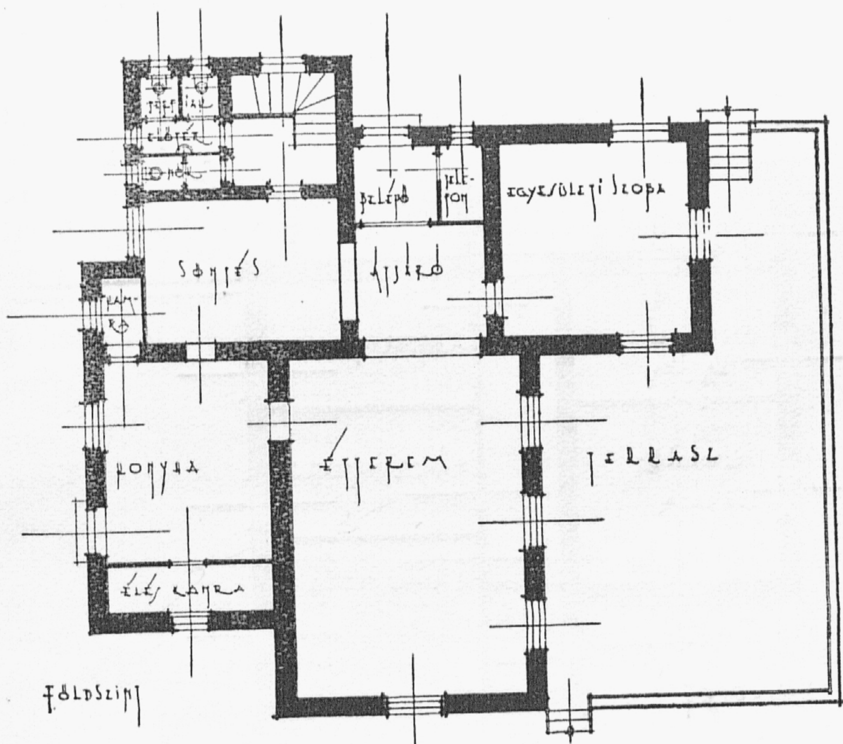
Menedékházunk földszinti alaprajza.
