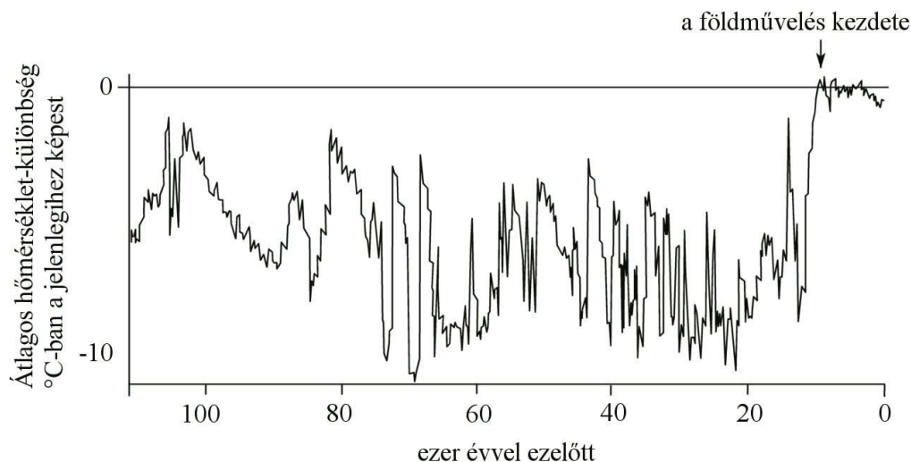
6. ábra. Az elmúlt 110 ezer év hőmérsékletváltozásai, jégminták alapján rekonstruálva Dansgaard ábrája Czelnai (1999) A világóceán c. könyvéből
