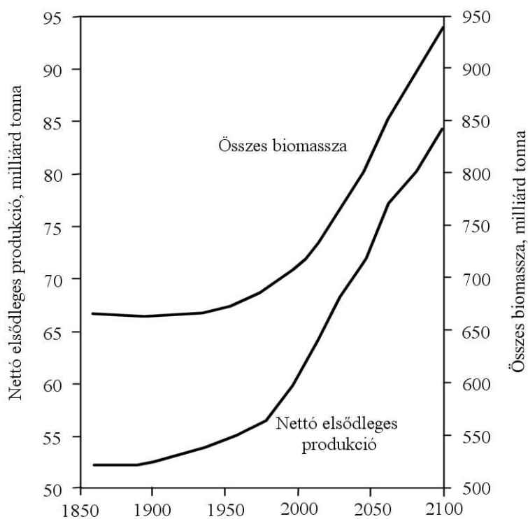
17. ábra. A biomassa és a nettó elsődleges produkció szimulált növekedése a \text{CO}_2 -koncentráció és a hőmérséklet emelkedésének hatására, 1850–2100 között. Forrás: Cramer et al. 2000, White et al. 1999
