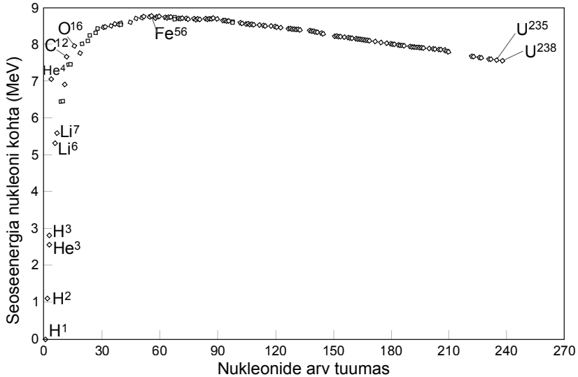
Joonis 1. Keskmine seoseenergia nukleoni kohta sõltuvalt nukleonide arvust tuumas. Allikas: Wikimedia Commons [2].
