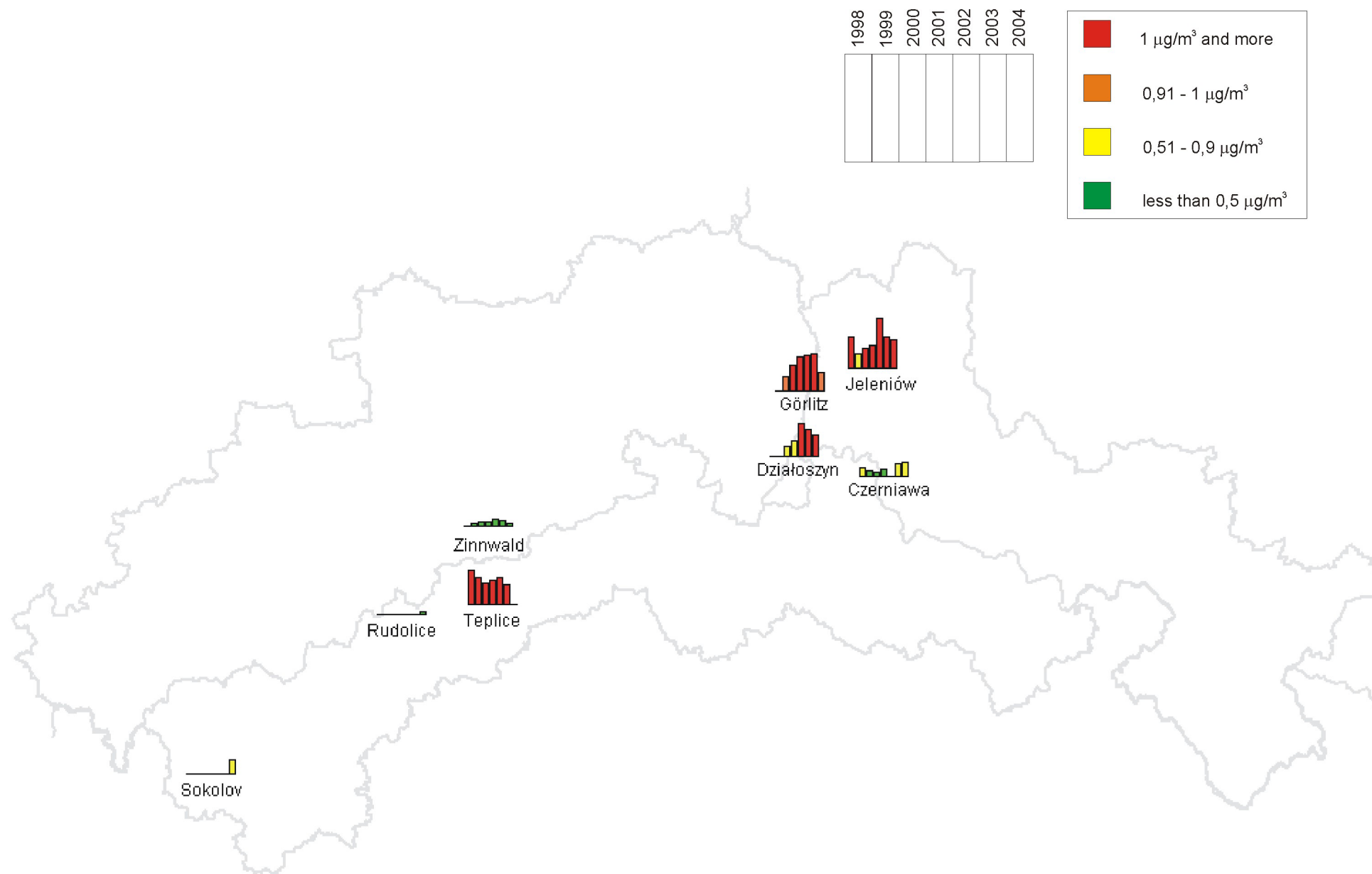
Rysunek 15. Średnioroczne wartości stężeń BaP w Pm 10 w trójgranicznym regionie (1998 - 2004)
