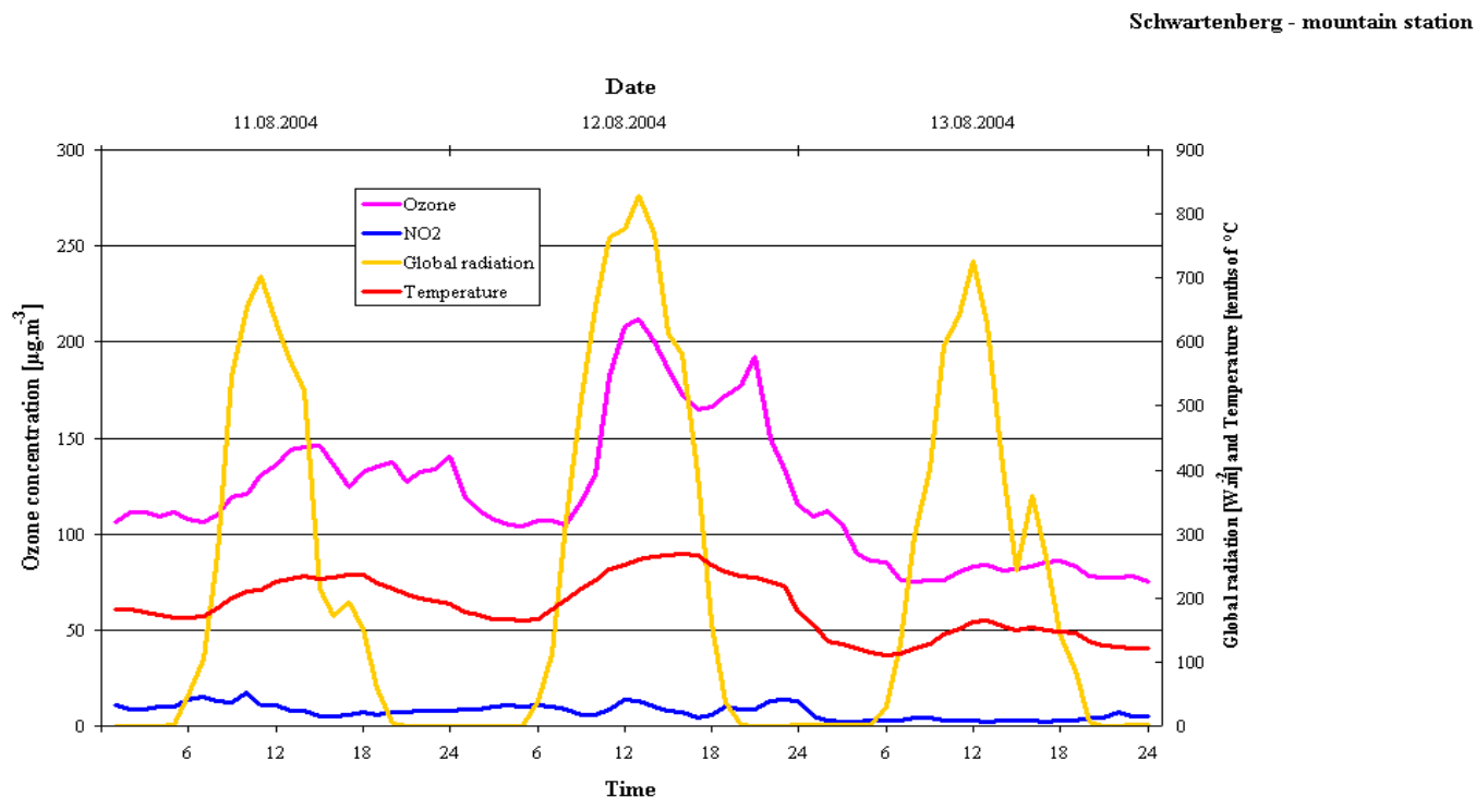
Figure 19. Summer episode: Schwartenberg - mountain station (DE) Obrázek 19. Letní epizoda: Schwartenberg, horská stanice (DE) Abbildung 19. Sommerepisode für die Bergstation Schwartenberg (DE) Rysunek 19. Epizod letni: Schwartenberg - stacja góraska (DE)
