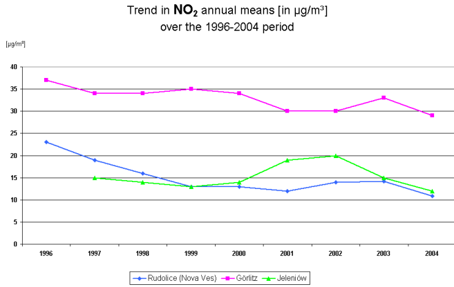
Figure 4. Changes in annual mean concentrations (1996–2004) Obrázek 4. Změny ročních průměrných koncentrací (období 1996–2004) Abbildung 4. Die Entwicklung der Jahresmittelwerte (1996 bis 2004) Rysunek 4. Zmiany stężeń średniorocznych (okres 1996–2004)
