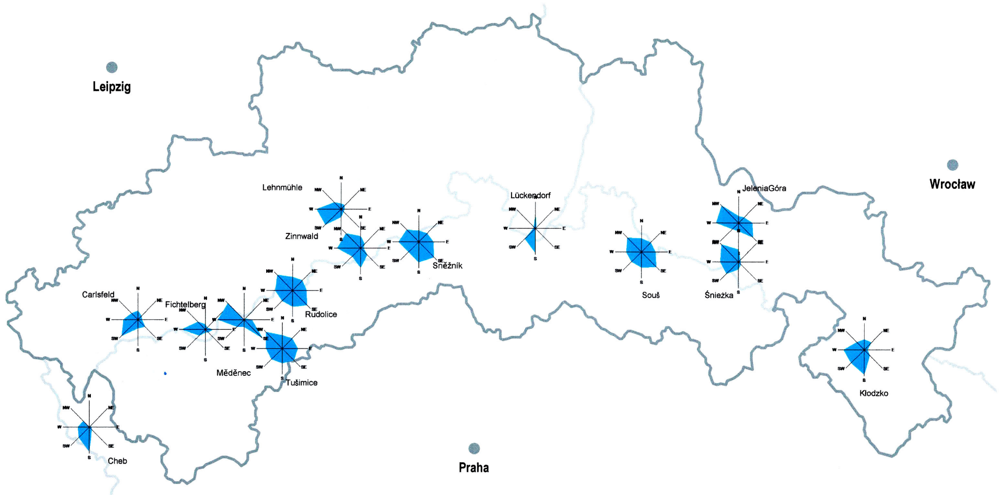
12 Figure 2. Frequency of wind directions in the Tri-border region, 2004 Obrázek 2. Četnost směru větru v příhraniční oblasti v roce, 2004 Abbildung 2. Windrichtungsverteilung im Dreiländereck, 2004 Rysunek 2. Częstości kierunków wiatru w trójgranicznym regionie, 2004
