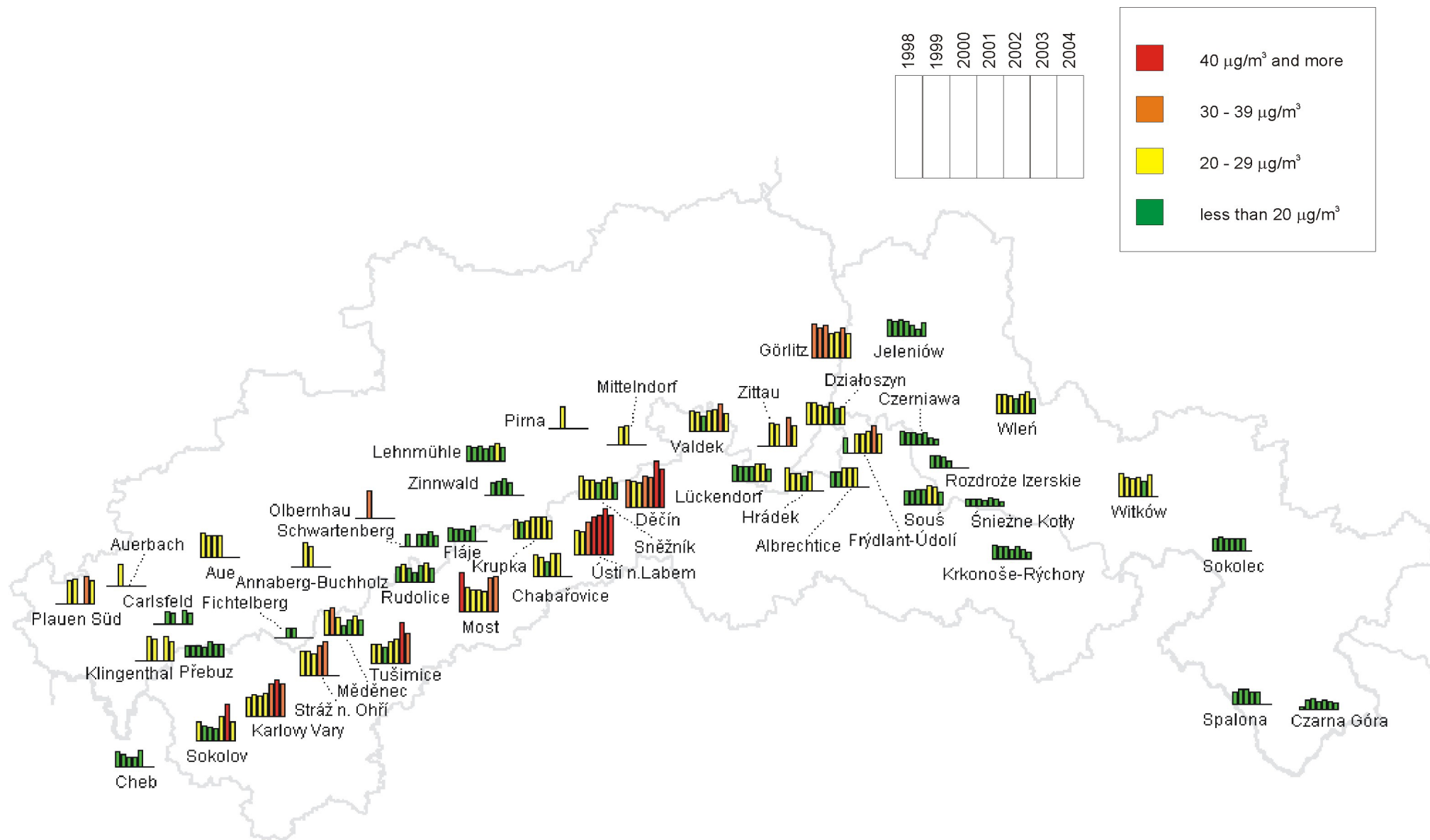
Figure 13. Annual mean values of suspended particulate matter PM 10 in the Tri-border Region (1998 - 2004) Obrázek 13. Roční průměrné hodnoty prašného aerosolu PM 10 v příhraniční oblasti (1998 - 2004) Abbildung 13. PM 10 -Schwebstaub-Jahresmittelwerte im Dreiländereck (1998 - 2004) Rysunek 13. Średnioroczne wartości stężeń pyłu zawieszonego PM 10 w trójgranicznym regionie (1998 - 2004)
