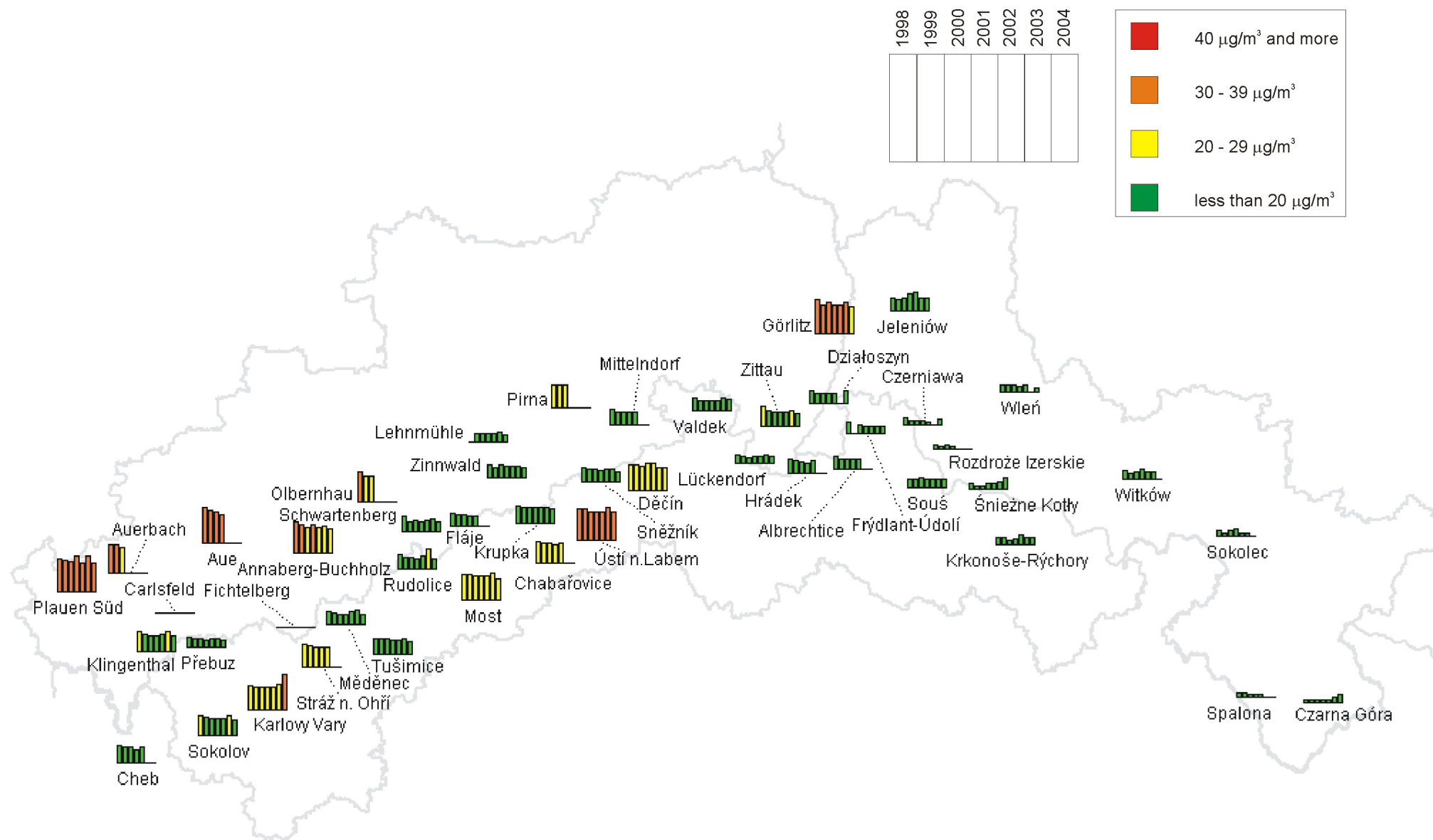
Figure 12. Annual mean values of nitrogen dioxide in the Tri-border Region (1998 - 2004) Obrázek 12. Roční průměrné hodnoty oxidu dusičitého v příhraniční oblasti (1998 - 2004) Abbildung 12. Stickstoffdioxid-Jahresmittelwerte im Dreiländereck (1998 - 2004) Rysunek 12. Średnioroczne wartości stężeń dwutlenku azotu w trójgranicznym regionie (1998 - 2004)
