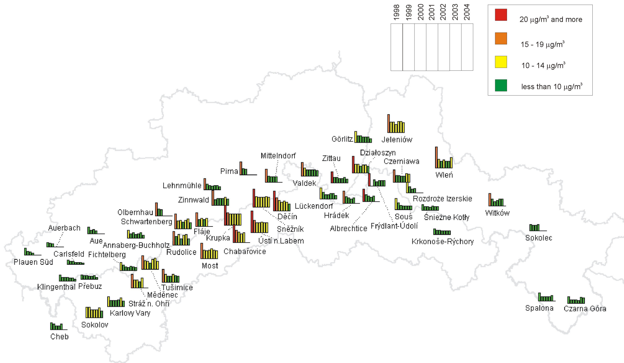
Figure 11. Annual mean values of sulphur dioxide in the Tri-border Region (1998 - 2004) Obrázek 11. Roční průměrné hodnoty oxidu siřičitého v příhraniční oblasti (1998 - 2004) Abbildung 11. Schwefeldioxid-Jahresmittelwerte im Dreiländereck (1998 - 2004) Rysunek 11. Średnioroczne wartości stężeń dwutlenku siarki w trójgranicznym regionie (1998 - 2004)
