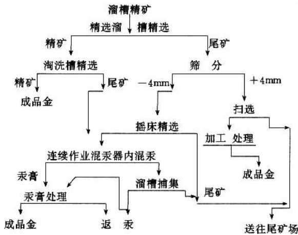
图 4-5-1 溜槽精矿的精选流程
