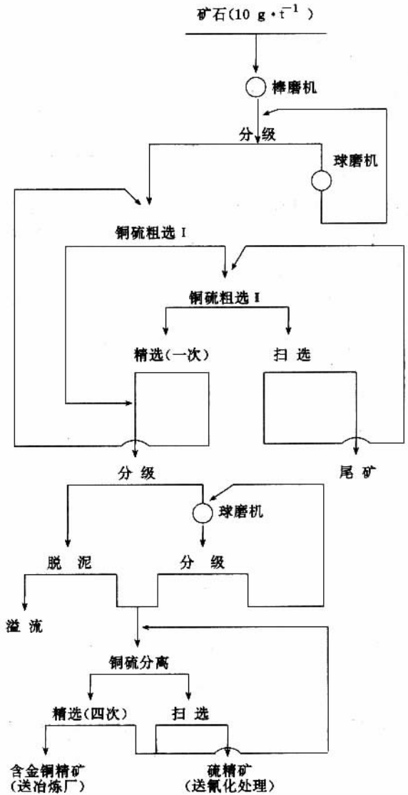
图 4-6-7 我国某选金厂工艺流程
