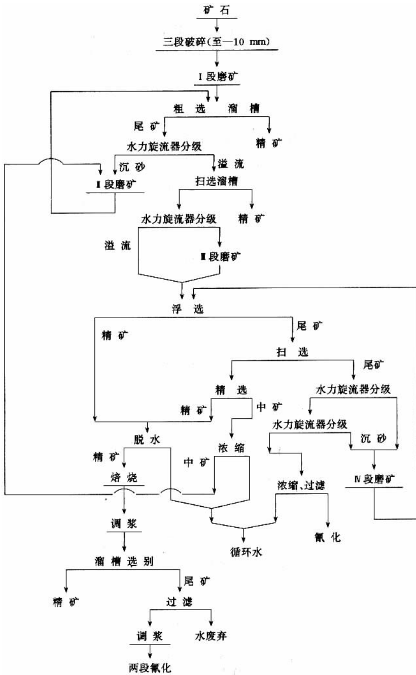
图 4-6-21 澳大利亚某选金厂处理难溶金-砷矿石的选冶工艺流程
