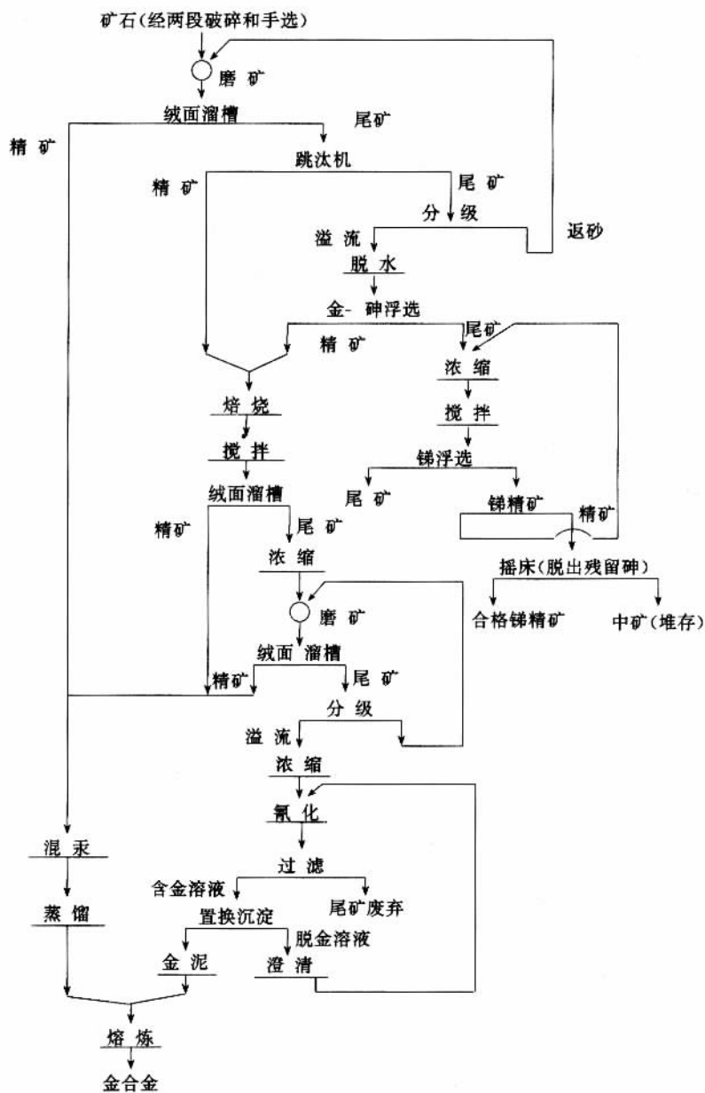
图 4-6-16 南非某选金厂金-锡矿石的生产工艺流程
