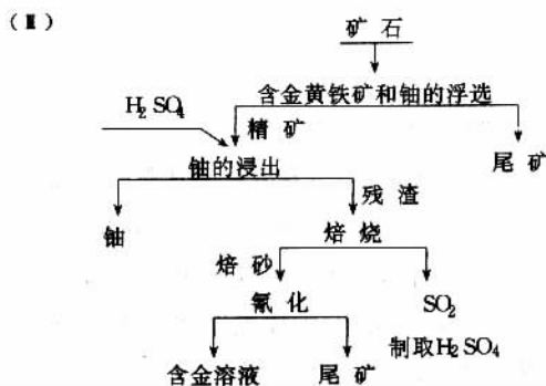
图 4-6-22 处理金铀矿石的原则流程
