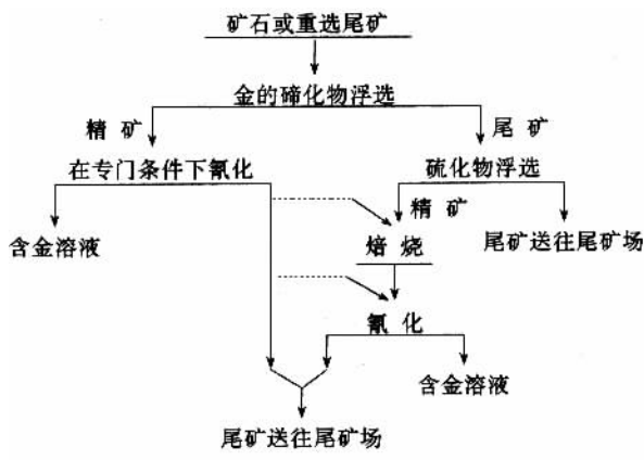
图 4-6-19 金-碲矿石优先浮选原则流程
