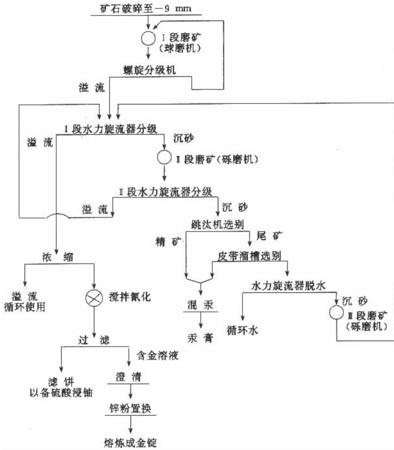
图 4-6-23 南非维斯捷尔恩 - 吉普 - 列维兹选冶厂生产工艺流程
