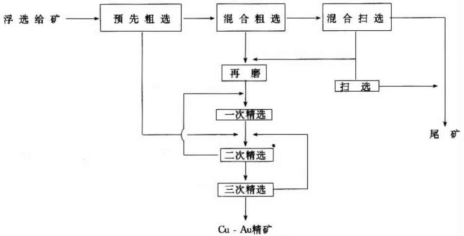
图 4-6-6 分步浮选流程
