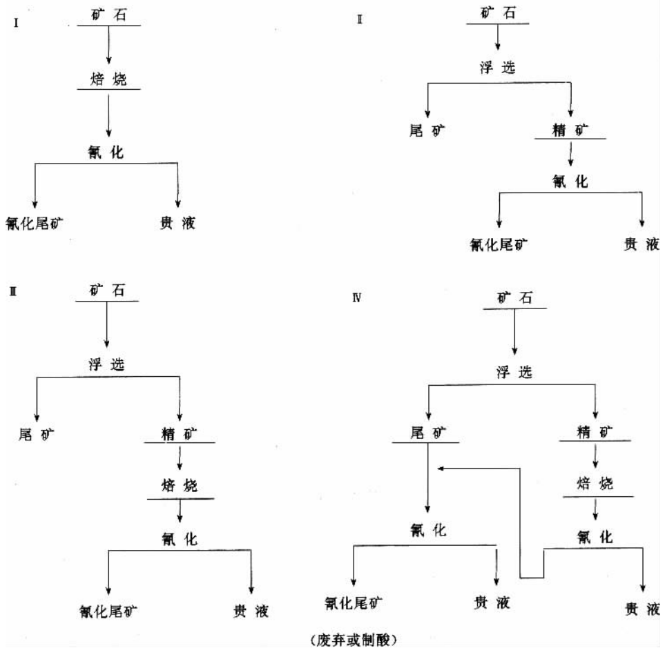
图 4-6-1 含金黄铁矿矿石选别原则流程
