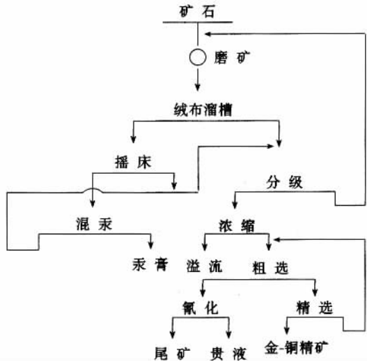
图 4-6-10 前苏联某金铜氧化矿石试验流程
