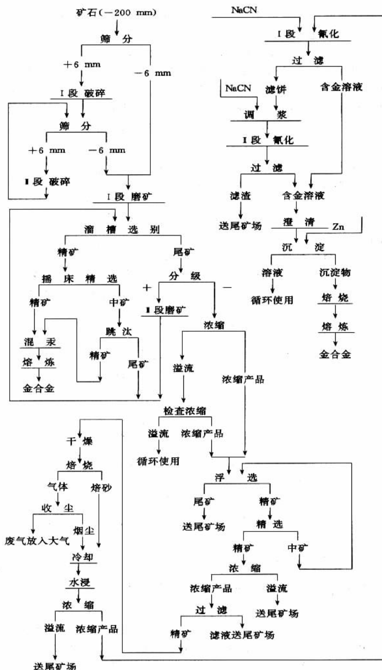
图 4-6-30 加纳阿利斯頓-高尔德-马英兹选金厂生产工艺流程
