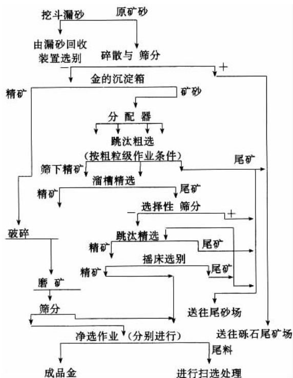
图 4-5-2 使用 MOII-2H 型跳汰机的选别流程
