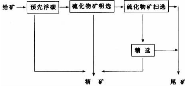
图 4-6-9 预先浮碳的分步浮选流程
