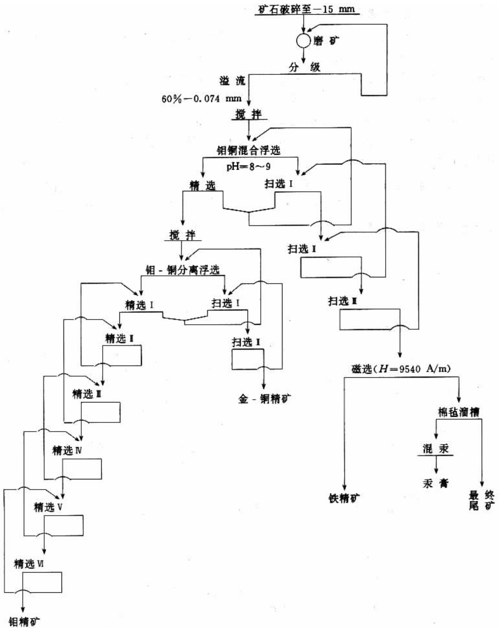
图 4-6-26 我国某选矿厂金-铜-钼-铁矿石选矿工艺流程
