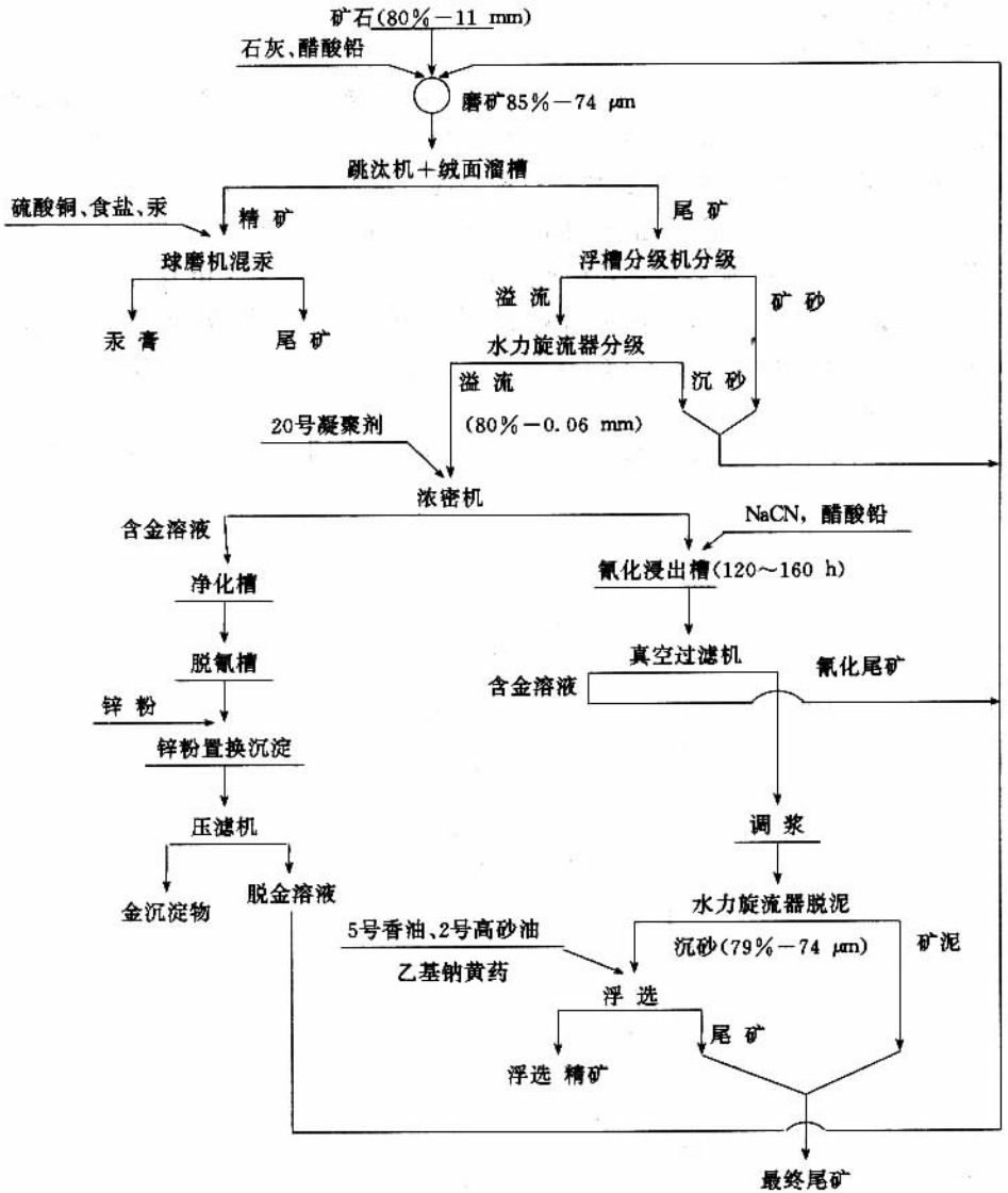
图 4-6-13 日本持越选矿厂矿石的生产工艺原则流程
