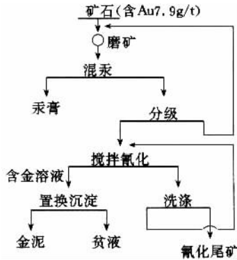
图4-5-20 我国某金矿混汞—氰化工艺试验流程
