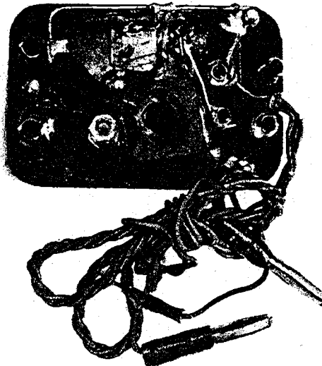
Radio-ontvangertjes, in lucifersdoosjes of andere kleine doosjes verborgen. Rechts boven kristalontvanger waarvan de draad als antenne dienst deed. De stekkers aan de draad van de onderste ontvanger werden aan de polen van een zaklantaarnbatterij vastgemaakt. Men kon met dergelijke toestellen de Londense uitzendingen volgen
