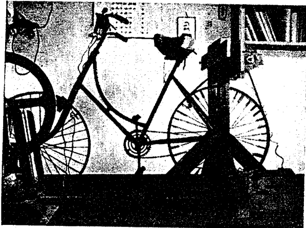
en fiets met spaken die met lood verzwaard zijn, gebruikt om een accu bij te laden
