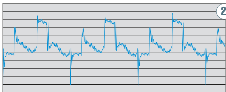
2 Форма сигнала, напряжения, выдаваемого инвертором на выходе с ИБП
