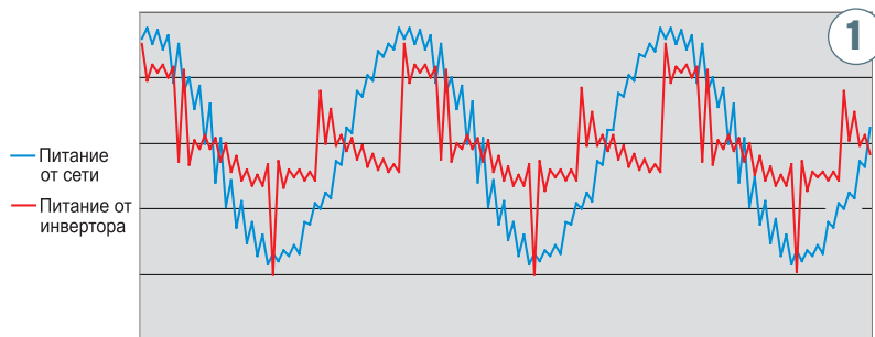
1 Сравнение формы напряжения, выдаваемого инвертором на выходе ИБП в автономном режиме с формой напряжения в сети
