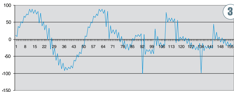
3 Переходная характеристика ИБП при переключении на инвертор
