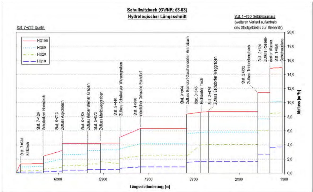
Abb. 17: Hydrologischer Gewässerlängsschnitt
