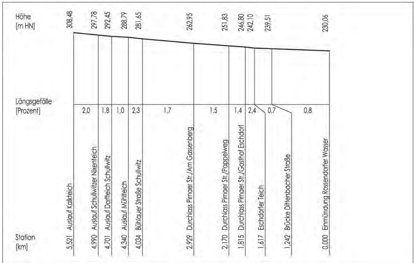
Abb. 7: Morphologischer Gewässerlängsschnitt
