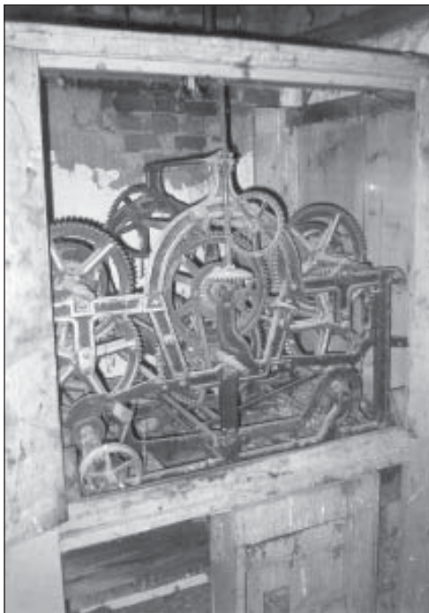
A régi mechanikus óramű
