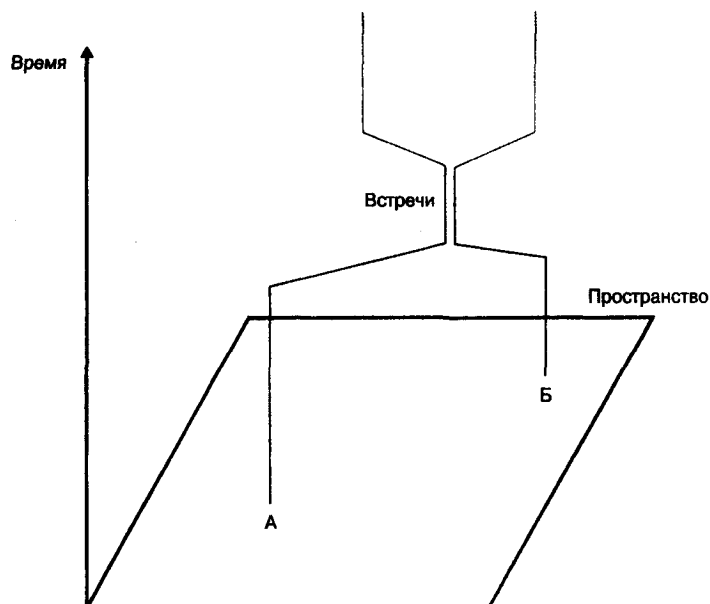
Рис. 2. Траектории индивидуального движения во времени и пространстве: А и Б движутся навстречу друг другу, проводят некоторое время вместе и затем расходятся
